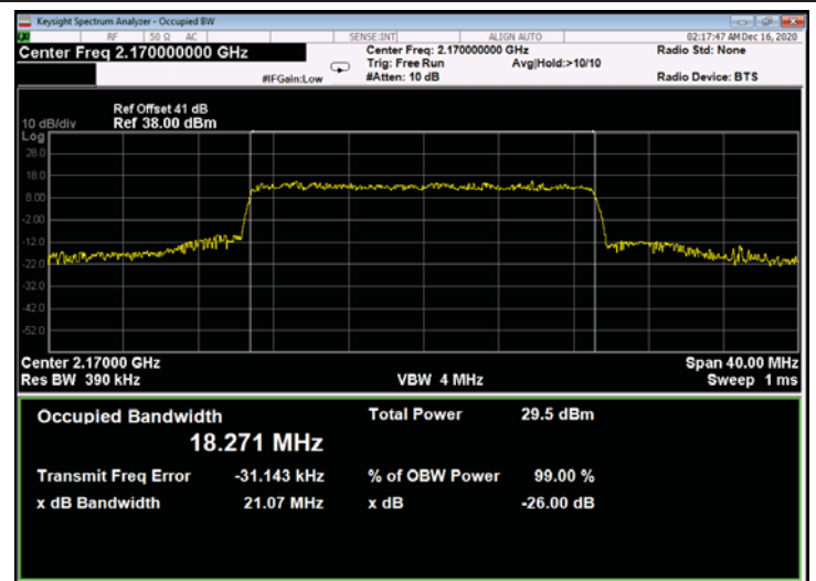
Figure 766: QPSK 20MHz B.W.; 2170.0MHz, 30kHz - Output
