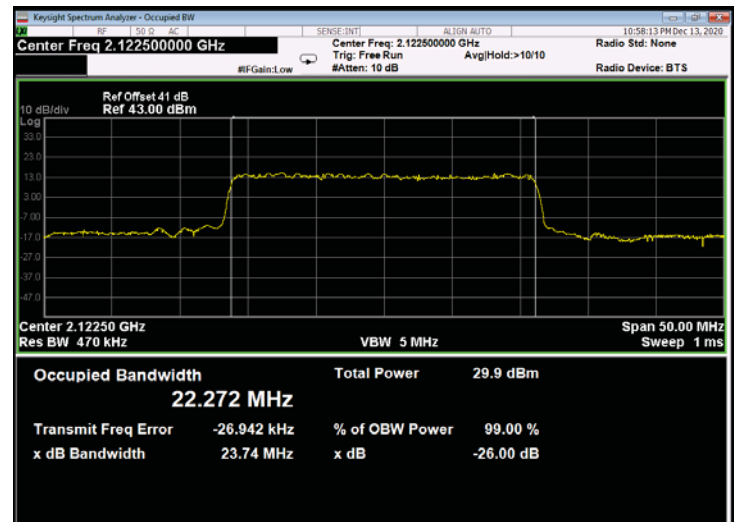
Figure 770: QPSK 25MHz B.W.; 2122.5MHz, 60kHz - Output
