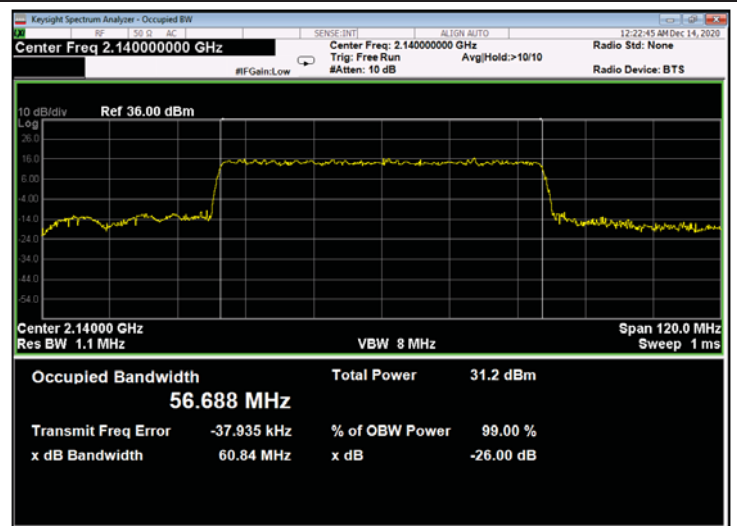
Figure 796: QPSK 60MHz B.W.; 2140.0MHz, 60kHz - Output
