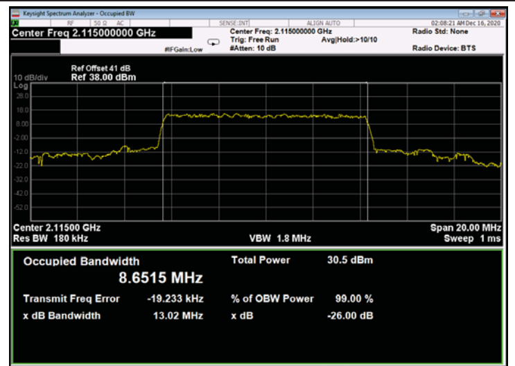
Figure 742: QPSK 10MHz B.W.; 2115.0MHz, 30kHz - Output
