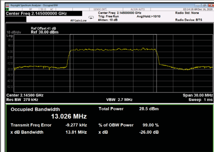
Figure 755: QPSK 15MHz B.W.; 2145.0MHz, 60kHz - Output
