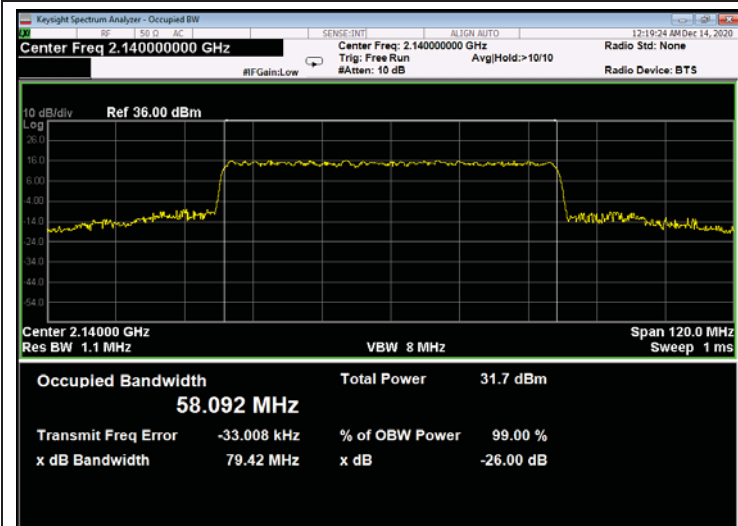
Figure 795: QPSK 60MHz B.W.;2140.0MHz, 30kHz - Output
