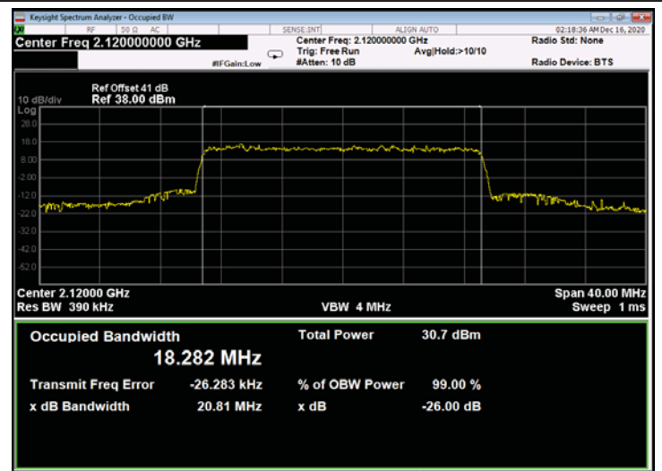
Figure 760: QPSK 20MHz B.W.; 2120.0MHz, 30kHz - Output
