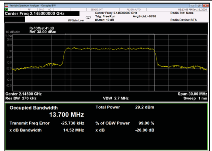
Figure 754: QPSK 15MHz B.W.; 2145.0MHz, 30kHz - Output
