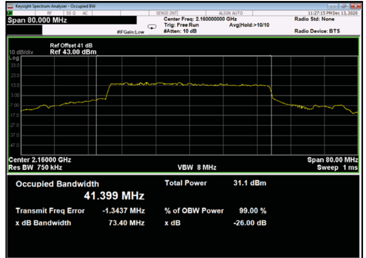
Figure 784: QPSK 40MHz B.W.; 2160.0MHz, 30kHz - Output
