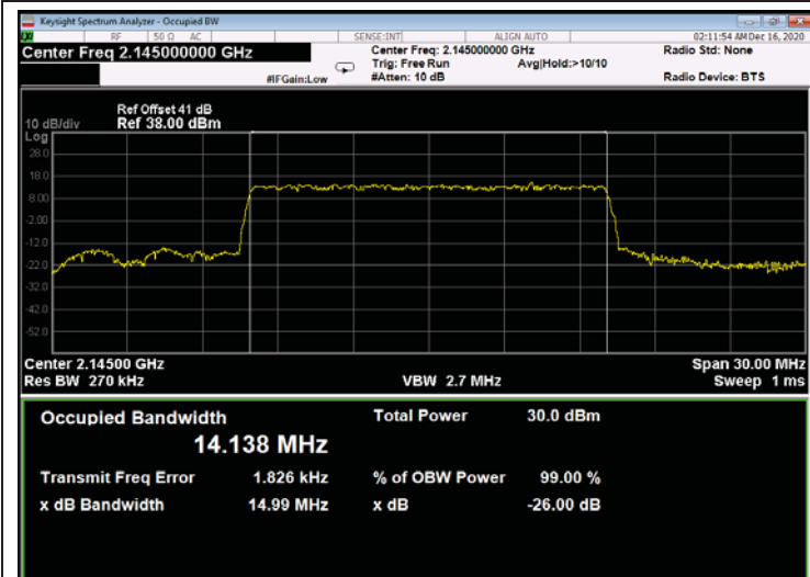
Figure 753: QPSK 15MHz B.W.; 2145.0MHz, 15kHz - Output
