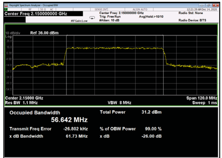
Figure 800: QPSK 60MHz B.W.; 2150.0MHz, 60kHz - Output
