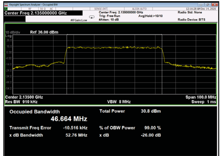
Figure 788: QPSK 50MHz B.W.; 2135.0MHz, 60kHz - Output
