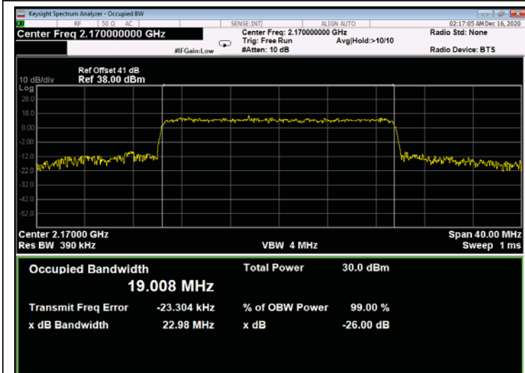
Figure 765: QPSK 20MHz B.W.; 2170.0MHz, 15kHz - Output
