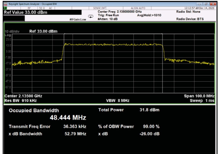
Figure 786: QPSK 50MHz B.W.; 2135.0MHz, 15kHz - Output
