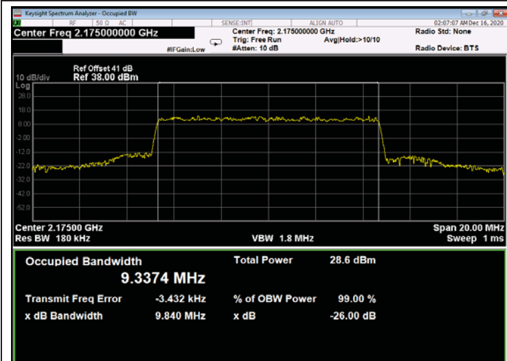
Figure 747: QPSK 10MHz B.W.; 2175.0MHz, 15kHz - Output
