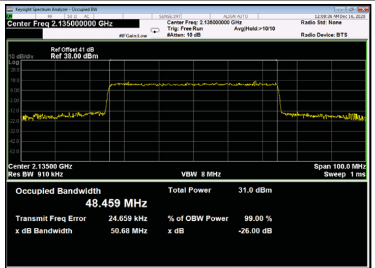
Figure 654: 64QAM 50MHz B.W.; 2135.0MHz, 15kHz - Output
