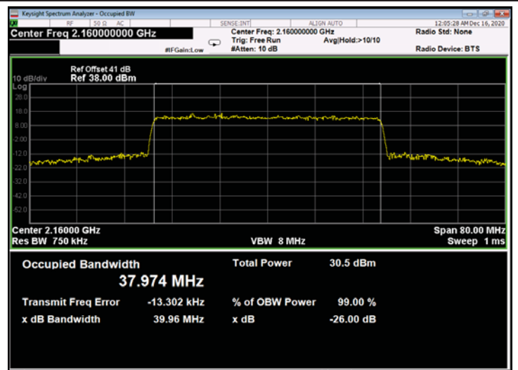
Figure 652: 64QAM 40MHz B.W.; 2160.0MHz, 30kHz - Output
