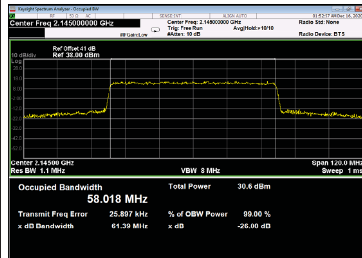
Figure 731: 256QAM 60MHz B.W.; 2145.0MHz, 30kHz - Output
