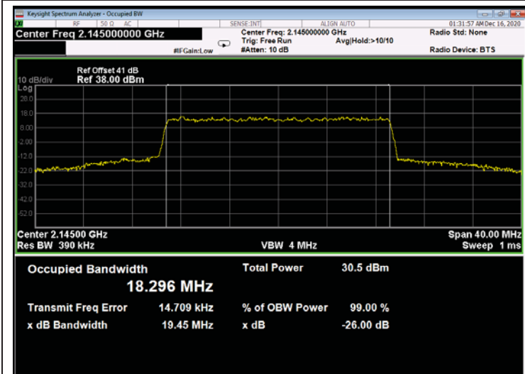
Figure 697: 256QAM 20MHz B.W.; 2145.0MHz, 30kHz - Output
