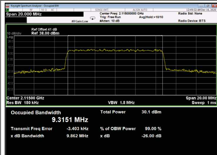
Figure 675: 256QAM 10MHz B.W.; 2115.00MHz, 15kHz - Output
