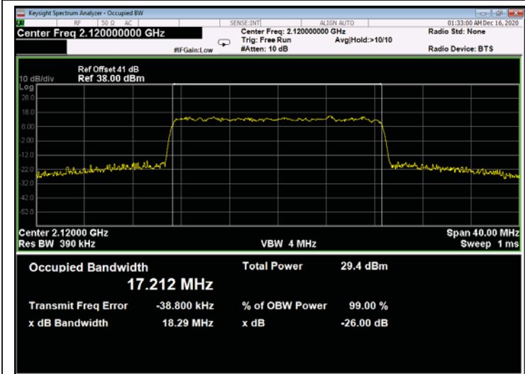
Figure 695: 256QAM 20MHz B.W.; 2120.0MHz, 60kHz - Output
