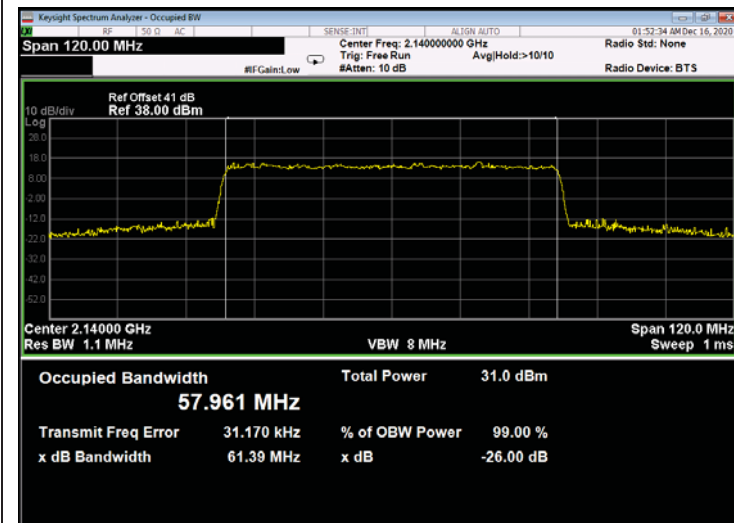
Figure 729: 256QAM 60MHz B.W.; 2140.0MHz, 30kHz - Output
