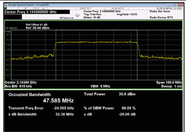
Figure 724: 256QAM 50MHz B.W.; 2145.0MHz, 30kHz - Output
