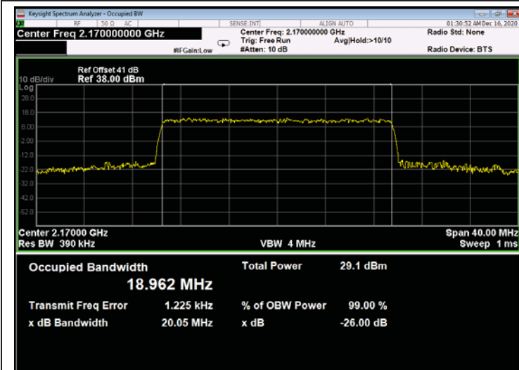
Figure 699: 256QAM 20MHz B.W.; 2170.0MHz, 15kHz - Output
