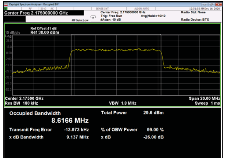
Figure 682: 256QAM 10MHz B.W.; 2175.0MHz, 30kHz - Output
