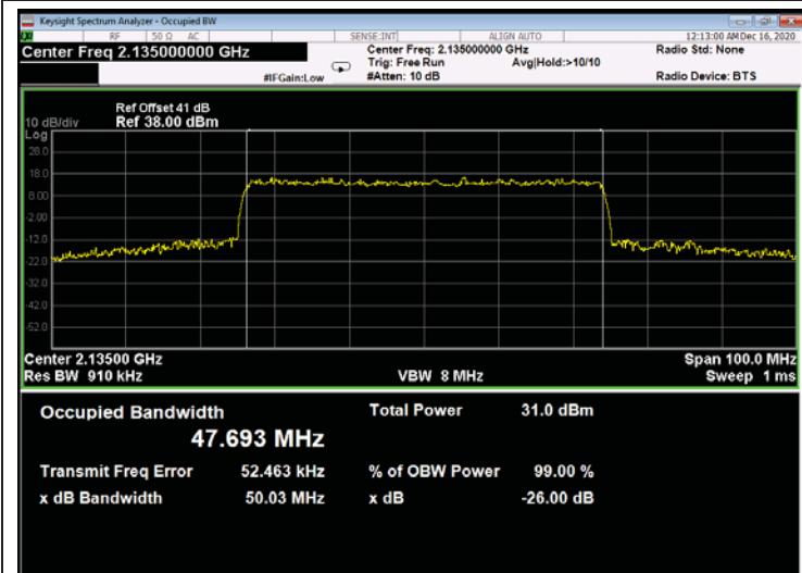
Figure 655: 64QAM 50MHz B.W.; 2135.0MHz, 30kHz - Output
