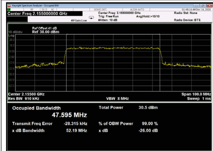
Figure 727: 256QAM 50MHz B.W.; 2155.0MHz, 30kHz - Output
