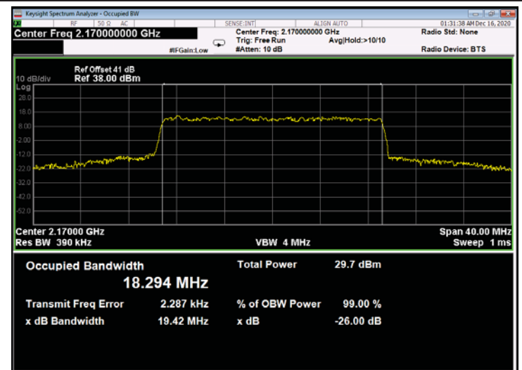
Figure 700: 256QAM 20MHz B.W.; 2170.0MHz, 30kHz - Output
