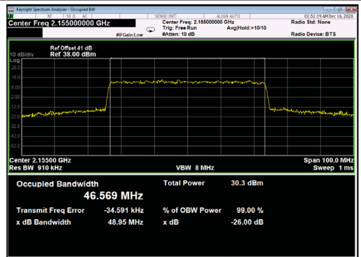
Figure 728: 256QAM 50MHz B.W.; 2155.0MHz, 60kHz - Output
