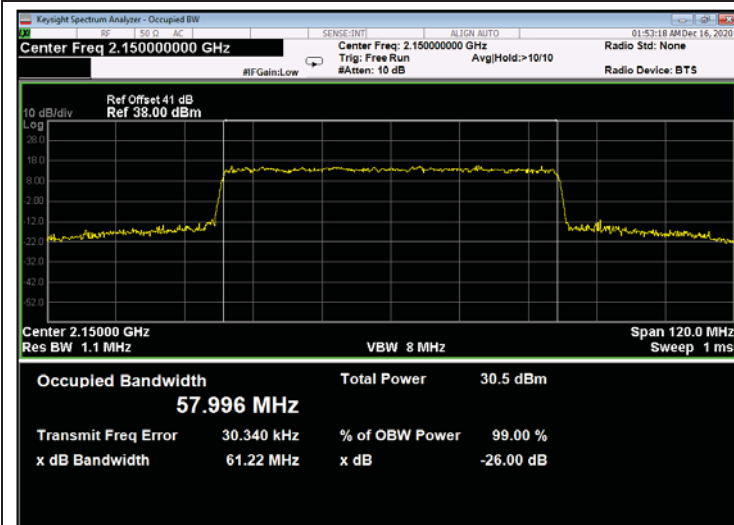
Figure 733: 256QAM 60MHz B.W.; 2150.0MHz, 30kHz - Output
