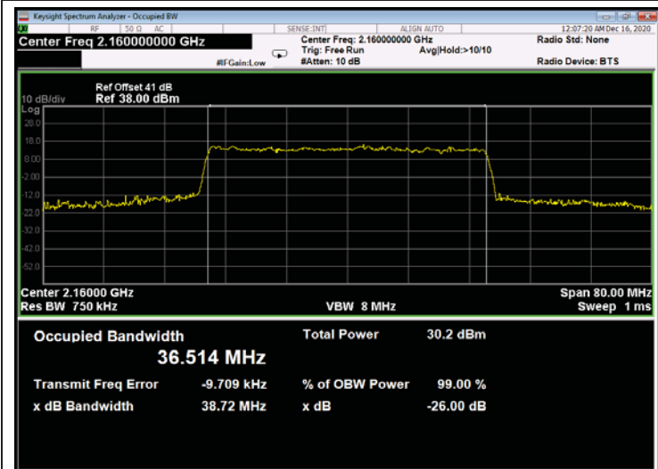
Figure 653: 64QAM 40MHz B.W.; 2160.0MHz, 60kHz - Output
