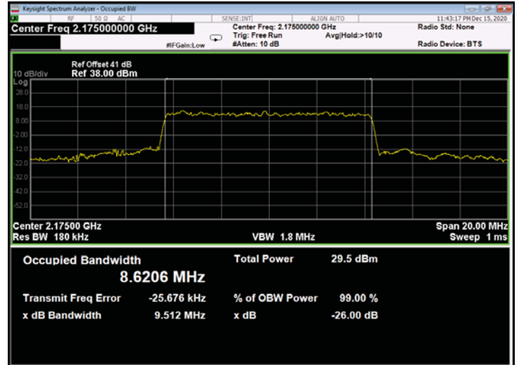
Figure 616: 64QAM 10MHz B.W.; 2175.0MHz, 30kHz - Output
