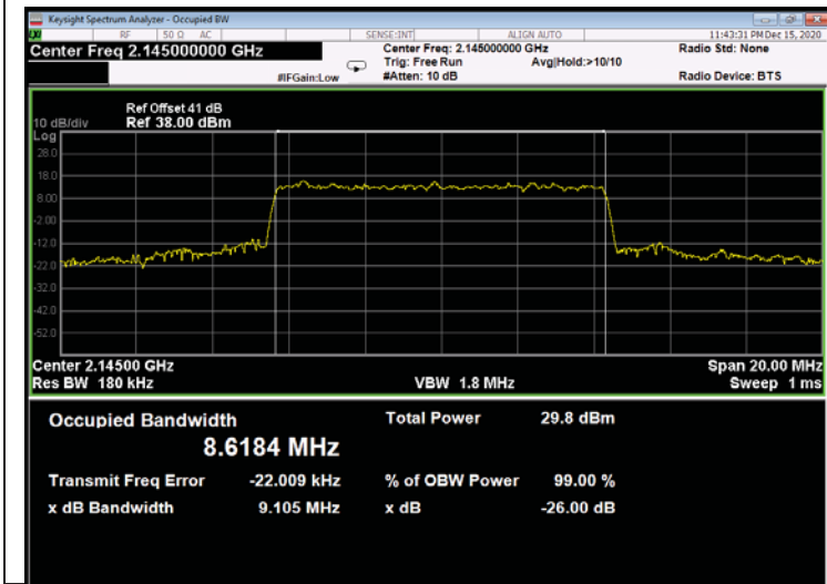
Figure 613: 64QAM 10MHz B.W.; 2145.00MHz, 30kHz - Output
