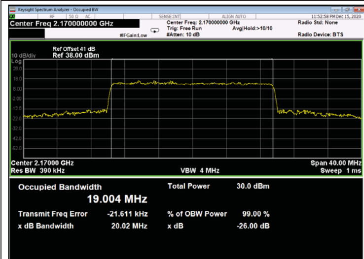
Figure 633: 64QAM 20MHz B.W.; 2170.0MHz, 15kHz - Output
