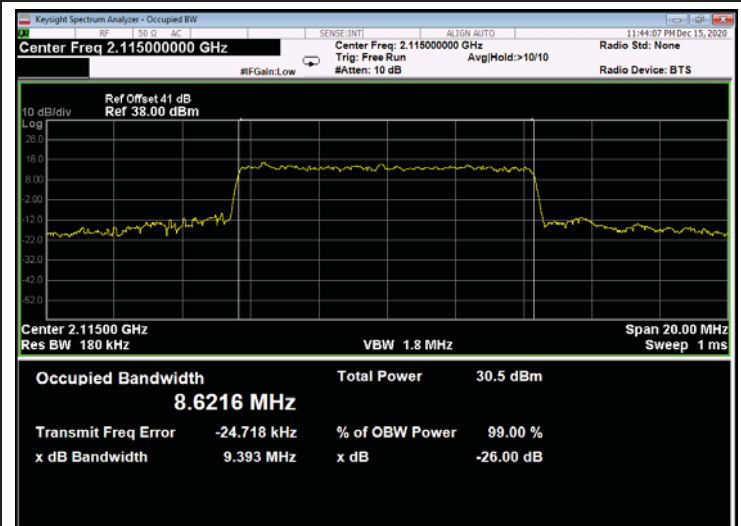
Figure 610: 64QAM 10MHz B.W.; 2115.00MHz, 30kHz - Output
