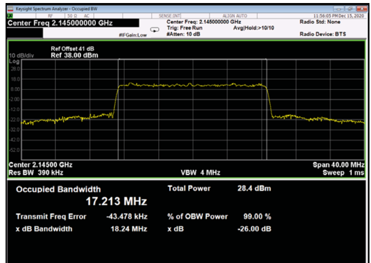
Figure 632: 64QAM 20MHz B.W.; 2145.0MHz, 60kHz - Output
