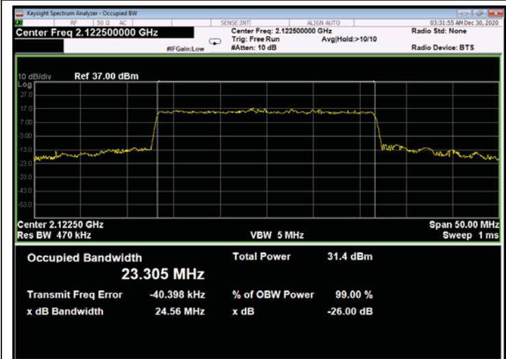
Figure 637: 64QAM 25MHz B.W.; 2122.5.0MHz, 30kHz - Output
