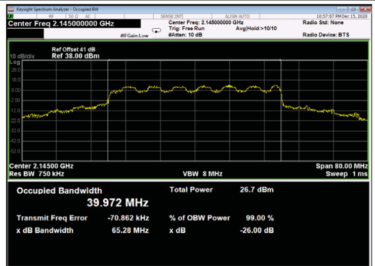
Figure 582: 16QAM 40MHz B.W.; 2145.0MHz, 15kHz - Output
