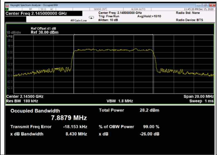
Figure 614: 64QAM 10MHz B.W.; 2145.00MHz, 60kHz - Output
