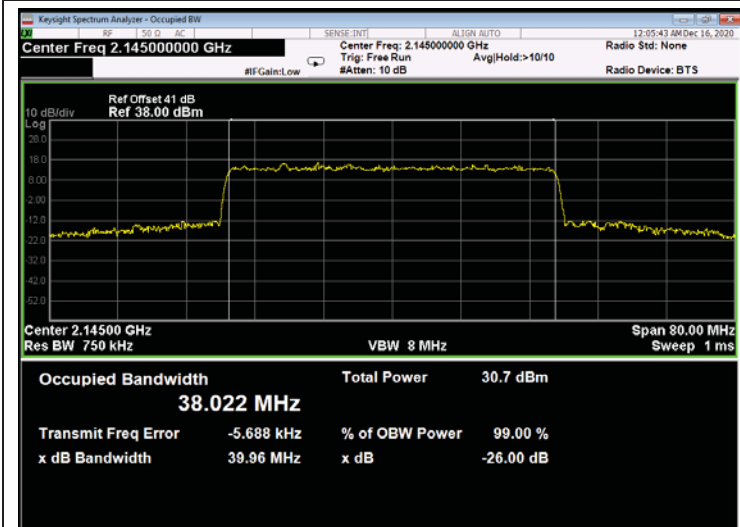
Figure 649: 64QAM 40MHz B.W.; 2145.0MHz, 30kHz - Output
