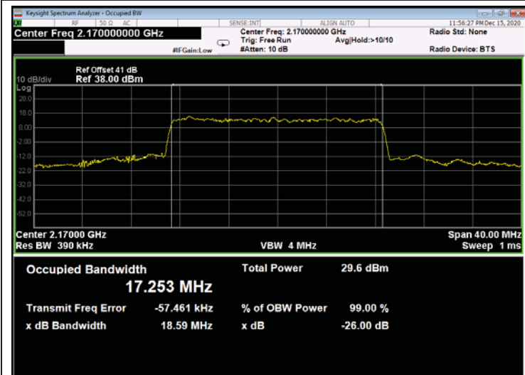
Figure 635: 64QAM 20MHz B.W.; 2170.0MHz, 60kHz - Output
