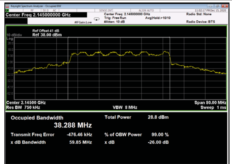
Figure 584: 16QAM 40MHz B.W.; 2145.0MHz, 60kHz - Output
