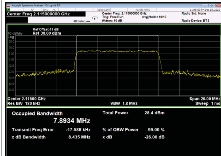
Figure 611: 64QAM 10MHz B.W.; 2115.00MHz, 60kHz - Output
