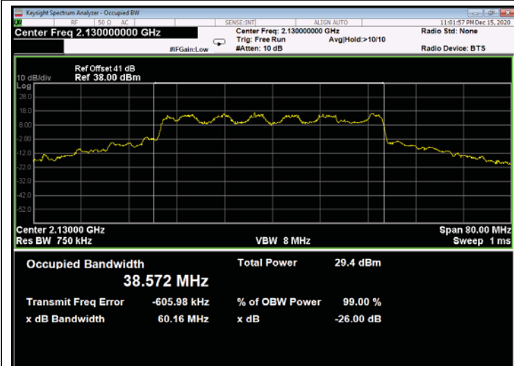
Figure 581: 16QAM 40MHz B.W.; 2130.0MHz, 60kHz - Output
