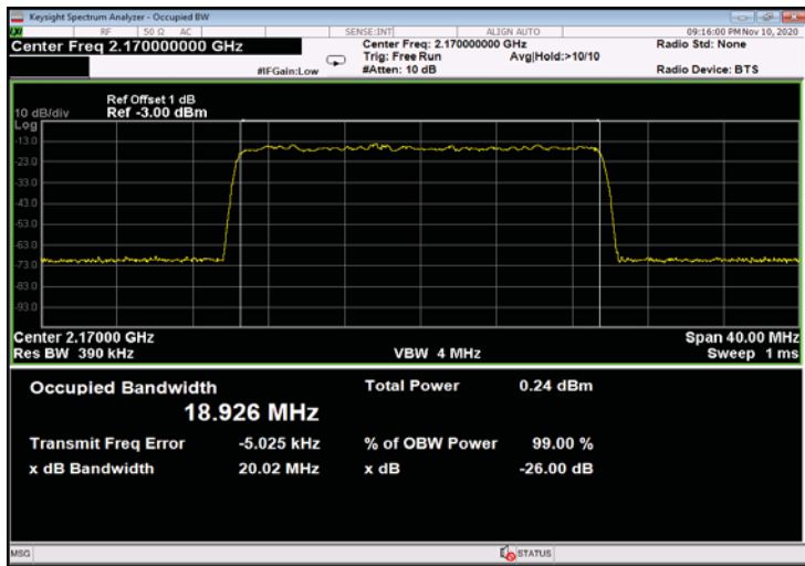
Figure 501: QPSK 20MHz B.W.; 2170.0MHz, 15kHz - Input
