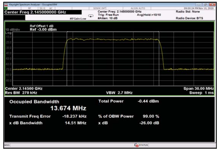
Figure 490: QPSK 15MHz B.W.; 2145.0MHz, 30kHz - Input
