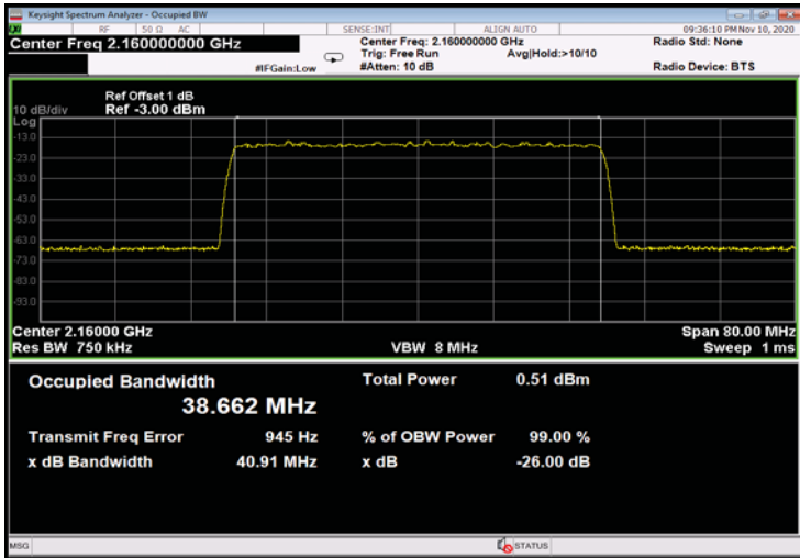
Figure 519: QPSK 40MHz B.W.; 2160.0MHz, 15kHz - Input
