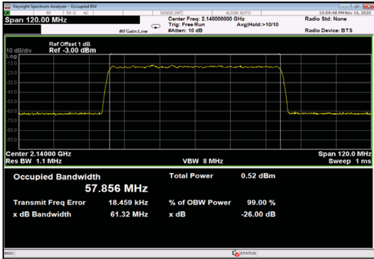
Figure 531: QPSK 60MHz B.W.; 2140.0MHz, 30kHz - Input
