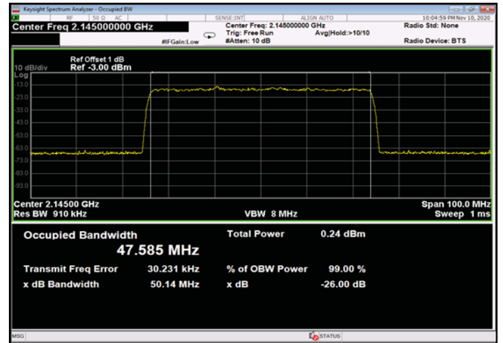
Figure 526: QPSK 50MHz B.W.; 2145.0MHz, 30kHz - Input
