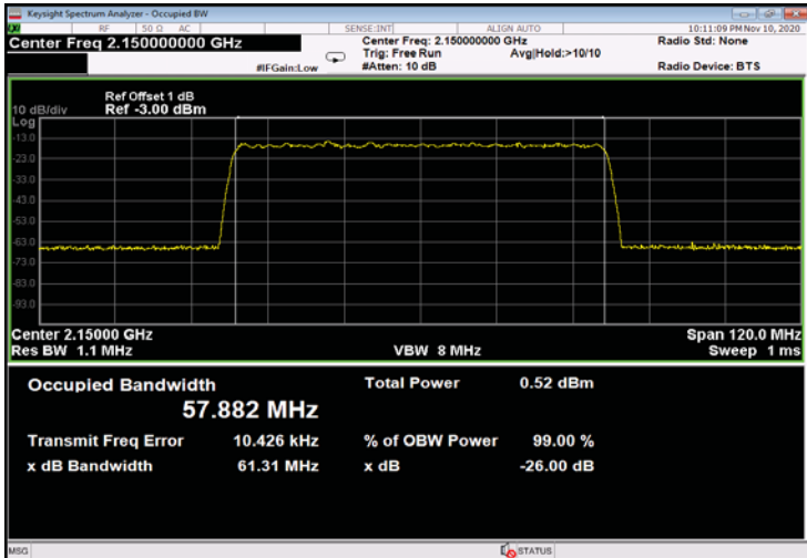
Figure 535: QPSK 60MHz B.W.; 2150.0MHz, 30kHz - Input
