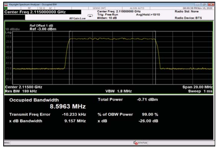
Figure 478: QPSK 10MHz B.W.; 2115.0MHz, 30kHz - Input
