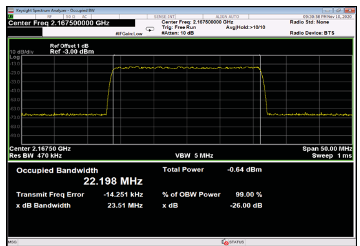
Figure 512: QPSK 25MHz B.W.; 2167.5MHz, 60kHz - Input
