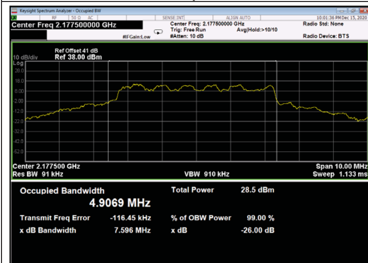
Figure 541: 16QAM 5MHz B.W.; 2177.5MHz, 15kHz - Output
