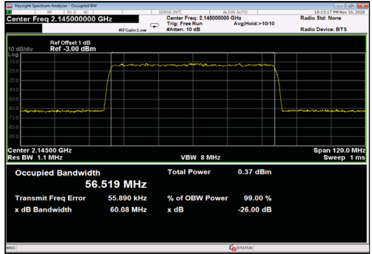
Figure 534: QPSK 60MHz B.W.; 2145.0MHz, 60kHz - Input
