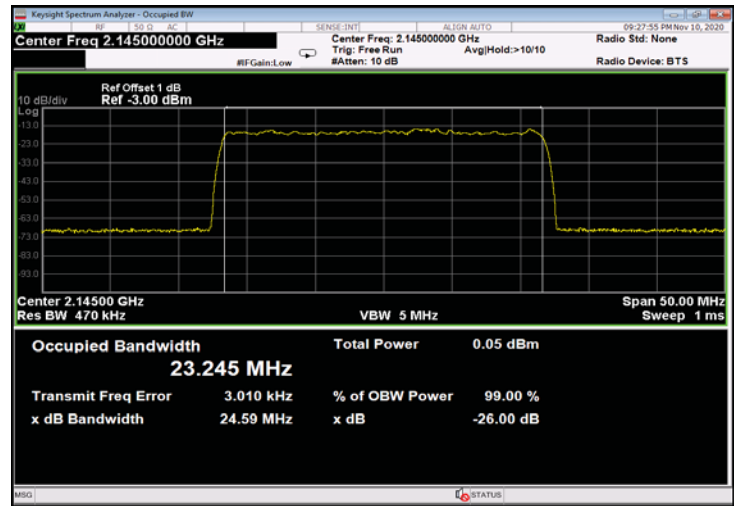
Figure 508: QPSK 25MHz B.W.; 2145.0MHz, 30kHz - Input
