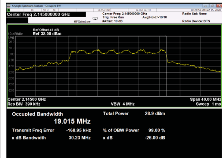
Figure 565: 16QAM 20MHz B.W.; 2145.0MHz, 30kHz - Output
