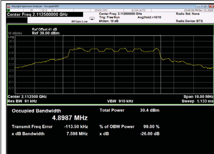
Figure 537: 16QAM 5MHz B.W.; 2112.5MHz, 15kHz - Output
