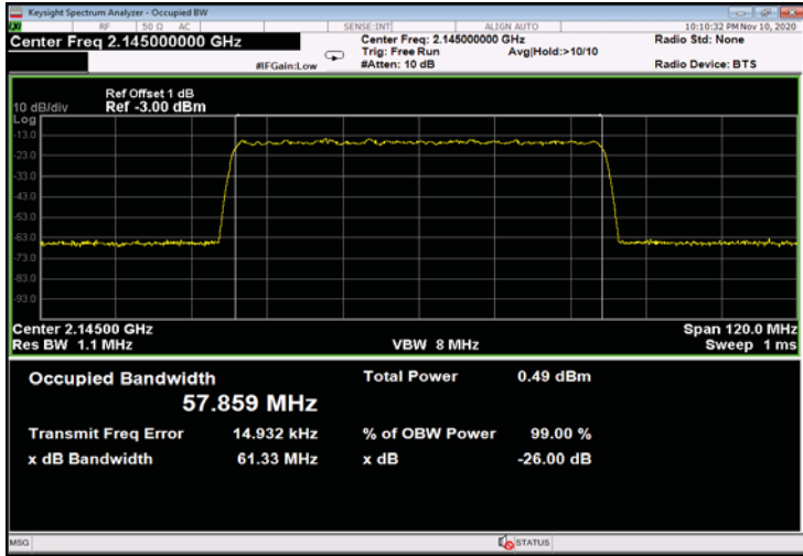
Figure 533: QPSK 60MHz B.W.; 2145.0MHz, 30kHz - Input
