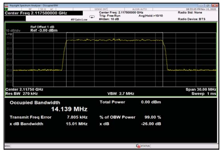
Figure 486: QPSK 15MHz B.W.; 2117.5MHz, 15kHz - Input
