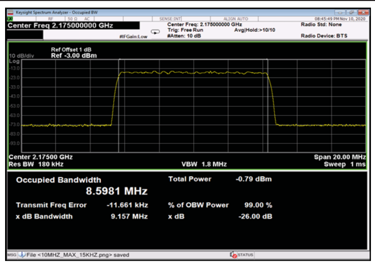
Figure 484: QPSK 10MHz B.W.; 2175.0MHz, 30kHz - Input
