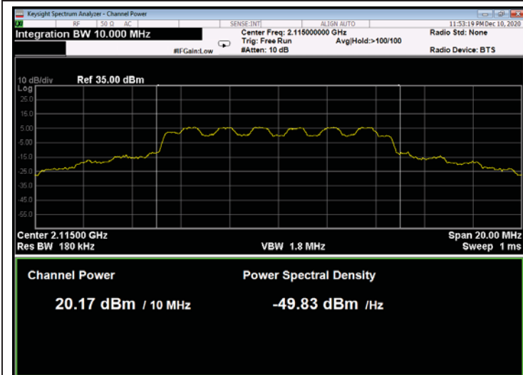
Figure 15: 16QAM 10MHz B.W.; 2115.0MHz, 15kHz
