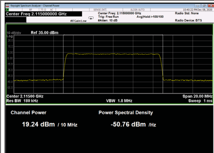
Figure 81: 64QAM 10MHz B.W.;2115.0MHz, 15kHz
