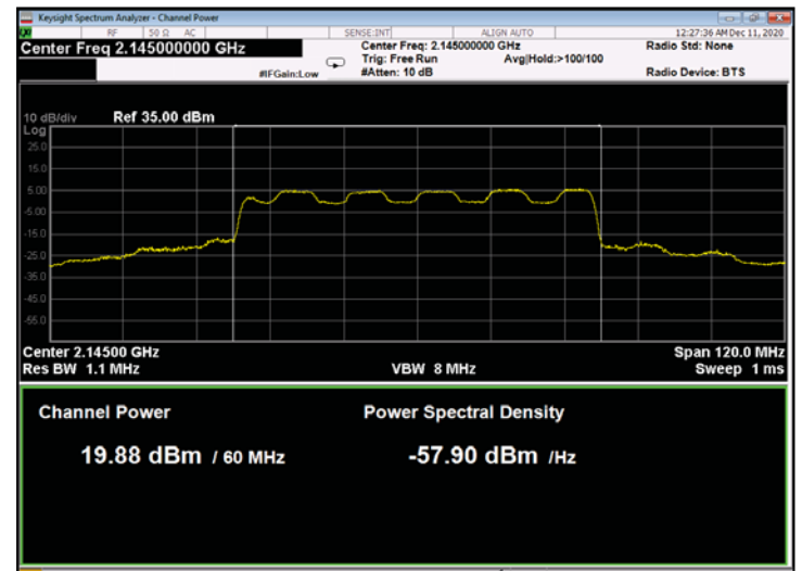
Figure 72: 16QAM 60MHz B.W.; 2145.0MHz, 60kHz
