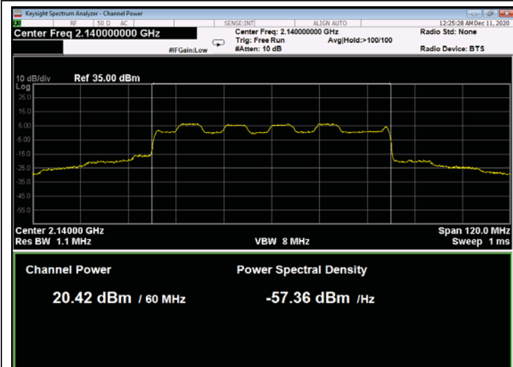
Figure 69: 16QAM 60MHz B.W.; 2140.0MHz, 30kHz
