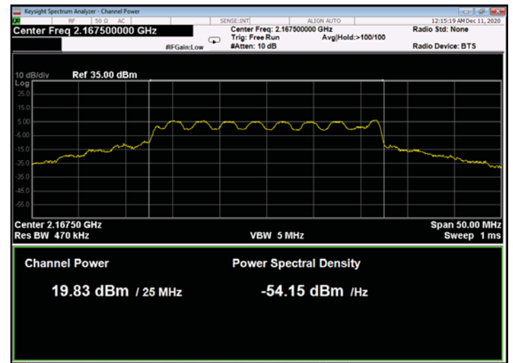
Figure 48: 16QAM 25MHz B.W.; 2167.5MHz, 15kHz
