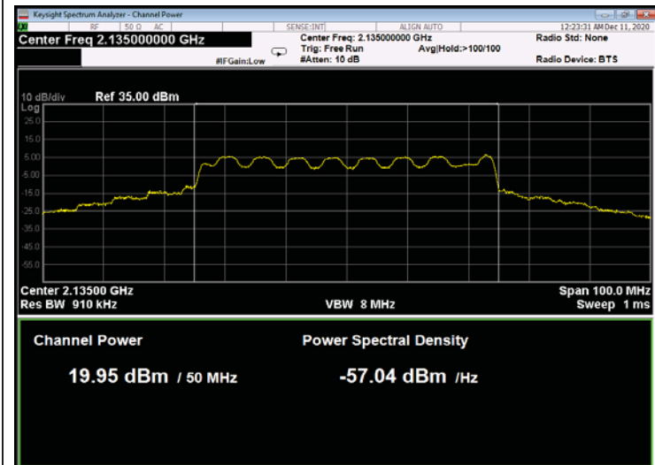
Figure 61: 16QAM 50MHz B.W.; 2135.0MHz, 30kHz
