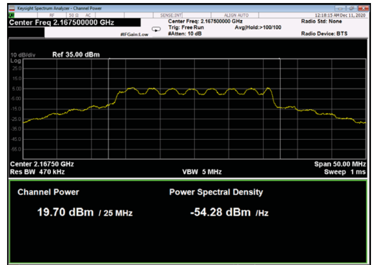
Figure 50: 16QAM 25MHz B.W.; 2167.5MHz, 60kHz
