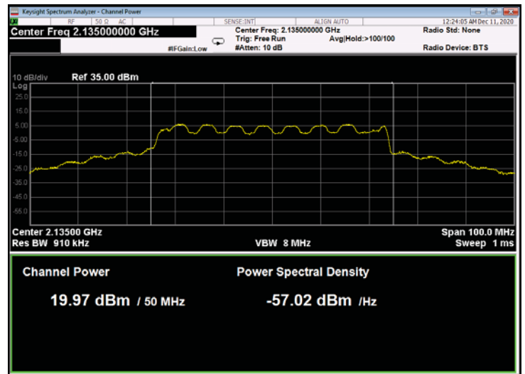
Figure 62: 16QAM 50MHz B.W.; 2135.0MHz, 60kHz
