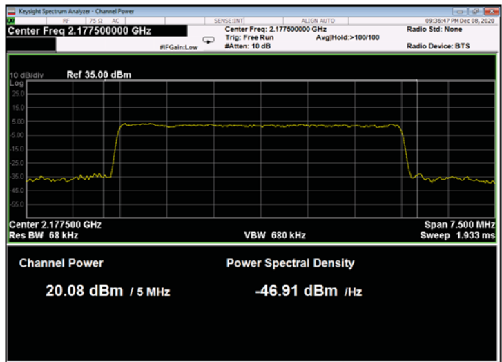
Figure 79: 64QAM 5MHz B.W.; 2177.5MHz, 15kHz
