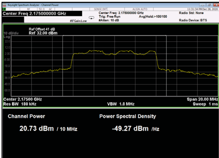
Figure 23: 16QAM 10MHz B.W.; 2175.0MHz, 60kHz
