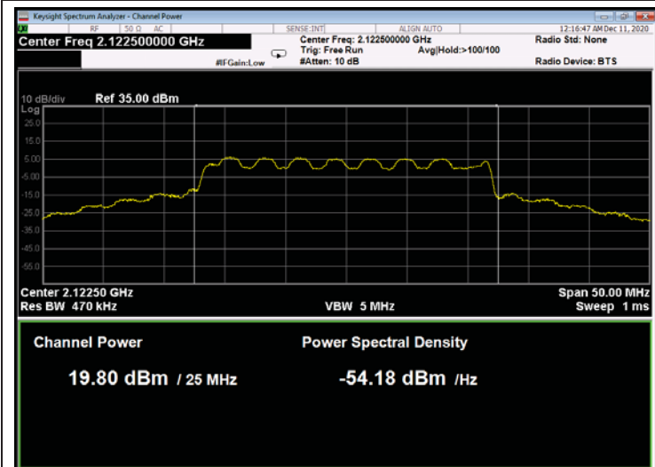
Figure 43: 16QAM 25MHz B.W.; 2122.5MHz, 30kHz
