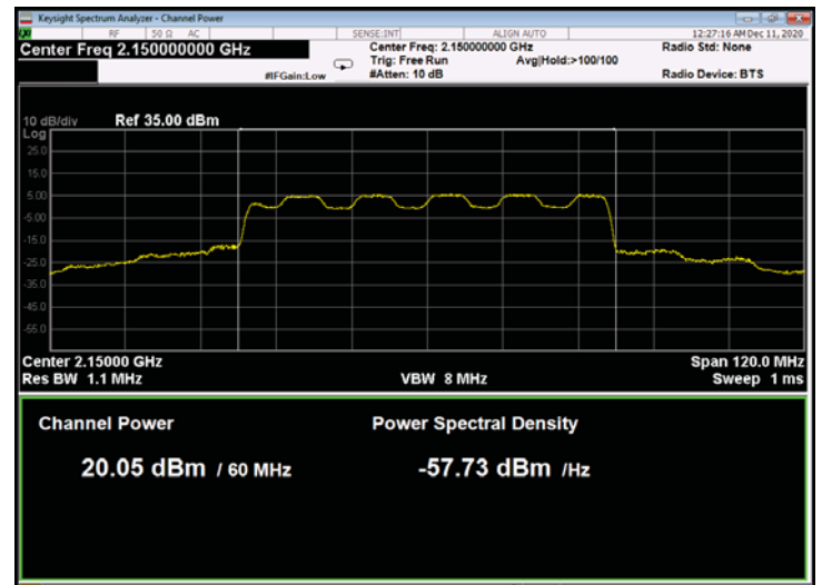
Figure 74: 16QAM 60MHz B.W.; 2150.0MHz, 60kHz
