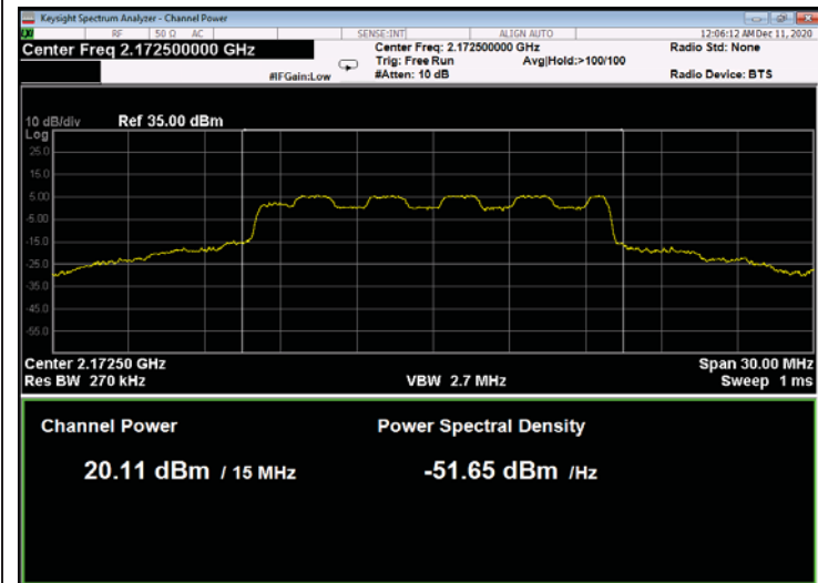
Figure 31: 16QAM 15MHz B.W.; 2172.5MHz, 30kHz
