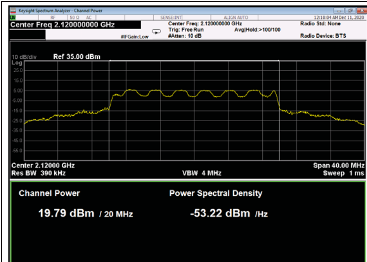
Figure 33: 16QAM 20MHz B.W.; 2120.0MHz, 15kHz
