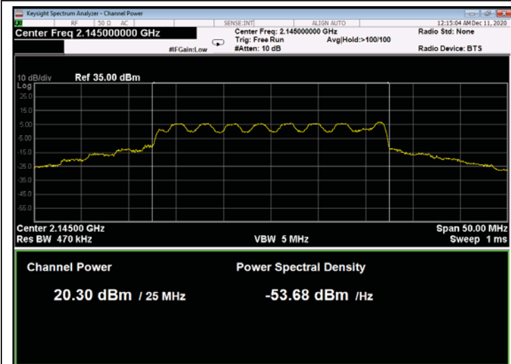
Figure 45: 16QAM 25MHz B.W.; 2145.0MHz, 15kHz
