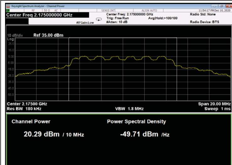
Figure 21: 16QAM 10MHz B.W.; 2175.0MHz, 15kHz
