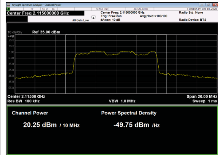
Figure 17: 16QAM 10MHz B.W.; 2115.0MHz, 60kHz
