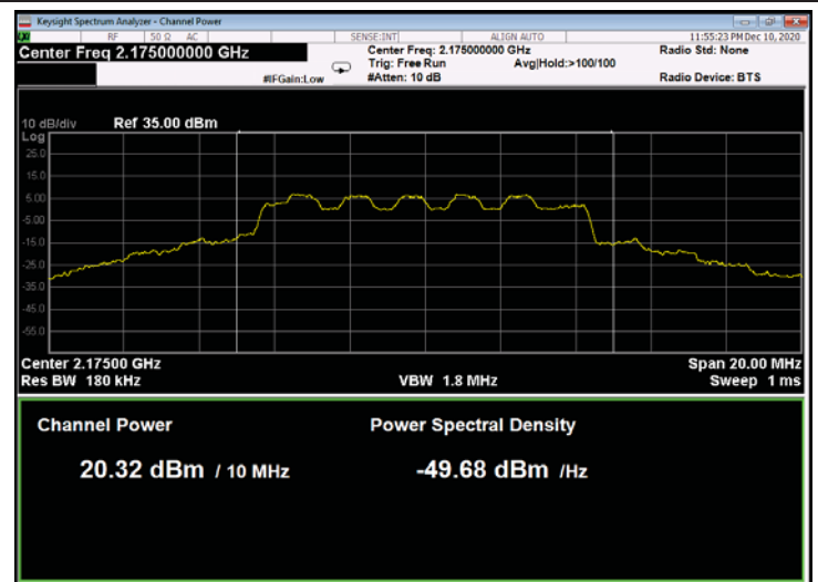
Figure 22: 16QAM 10MHz B.W.; 2175.0MHz, 30kHz
