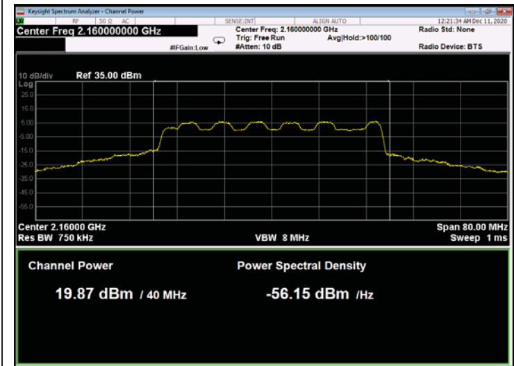
Figure 59: 16QAM 40MHz B.W.; 2160.0MHz, 60kHz
