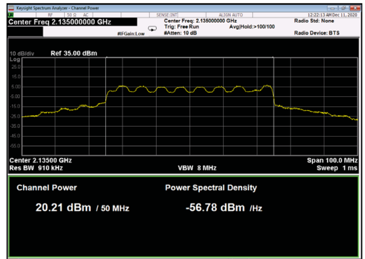
Figure 60: 16QAM 50MHz B.W.; 2135.0MHz, 15kHz
