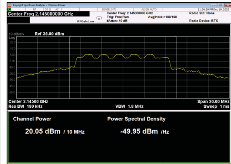
Figure 19: 16QAM 10MHz B.W.; 2145.0MHz, 30kHz
