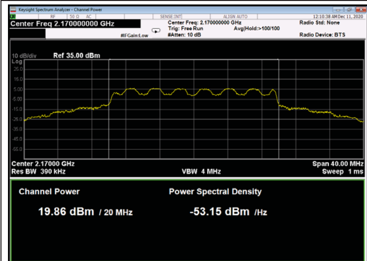
Figure 39: 16QAM 20MHz B.W.; 2170.0MHz, 15kHz
