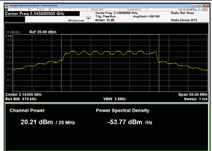
Figure 46: 16QAM 25MHz B.W.; 2145.0MHz, 30kHz
