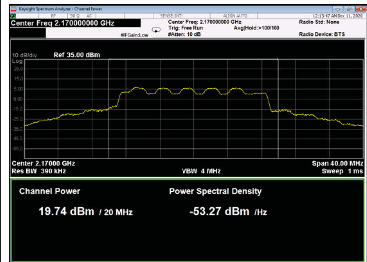
Figure 41: 16QAM 20MHz B.W.; 2170.0MHz, 60kHz
