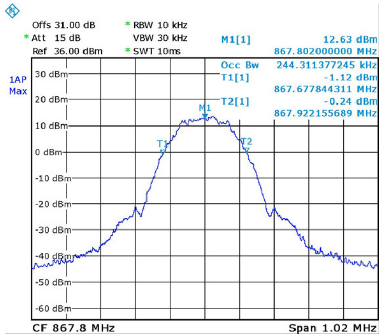
Figure 80. — 867.8MHz GSM Input
