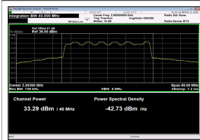
Figure 44: 16QAM 40MHz B.W.; 2593.0MHz, 15kHz
