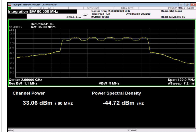
Figure 54: 16QAM 60MHz B.W.; 2660.0MHz, 30kHz
