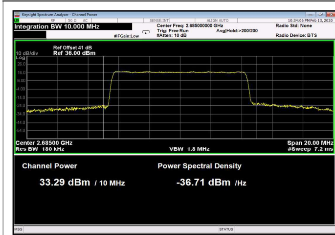
Figure 68: 64QAM 10MHz B.W.; 2685.0MHz, 15kHz
