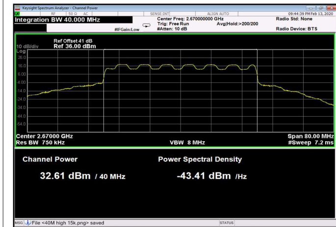
Figure 48: 16QAM 40MHz B.W.; 2670.0MHz, 30kHz
