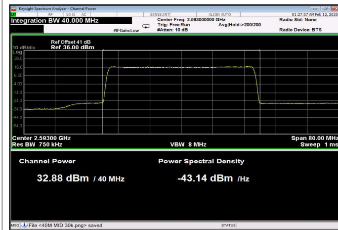
Figure 94: 64QAM 40MHz B.W.; 2593.0MHz, 60kHz
