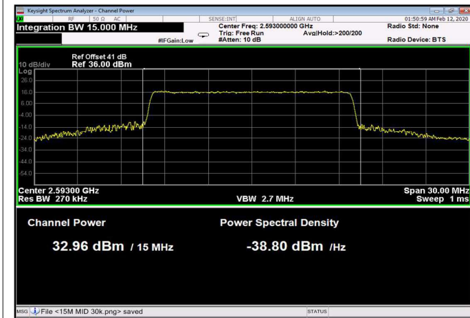
Figure 76: 64QAM 15MHz B.W.; 2593.0MHz, 60kHz
