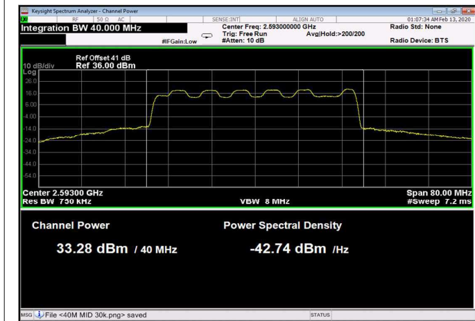
Figure 46: 16QAM 40MHz B.W.; 2593.0MHz, 60kHz
