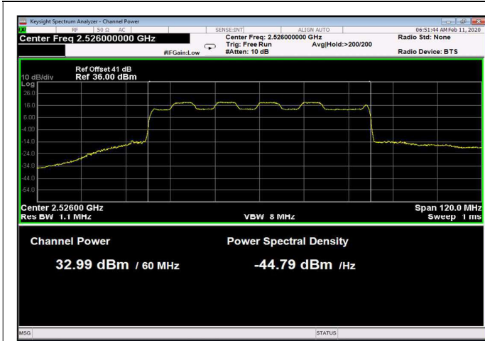
Figure 50: 16QAM 60MHz B.W.; 2526.0MHz, 30kHz
