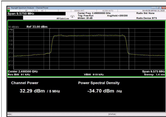
Figure 56: 64QAM 5MHz B.W.; 2498.5MHz, 15kHz
