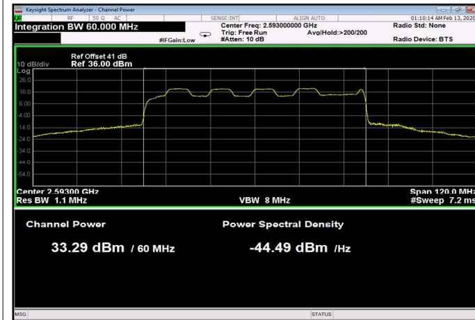
Figure 52: 16QAM 60MHz B.W.; 2593.0MHz, 30kHz
