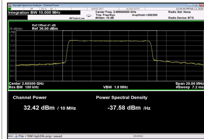
Figure 70: 64QAM 10MHz B.W.; 2685.0MHz, 60kHz
