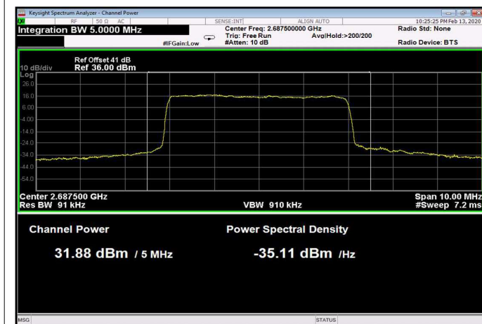
Figure 60: 64QAM 5MHz B.W.; 2687.5MHz, 15kHz
