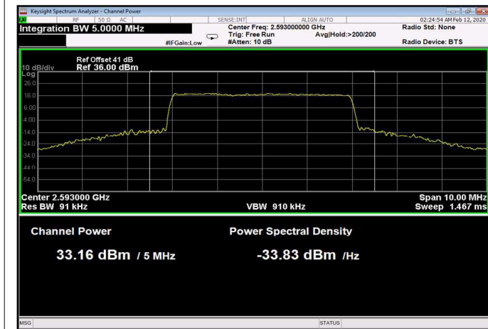
Figure 58: 16QAM 5MHz B.W.; 2593.0MHz, 15kHz
