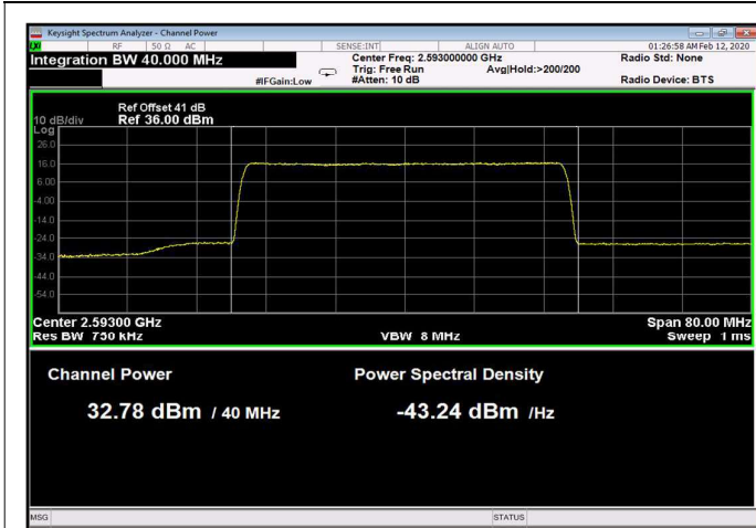
Figure 92: 64QAM 40MHz B.W.; 2593.0MHz, 15kHz
