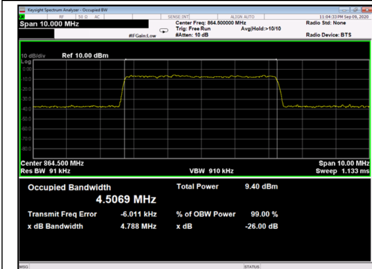
Figure 302: QPSK 5MHz B.W.; 864.5MHz, 15kHz - Input
