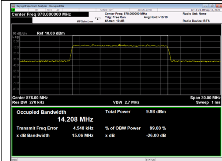
Figure 320: QPSK 15MHz B.W.; 878.0MHz, 15kHz - Input
