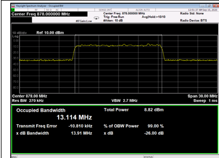
Figure 322: QPSK 15MHz B.W.; 878.0MHz, 60kHz - Input
