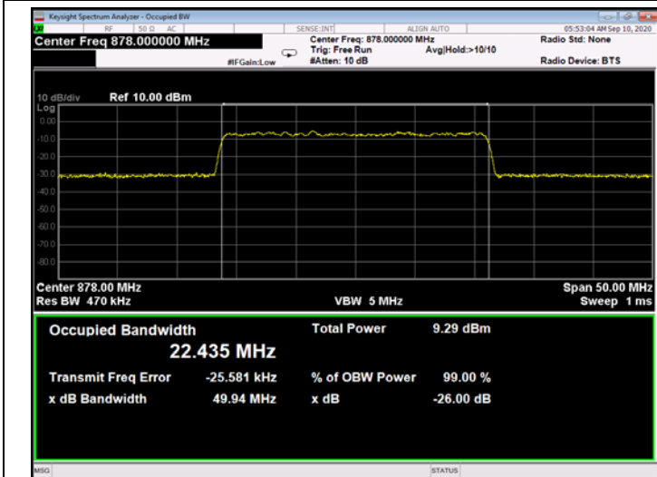
Figure 298: 256QAM 25MHz B.W.; 878.0MHz, 60kHz - Input
