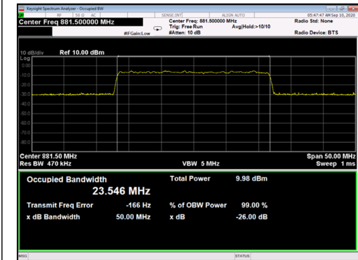
Figure 300: 256QAM 25MHz B.W.; 881.5MHz, 30kHz - Input
