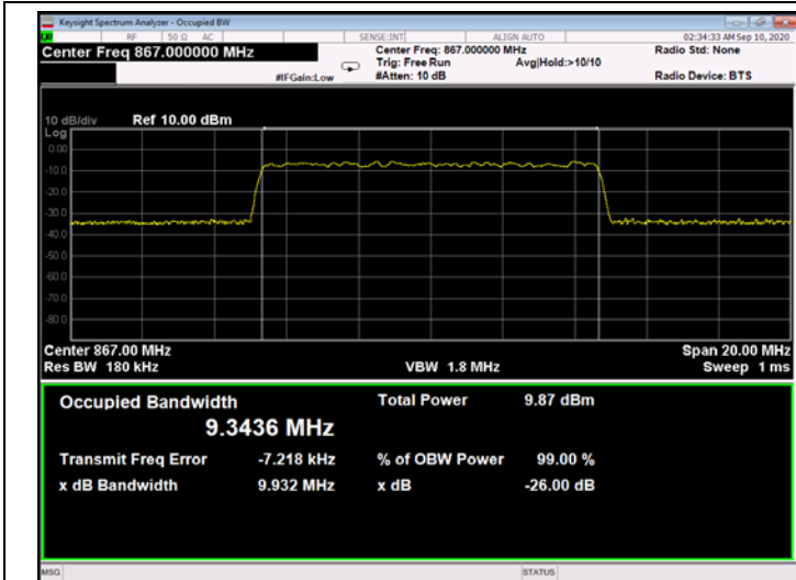
Figure 266: 256QAM 10MHz B.W.; 867.0MHz, 15kHz - Input
