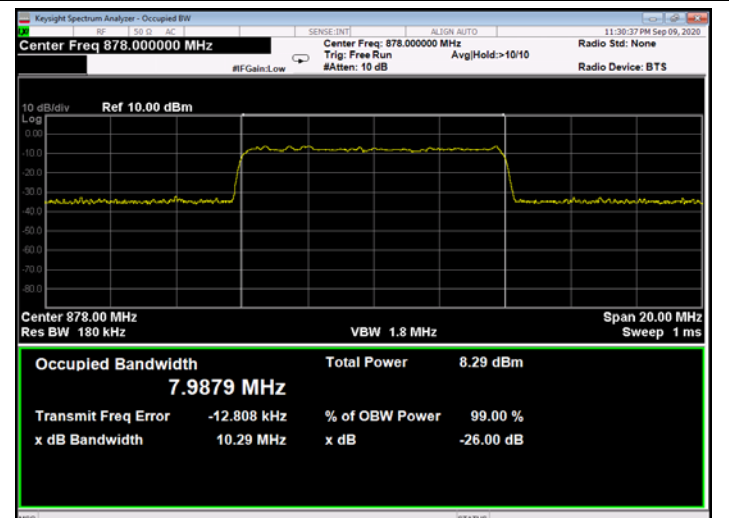
Figure 313: QPSK 10MHz B.W.; 878.0MHz, 60kHz - Input
