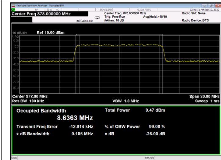
Figure 270: 256QAM 10MHz B.W.; 878.0MHz, 30kHz - Input
