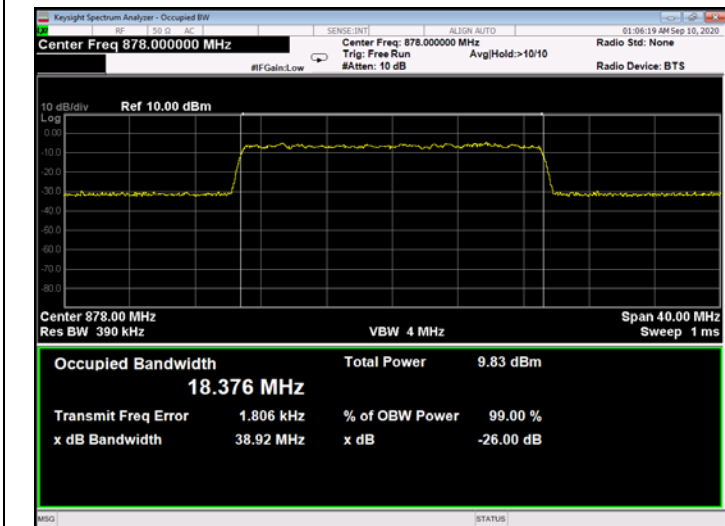
Figure 330: QPSK 20MHz B.W.; 878.0MHz, 30kHz - Input
