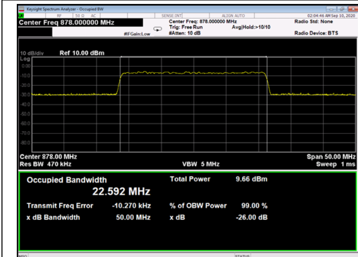
Figure 340: QPSK 25MHz B.W.; 878.0MHz, 60kHz - Input
