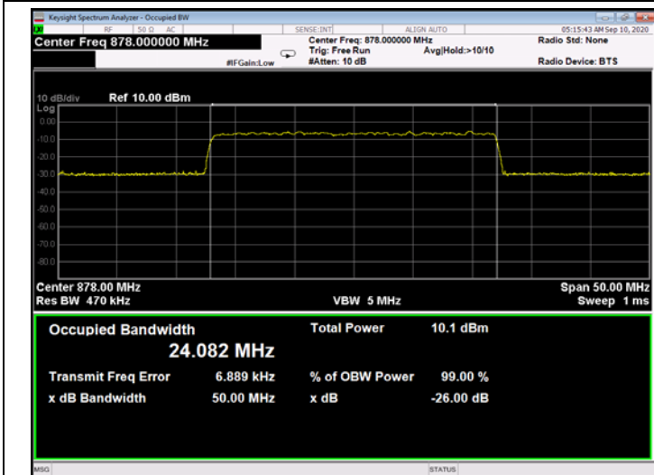
Figure 296: 256QAM 25MHz B.W.; 878.0MHz, 15kHz - Input
