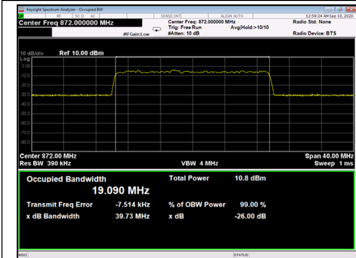
Figure 326: QPSK 20MHz B.W.; 872.0MHz, 15kHz - Input
