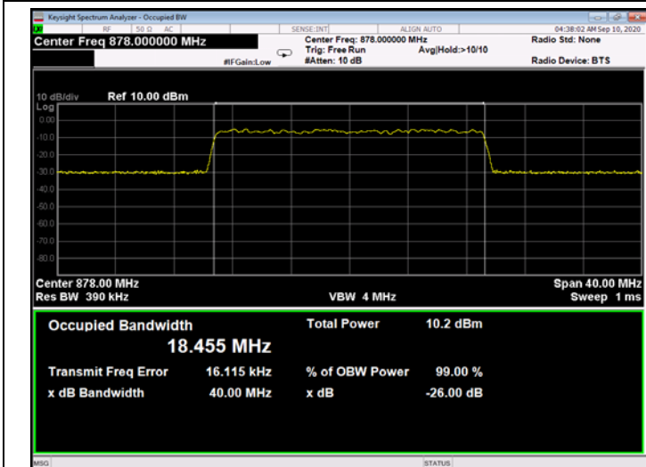
Figure 288: 256QAM 20MHz B.W.; 878.0MHz, 30kHz - Input
