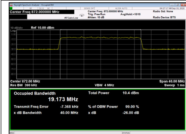
Figure 284: 256QAM 20MHz B.W.; 872.0MHz, 15kHz - Input
