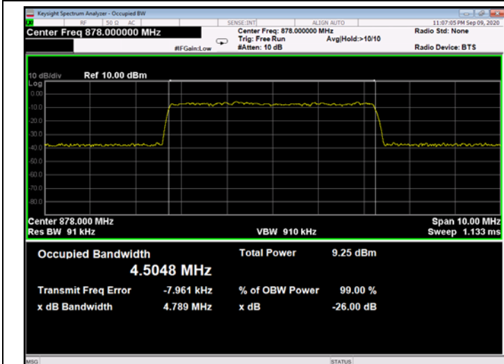
Figure 304: QPSK 5MHz B.W.; 878.0MHz, 15kHz - Input
