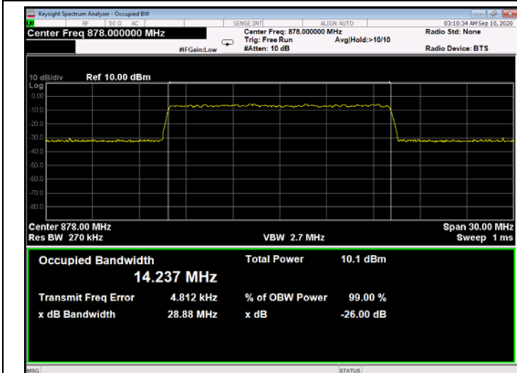
Figure 278: 256QAM 15MHz B.W.; 878.0MHz, 15kHz - Input
