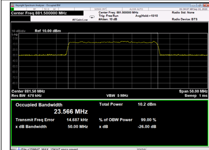
Figure 342: QPSK 25MHz B.W.; 881.5MHz, 30kHz - Input
