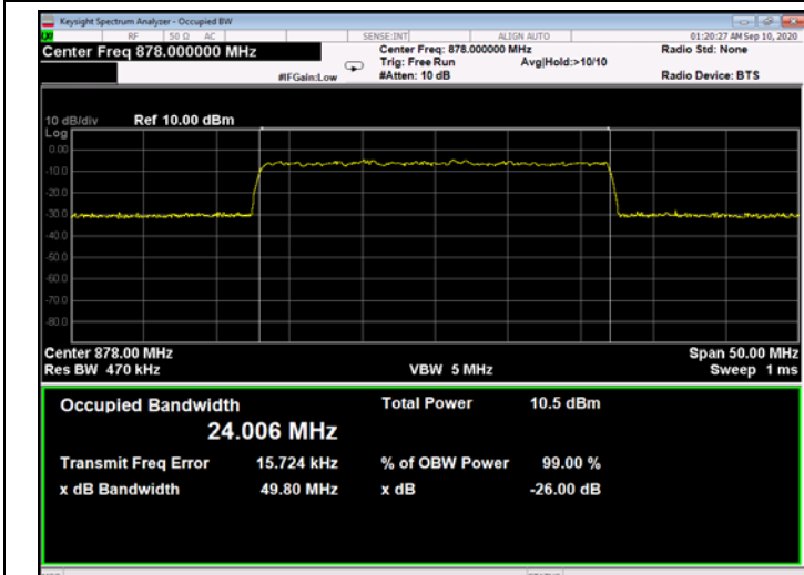
Figure 338: QPSK 25MHz B.W.; 878.0MHz, 15kHz - Input
