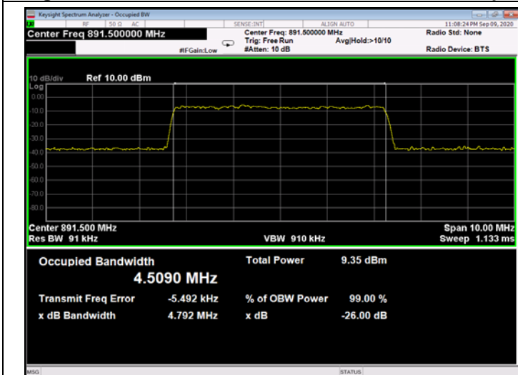
Figure 306: QPSK 5MHz B.W.; 891.50MHz, 15kHz - Input
