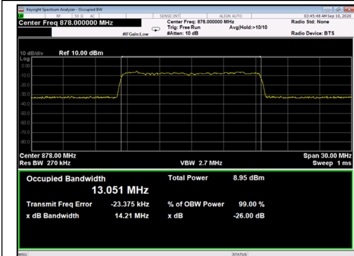
Figure 280: 256QAM 15MHz B.W.; 878.0MHz, 60kHz - Input
