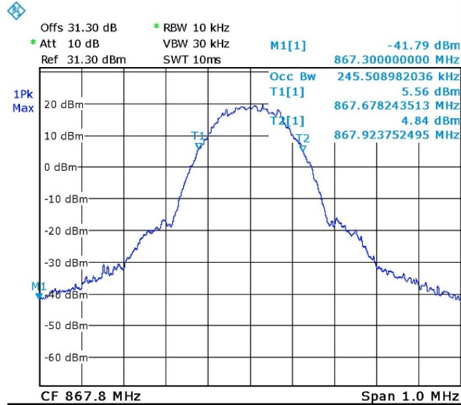
Figure 77. — 867.8MHz GSM Input
