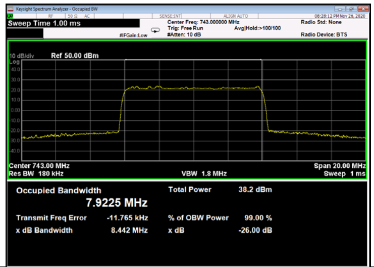
Figure 382: QPSK 10MHz B.W.; 743.0MHz, 60kHz - Output
