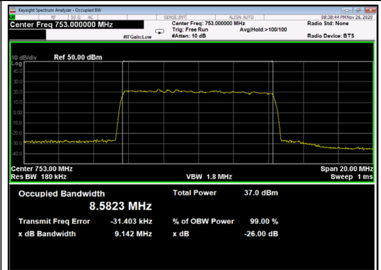
Figure 384: QPSK 10MHz B.W.; 753.0MHz, 30kHz - Output
