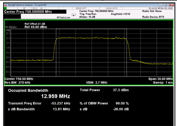
Figure 394: QPSK 15MHz B.W.; 750.5MHz, 60kHz - Output
