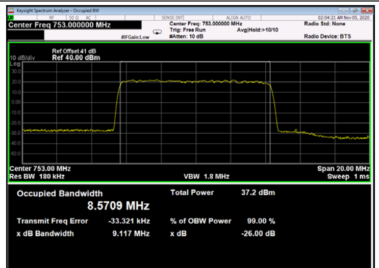
Figure 351: 256QAM 10MHz B.W.; 753.0MHz, 30kHz - Output
