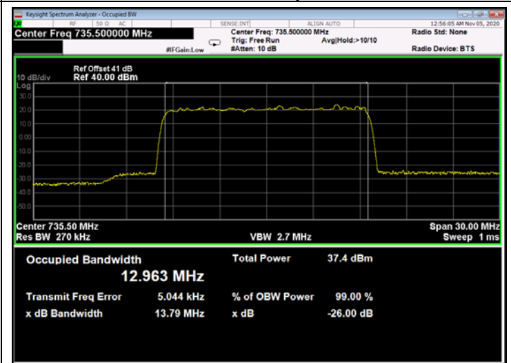
Figure 388: QPSK 15MHz B.W.; 735.5MHz, 60kHz - Output
