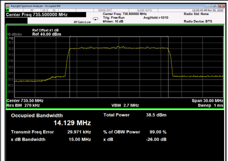
Figure 386: QPSK 15MHz B.W.; 735.5MHz, 15kHz - Output
