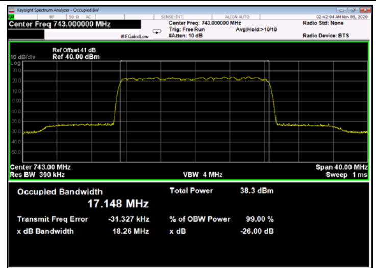
Figure 367: 256QAM 20MHz B.W.; 743.0MHz, 60kHz - Output
