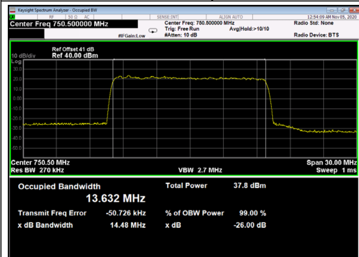
Figure 393: QPSK 15MHz B.W.; 750.5MHz, 30kHz - Output
