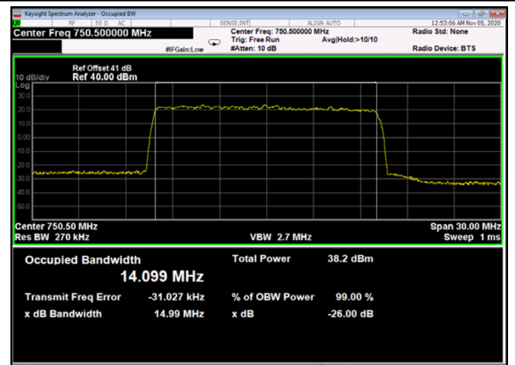
Figure 392: QPSK 15MHz B.W.; 750.5MHz, 15kHz - Output
