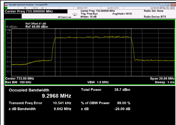
Figure 377: QPSK 10MHz B.W.; 733.0MHz, 15kHz - Output
