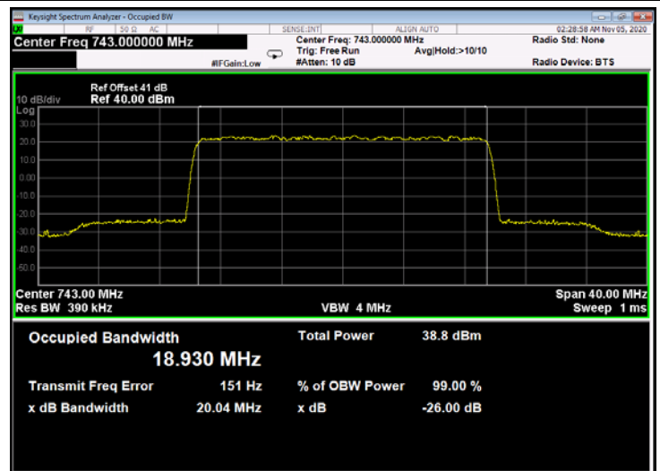
Figure 365: 256QAM 20MHz B.W.; 743.0MHz, 15kHz - Output
