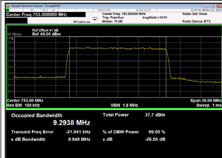
Figure 383: QPSK 10MHz B.W.; 753.0MHz, 15kHz - Output
