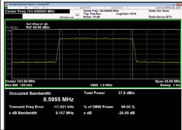
Figure 381: QPSK 10MHz B.W.; 743.0MHz, 30kHz - Output
