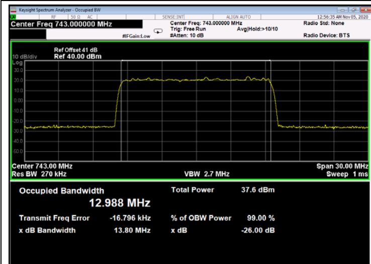
Figure 391: QPSK 15MHz B.W.; 743.0MHz, 60kHz - Output
