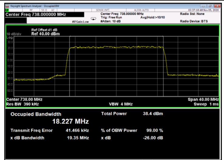
Figure 363: 256QAM 20MHz B.W.; 738.0MHz, 30kHz - Output
