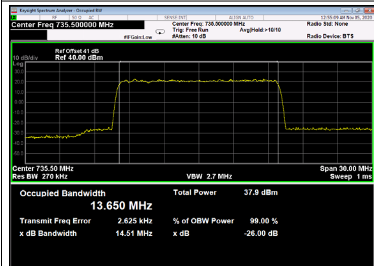
Figure 387: QPSK 15MHz B.W.; 735.5MHz, 30kHz - Output
