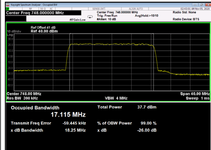
Figure 370: 256QAM 20MHz B.W.; 748.0MHz, 60kHz - Output
