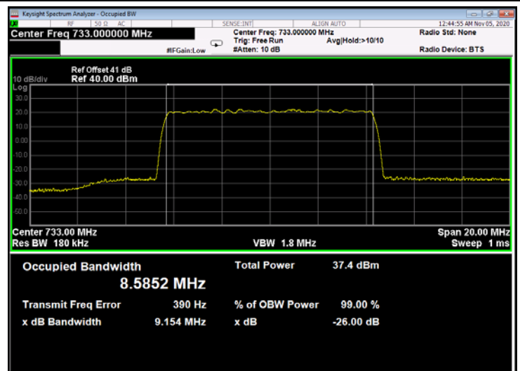
Figure 378: QPSK 10MHz B.W.; 733.0MHz, 30kHz - Output
