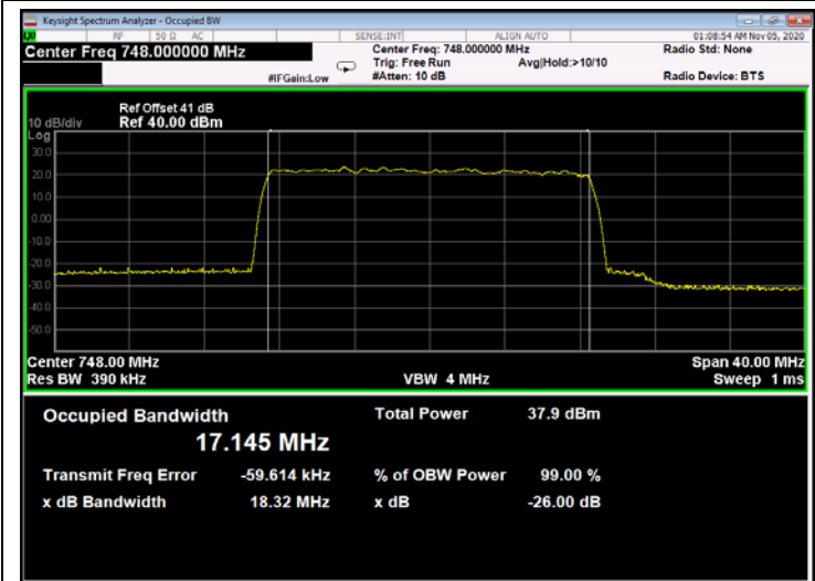
Figure 403: QPSK 20MHz B.W.; 748.0MHz, 60kHz - Output
