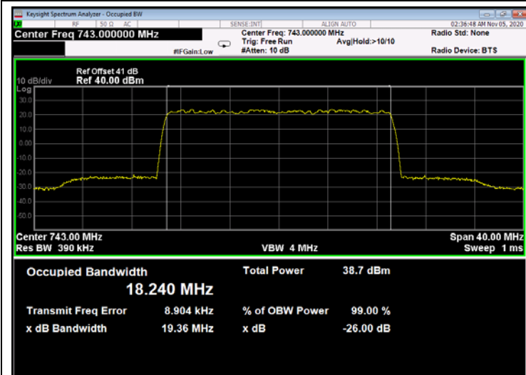
Figure 366: 256QAM 20MHz B.W.; 743.0MHz, 30kHz - Output
