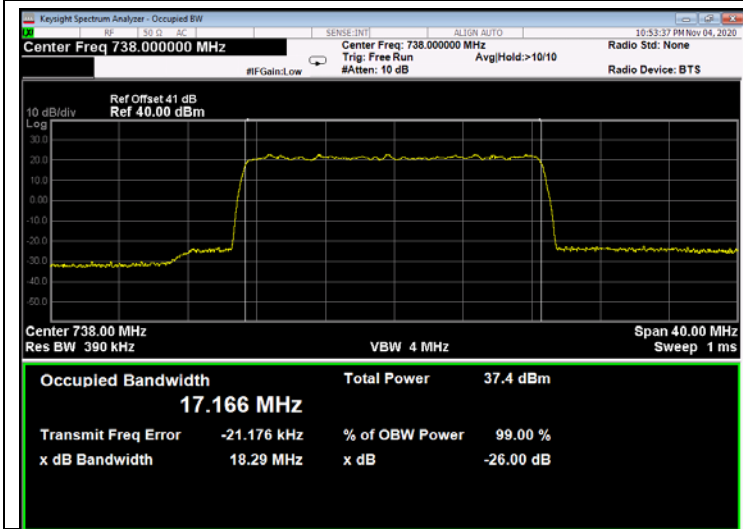
Figure 331: 64QAM 20MHz B.W.; 738.0MHz, 60kHz - Output
