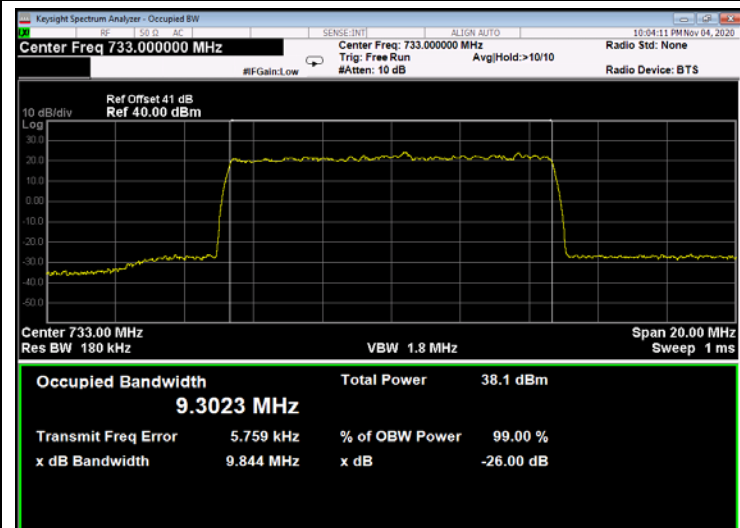
Figure 311: 64QAM 10MHz B.W.; 733.0MHz, 15kHz - Output
