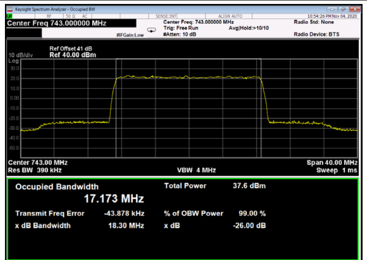
Figure 334: 64QAM 20MHz B.W.; 743.0MHz, 60kHz - Output
