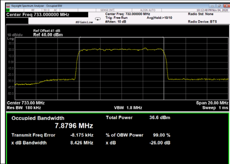
Figure 313: 64QAM 10MHz B.W.; 733.0MHz, 60kHz - Output
