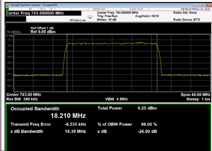
Figure 267: QPSK 20MHz B.W.; 743.0MHz, 30kHz - Input
