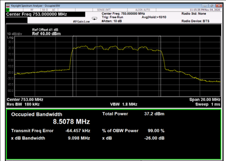
Figure 285: 16QAM 10MHz B.W.; 753.0MHz, 30kHz - Output
