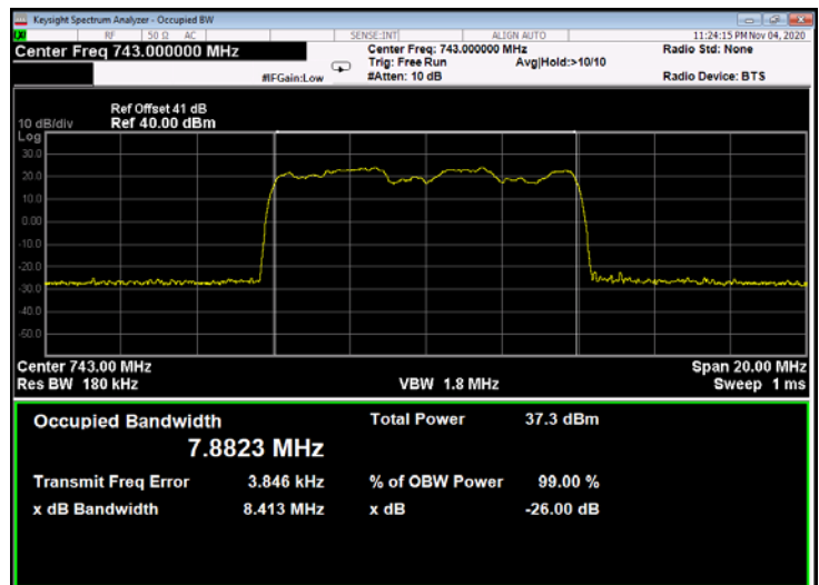
Figure 283: 16QAM 10MHz B.W.; 743.0MHz, 60kHz - Output
