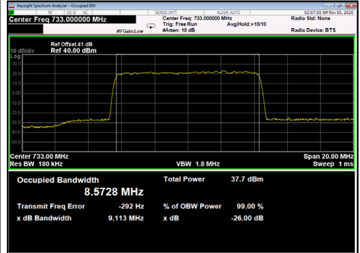
Figure 345: 256QAM 10MHz B.W.; 733.0MHz, 30kHz - Output
