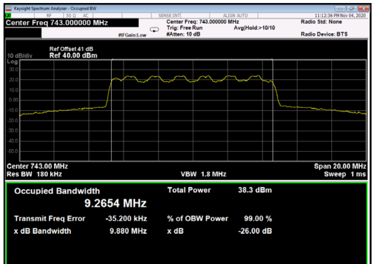
Figure 281: 16QAM 10MHz B.W.; 743.0MHz, 15kHz- Output
