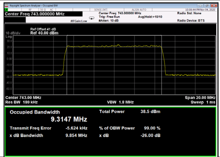
Figure 314: 64QAM 10MHz B.W.; 743.0MHz, 15kHz - Output
