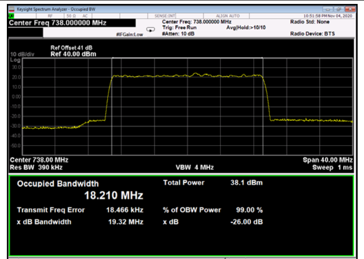
Figure 330: 64QAM 20MHz B.W.; 738.0MHz, 30kHz - Output
