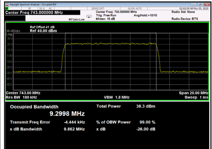
Figure 347: 256QAM 10MHz B.W.; 743.0MHz, 15kHz - Output
