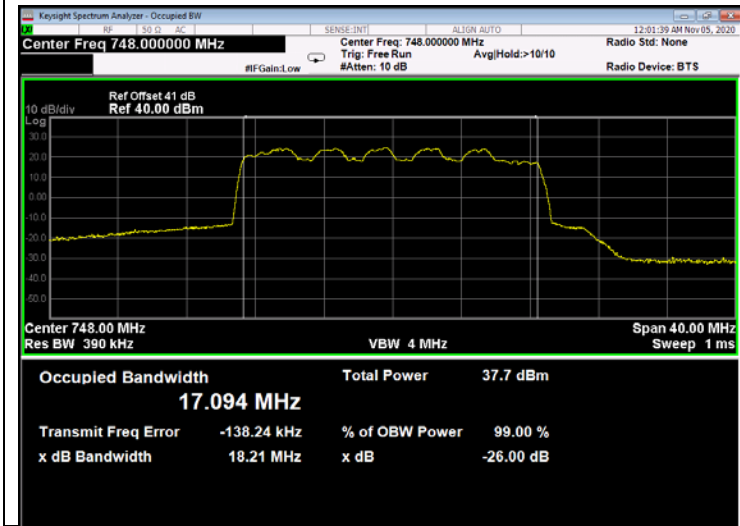
Figure 304: 16QAM 20MHz B.W.; 748.0MHz, 60kHz - Output
