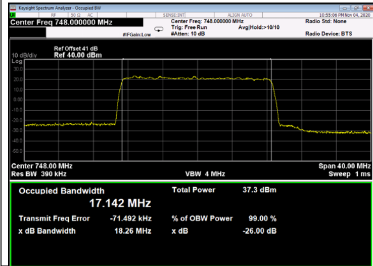
Figure 337: 64QAM 20MHz B.W.; 748.0MHz, 60kHz Output
