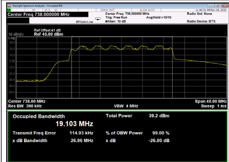
Figure 296: 16QAM 20MHz B.W.; 738.0MHz, 15kHz - Output
