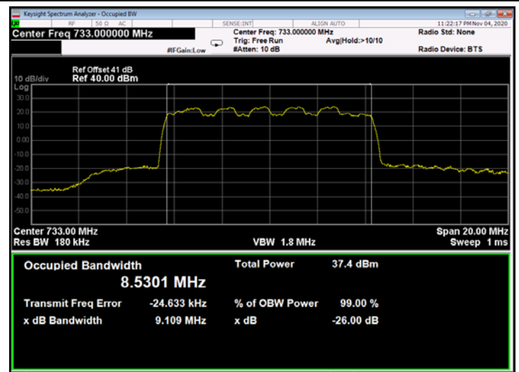
Figure 279: 16QAM 10MHz B.W.; 733.0MHz, 30kHz- Output
