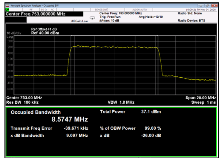
Figure 318: 64QAM 10MHz B.W.; 753.0MHz, 30kHz - Output
