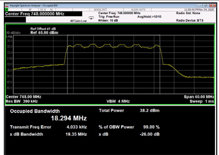
Figure 303: 16QAM 20MHz B.W.; 748.0MHz, 30kHz - Output
