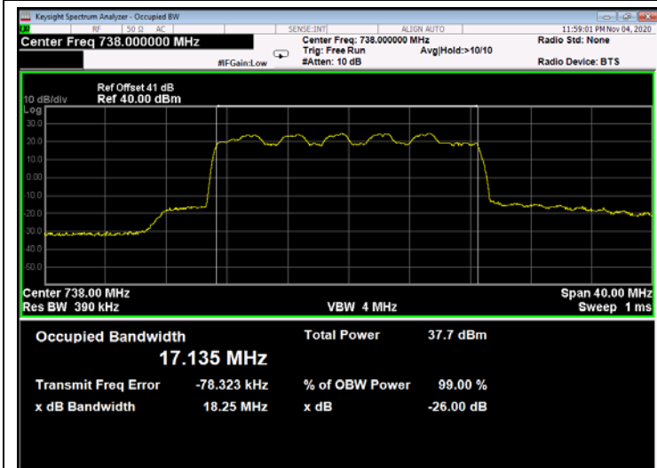
Figure 298: 16QAM 20MHz B.W.; 738.0MHz, 60kHz - Output
