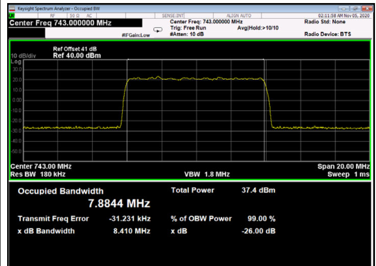
Figure 349: 256QAM 10MHz B.W.; 743.0MHz, 60kHz - Output
