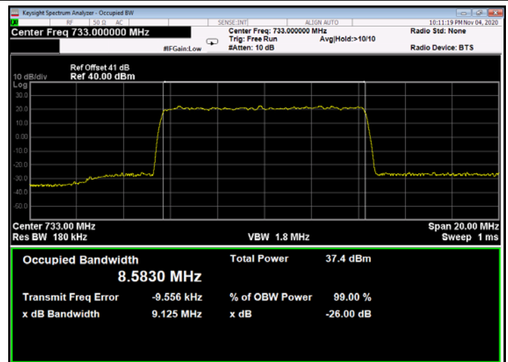
Figure 312: 64QAM 10MHz B.W.; 733.0MHz, 30kHz - Output
