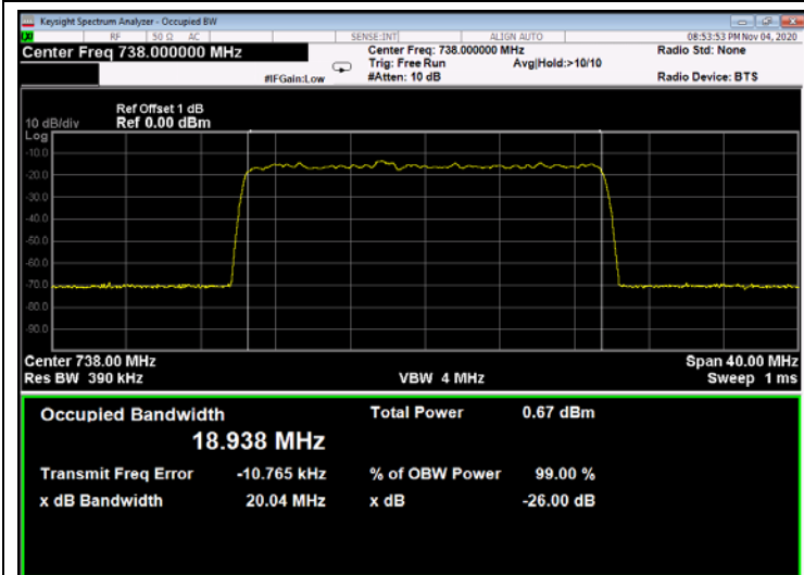
Figure 263: QPSK 20MHz B.W.; 738.0MHz, 15kHz - Input
