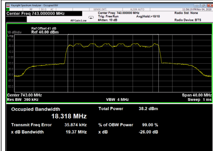
Figure 300: 16QAM 20MHz B.W.; 743.0MHz, 30kHz - Output
