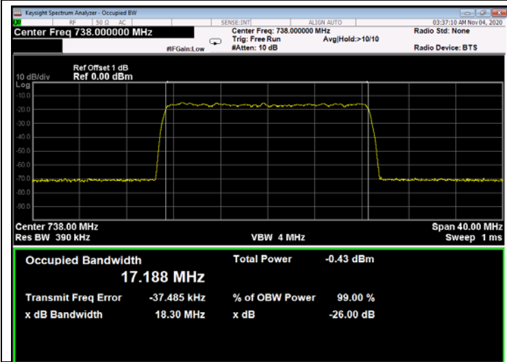
Figure 199: 64QAM 20MHz B.W.; 738.0MHz, 60kHz - Input
