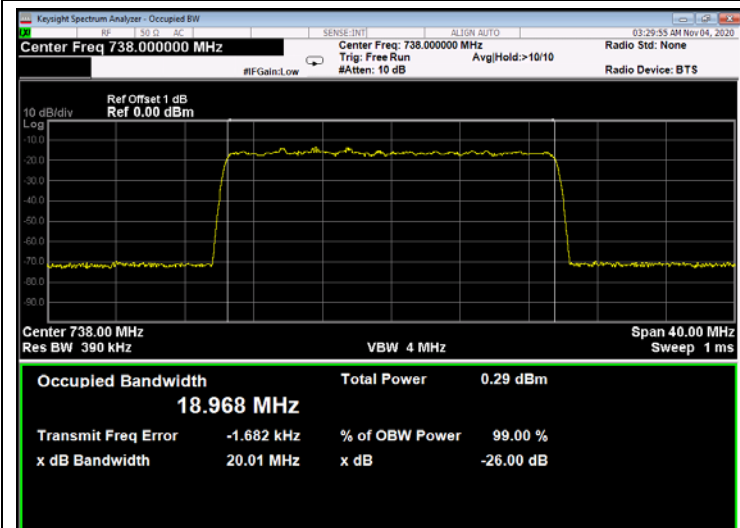
Figure 197: 64QAM 20MHz B.W.; 738.0MHz, 15kHz - Input
