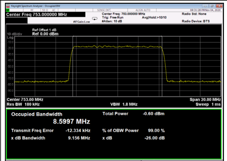
Figure 252: QPSK 10MHz B.W.; 753.0MHz, 30kHz - Input
