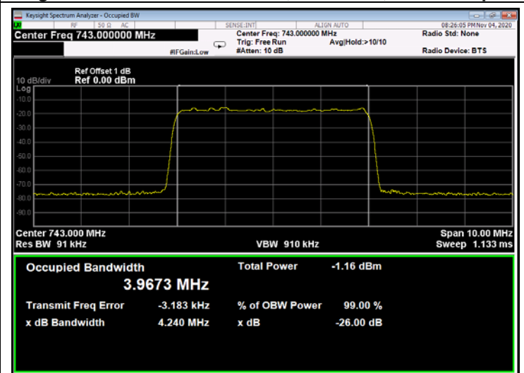
Figure 242: QPSK 5MHz B.W.; 743.0MHz, 30kHz - Input
