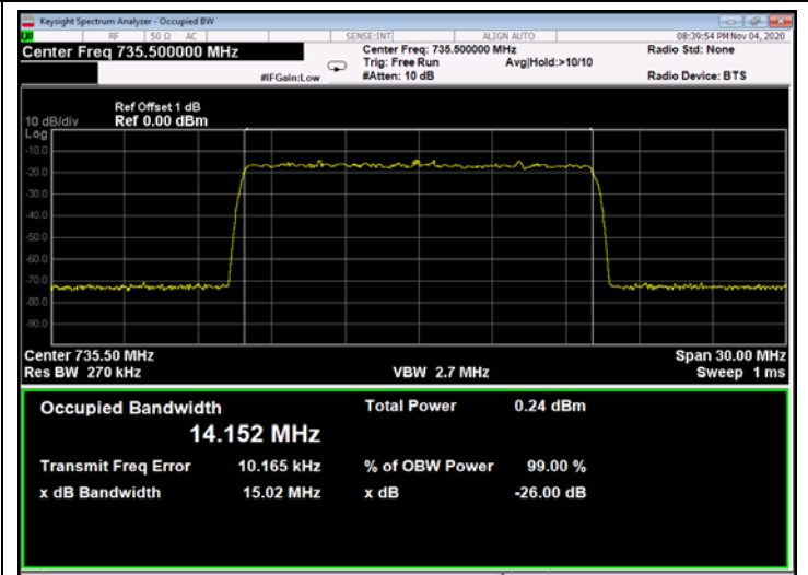
Figure 254: QPSK 15MHz B.W.; 735.5MHz, 15kHz - Input
