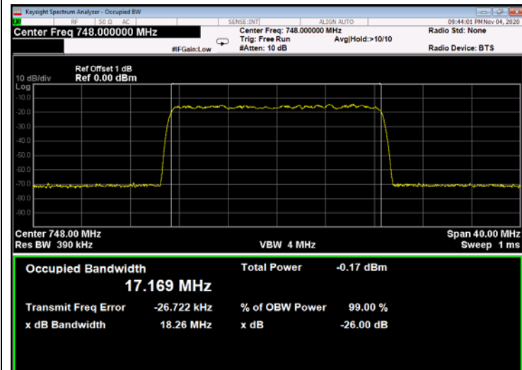
Figure 238: 256QAM 20MHz B.W.; 748.0MHz, 60kHz - Input
