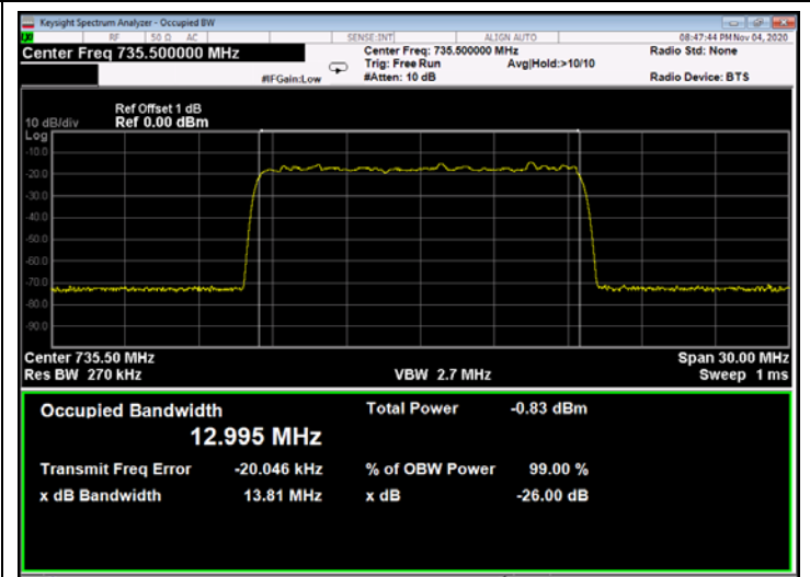
Figure 256: QPSK 15MHz B.W.; 735.5MHz, 60kHz - Input
