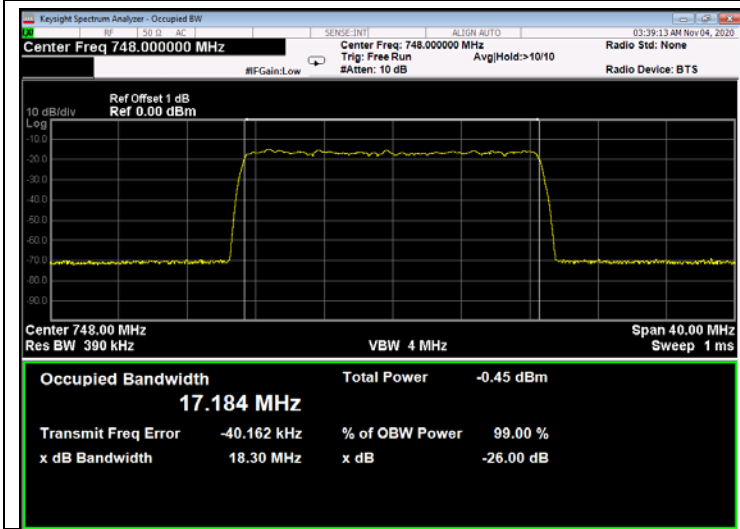
Figure 205: 64QAM 20MHz B.W.; 748.0MHz, 60kHz - Input
