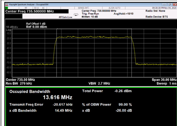
Figure 222: 256QAM 15MHz B.W.; 735.5MHz, 30kHz - Input
