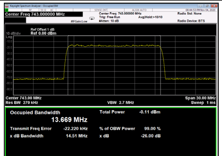
Figure 258: QPSK 15MHz B.W.; 743.0MHz, 30kHz - Input
