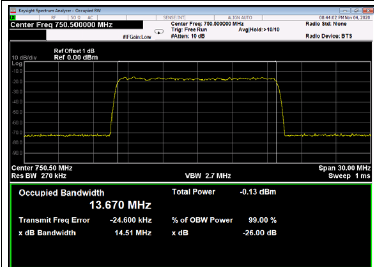
Figure 261: QPSK 15MHz B.W.; 750.5MHz, 30kHz - Input
