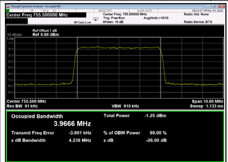
Figure 244: QPSK 5MHz B.W.; 755.5MHz, 30kHz - Input
