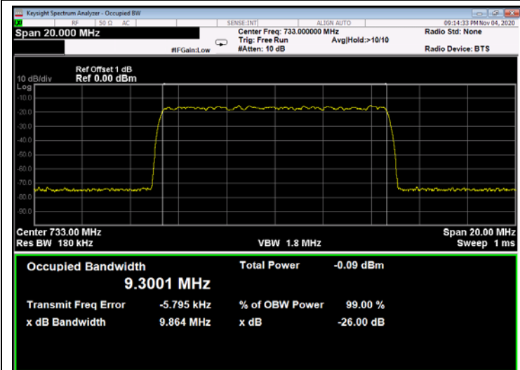
Figure 212: 256QAM 10MHz B.W.; 733.0MHz, 15kHz - Input
