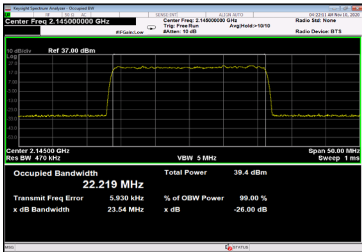
Figure 377: 64QAM 25MHz B.W.; 2145.0MHz, 60kHz - Input
