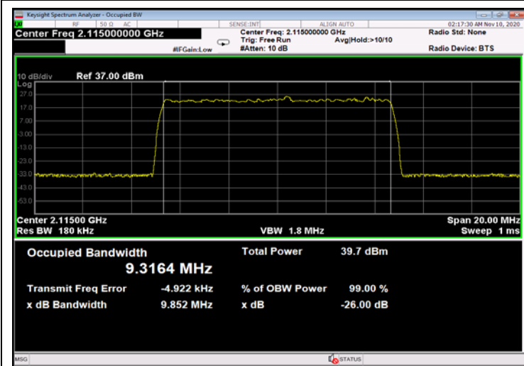
Figure 345: 64QAM 10MHz B.W.; 2115.00MHz, 15kHz - Input
