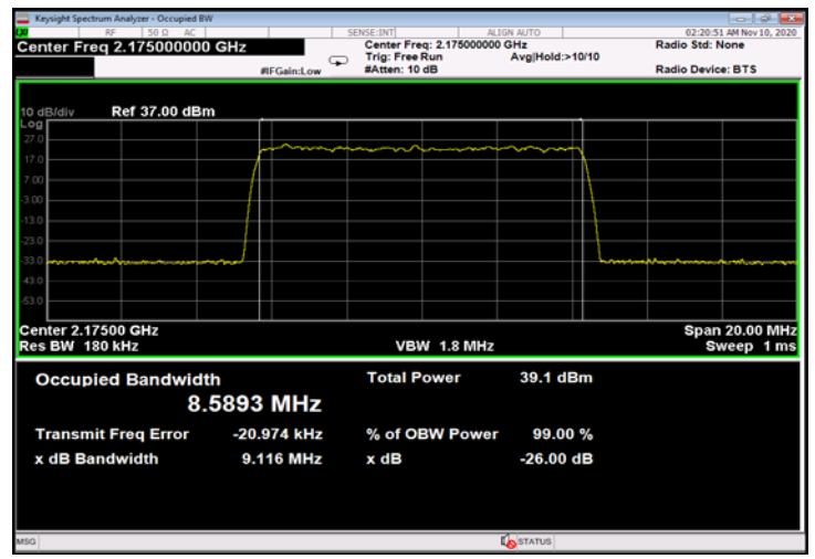
Figure 352: 64QAM 10MHz B.W.; 2175.0MHz, 30kHz - Input
