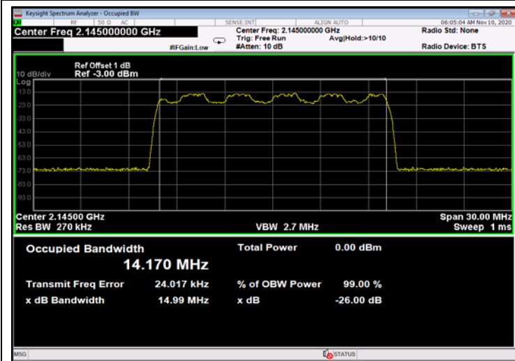
Figure 291: 16QAM 15MHz B.W.; 2145.0MHz, 15kHz - Input
