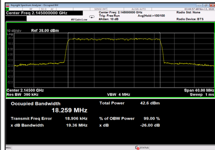
Figure 697: 256QAM 20MHz B.W.; 2145.0MHz, 30kHz - Output
