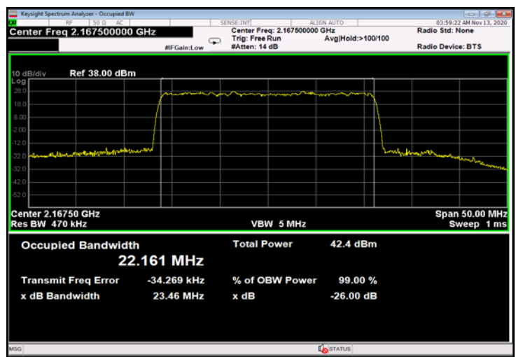
Figure 710: 256QAM 25MHz B.W.; 2167.5MHz, 60kHz - Output
