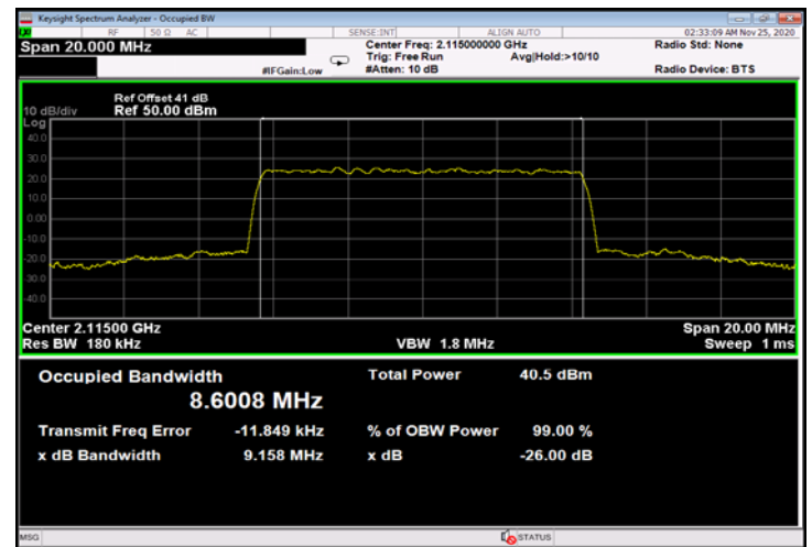
Figure 742: QPSK 10MHz B.W.; 2115.0MHz, 30kHz - Output
