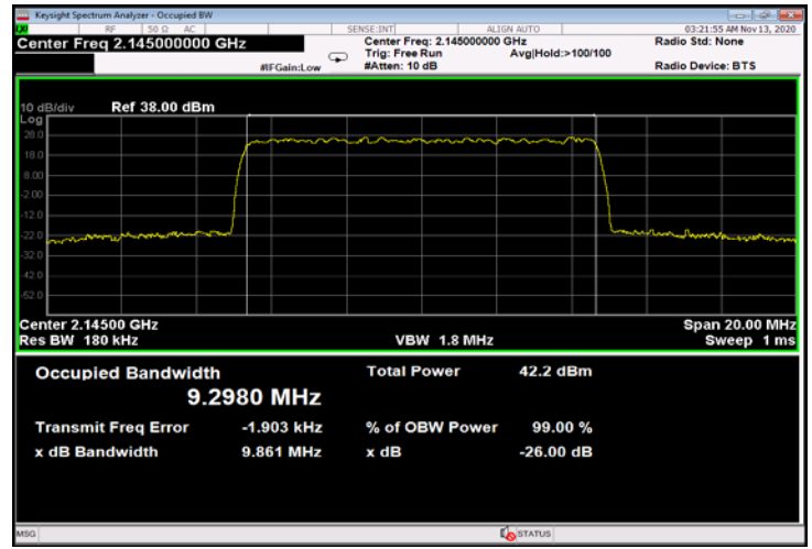
Figure 678: 256QAM 10MHz B.W.; 2145.0MHz, 15kHz - Output
