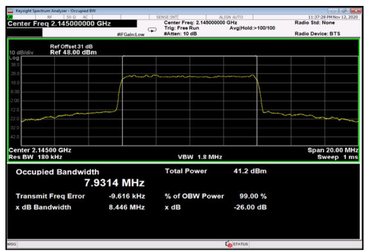
Figure 746: QPSK 10MHz B.W.; 2145.0MHz, 60kHz - Output
