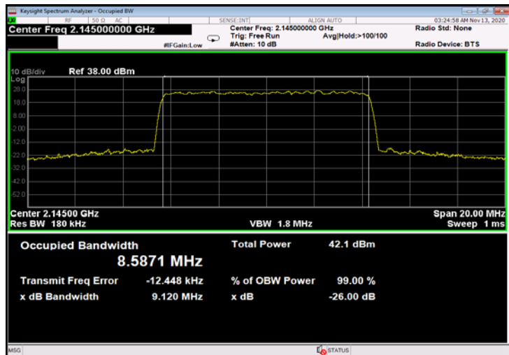
Figure 679: 256QAM 10MHz B.W.; 2145.0MHz, 30kHz - Output
