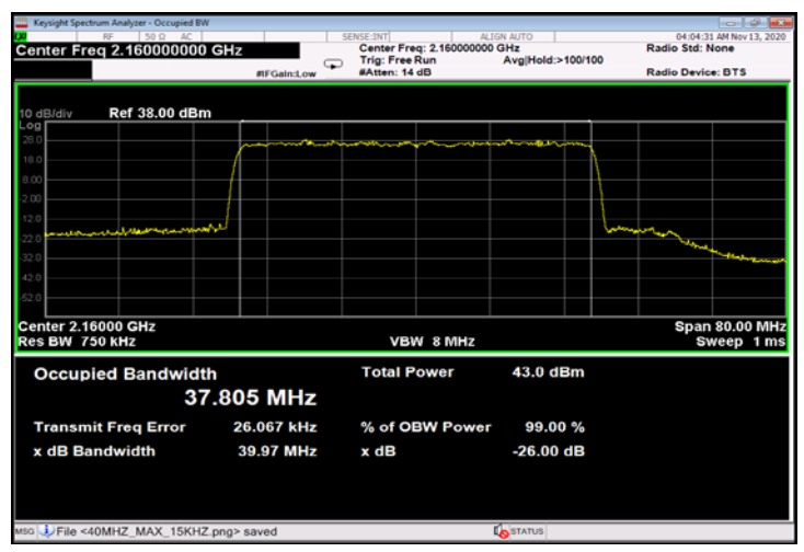
Figure 718: 256QAM 40MHz B.W.; 2160.0MHz, 30kHz - Output
