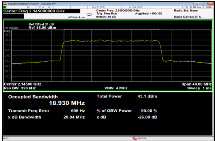
Figure 762: QPSK 20MHz B.W.; 2145.0MHz, 15kHz - Output
