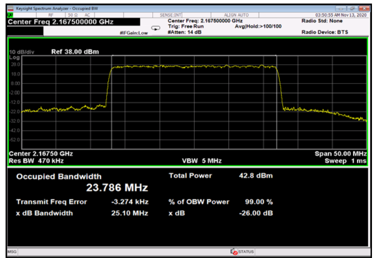
Figure 708: 256QAM 25MHz B.W.; 2167.5MHz, 15kHz - Output
