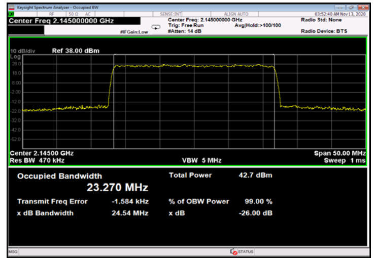
Figure 706: 256QAM 25MHz B.W.; 2145.0MHz, 30kHz - Output
