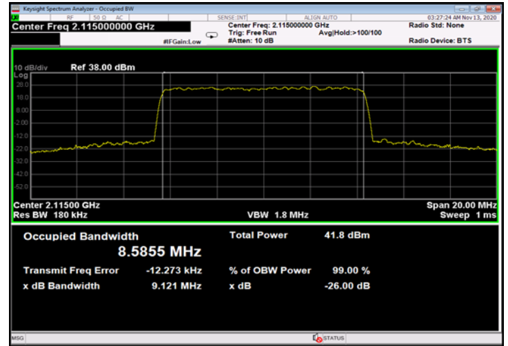
Figure 676: 256QAM 10MHz B.W.; 2115.0MHz, 30kHz - Output
