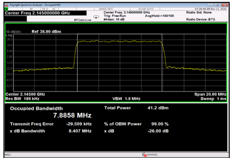
Figure 680: 256QAM 10MHz B.W.; 2145.0MHz, 60kHz - Output
