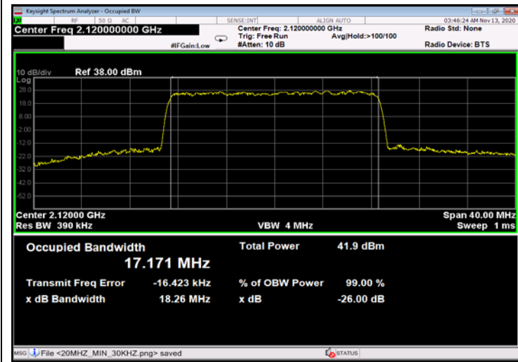
Figure 695: 256QAM 20MHz B.W.; 2120.0MHz, 60kHz - Output
