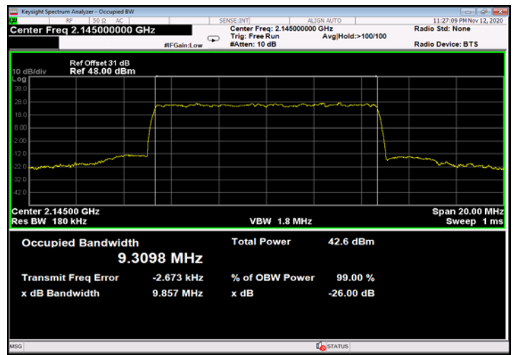
Figure 744: QPSK 10MHz B.W.; 2145.0MHz, 15kHz - Output
