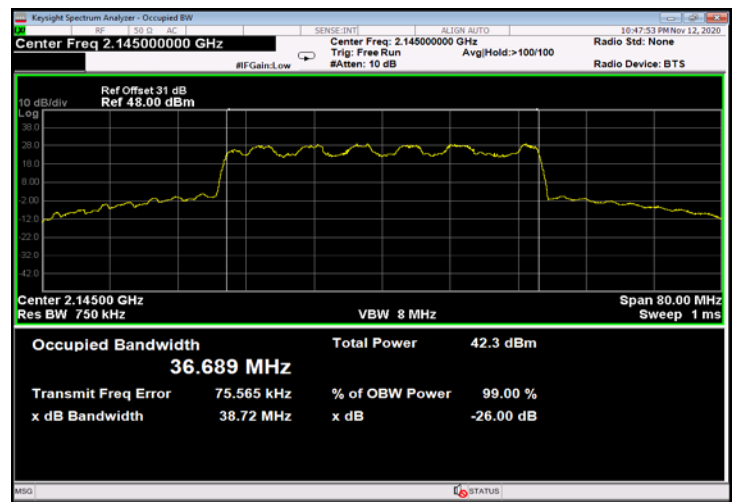
Figure 584: 16QAM 40MHz B.W.; 2145.0MHz, 60kHz - Output
