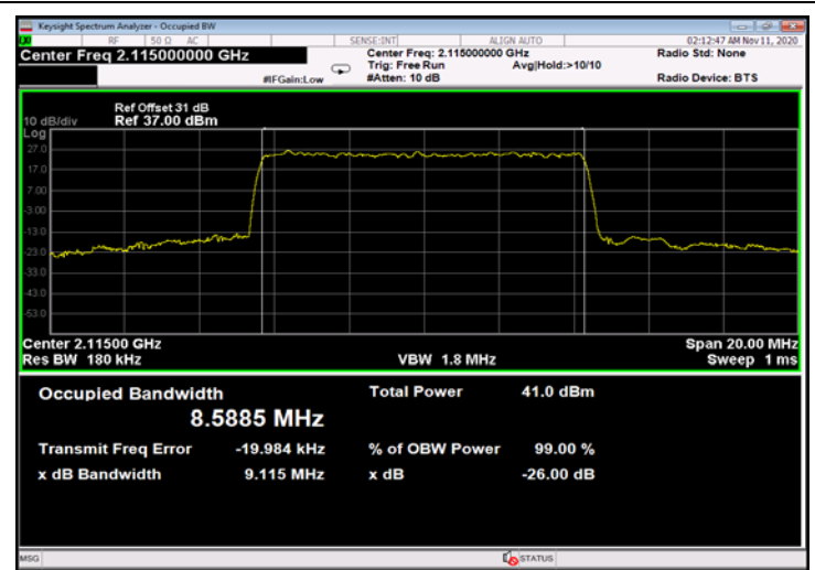
Figure 610: 64QAM 10MHz B.W.; 2115.0MHz, 30kHz - Output
