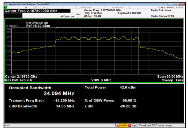
Figure 576: 16QAM 25MHz B.W.; 2167.5MHz, 15kHz - Output
