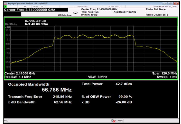
Figure 598: 16QAM 60MHz B.W.; 2140.0MHz, 60kHz - Output
