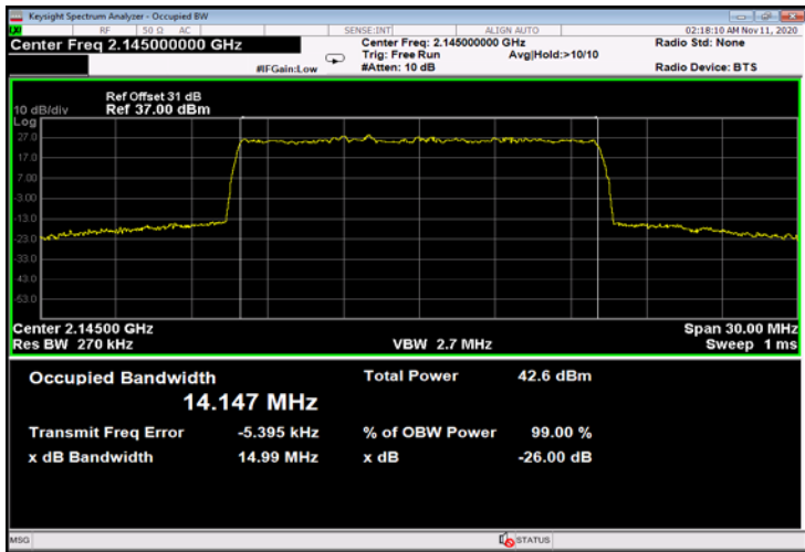
Figure 621: 64QAM 15MHz B.W.; 2145.0MHz, 15kHz - Output
