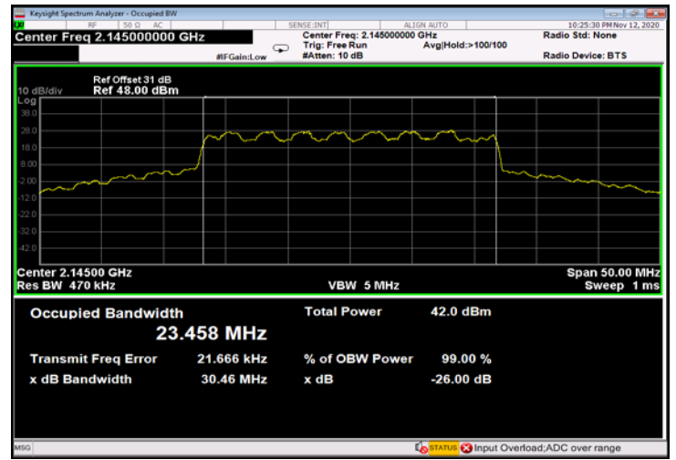
Figure 574: 16QAM 25MHz B.W.; 2145.0MHz, 30kHz - Output
