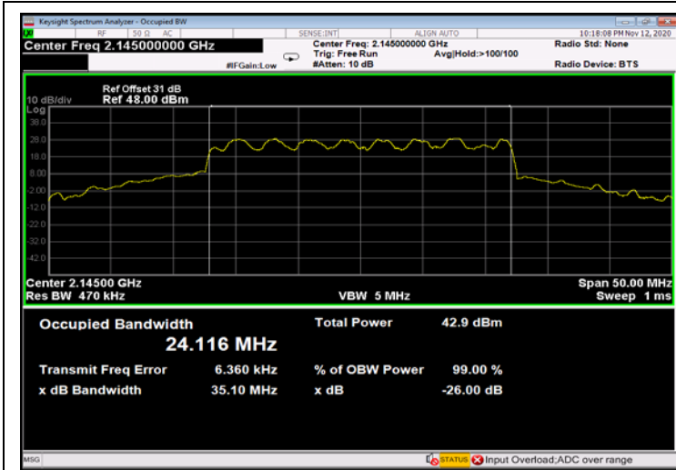
Figure 573: 16QAM 25MHz B.W.; 2145.0MHz, 15kHz - Output
