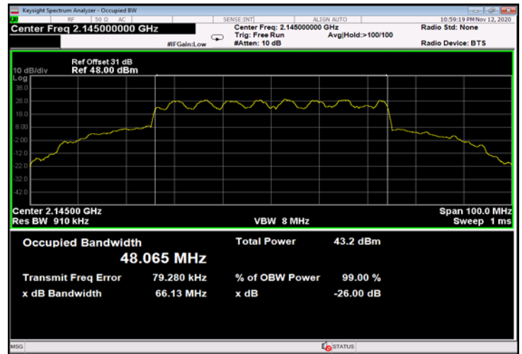
Figure 592: 16QAM 50MHz B.W.; 2145.0MHz, 30kHz - Output
