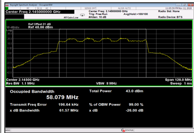
Figure 599: 16QAM 60MHz B.W.; 2145.0MHz, 30kHz - Output
