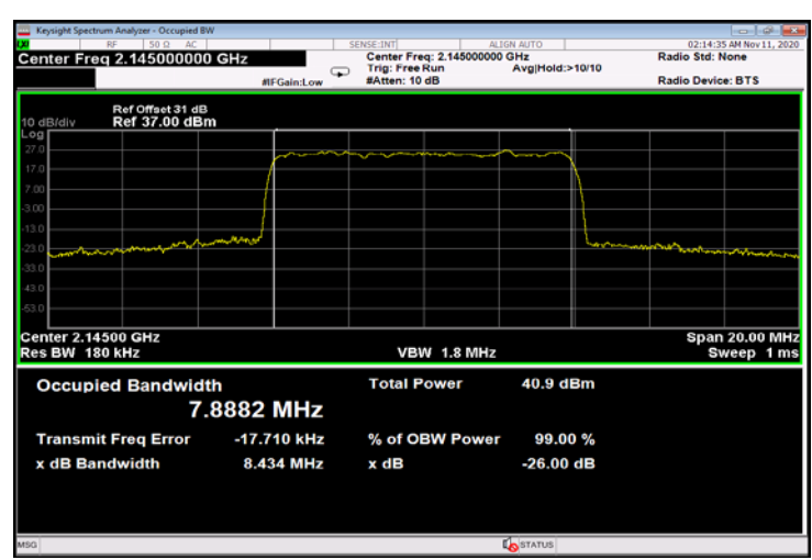
Figure 614: 64QAM 10MHz B.W.; 2145.0MHz, 60kHz - Output
