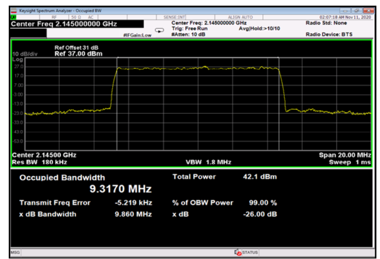
Figure 612: 64QAM 10MHz B.W.; 2145.0MHz, 15kHz - Output
