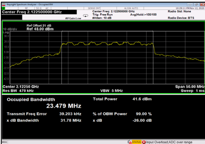
Figure 571: 16QAM 25MHz B.W.; 2122.5MHz, 30kHz - Output
