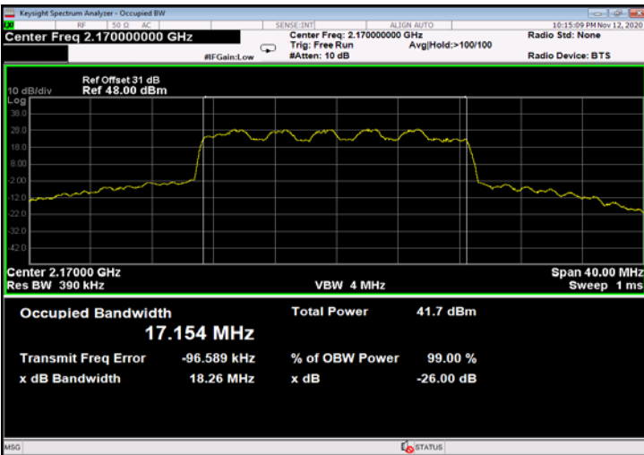
Figure 569: 16QAM 20MHz B.W.; 2170.0MHz, 60kHz - Output
