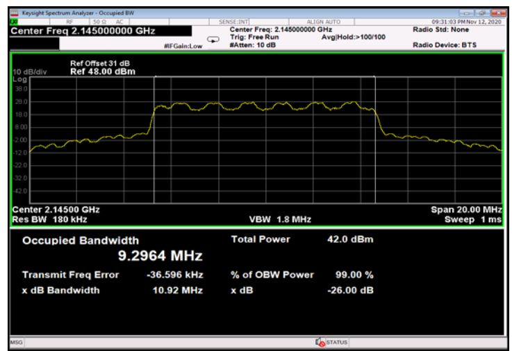
Figure 546: 16QAM 10MHz B.W.; 2145.0MHz, 15kHz - Output
