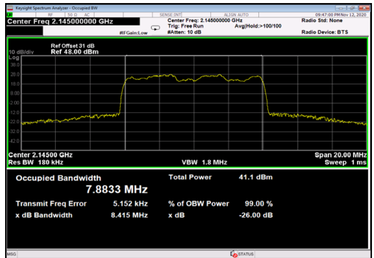
Figure 548: 16QAM 10MHz B.W.; 2145.0MHz, 60kHz - Output
