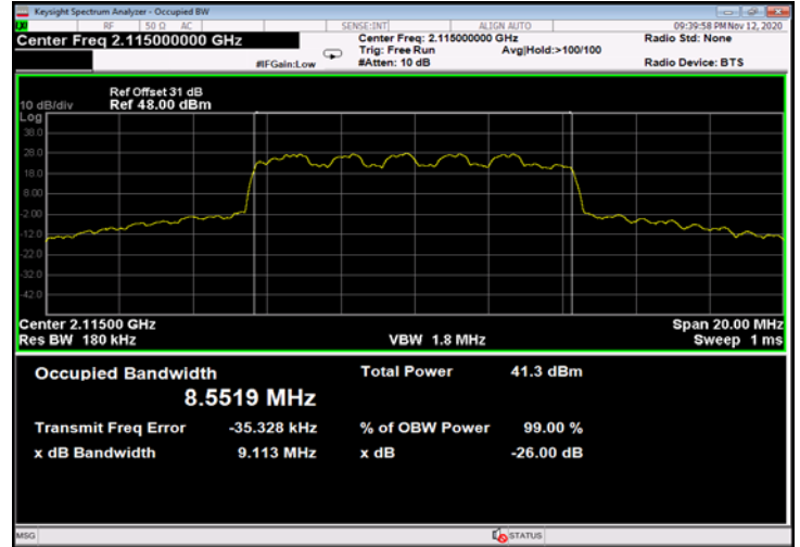
Figure 544: 16QAM 10MHz B.W.; 2115.0MHz, 30kHz - Output
