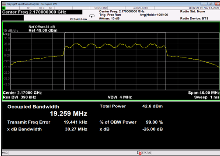
Figure 567: 16QAM 20MHz B.W.; 2170.0MHz, 15kHz - Output
