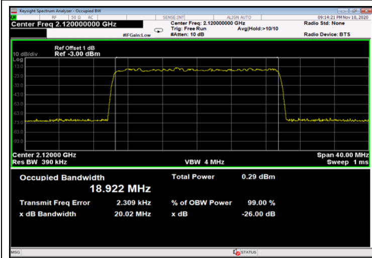
Figure 495: QPSK 20MHz B.W.; 2120.0MHz, 15kHz - Input
