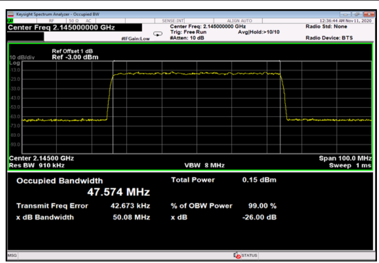
Figure 460: 256QAM 50MHz B.W.; 2145.0MHz, 30kHz - Input
