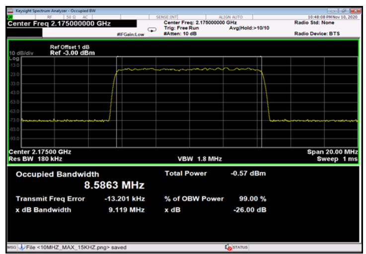
Figure 418: 256QAM 10MHz B.W.; 2175.0MHz, 30kHz - Input
