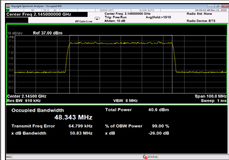
Figure 393: 64QAM 50MHz B.W.; 2145.0MHz, 15kHz - Input
