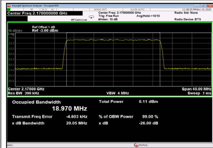
Figure 435: 256QAM 20MHz B.W.; 2170.0MHz, 15kHz - Input
