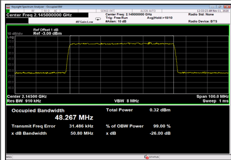
Figure 459: 256QAM 50MHz B.W.; 2145.0MHz, 15kHz - Input
