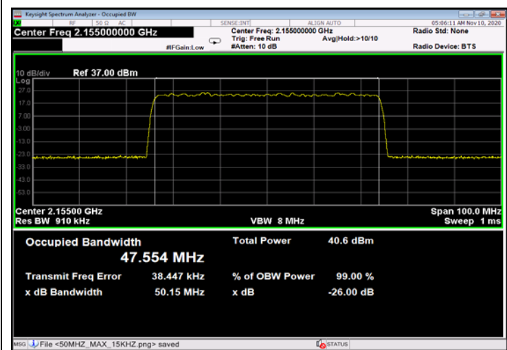
Figure 397: 64QAM 50MHz B.W.; 2155.0MHz, 30kHz - Input
