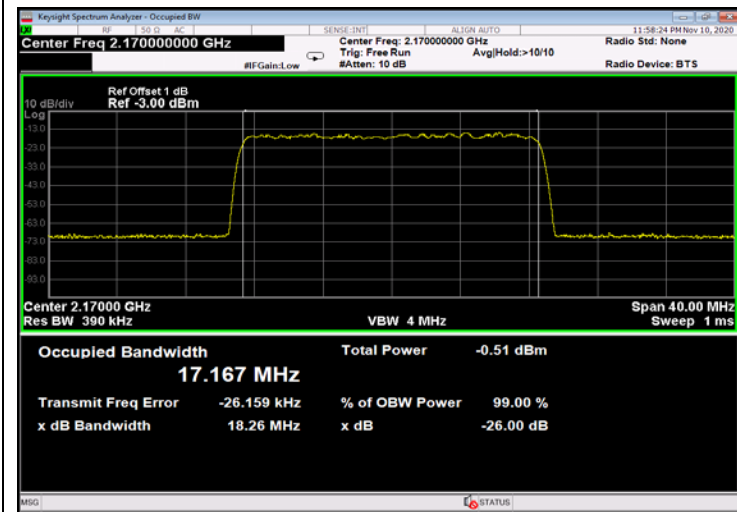
Figure 437: 256QAM 20MHz B.W.; 2170.0MHz, 60kHz - Input
