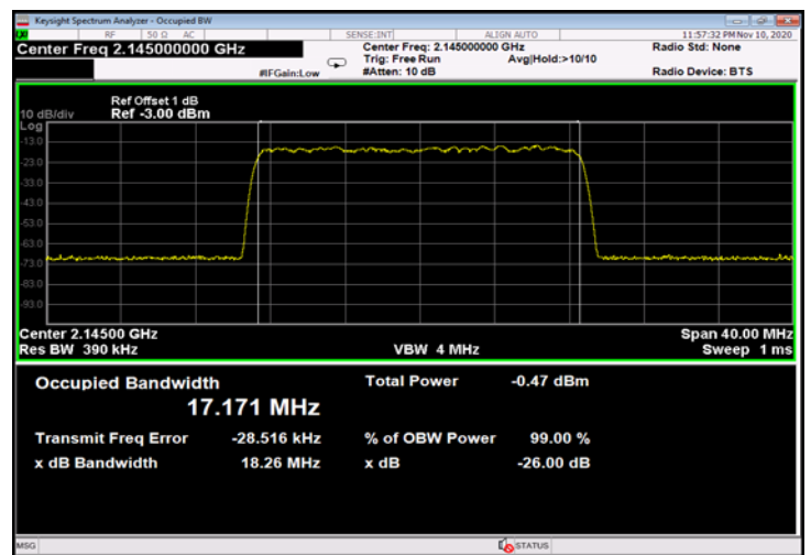
Figure 434: 256QAM 20MHz B.W.; 2145.0MHz, 60kHz - Input
