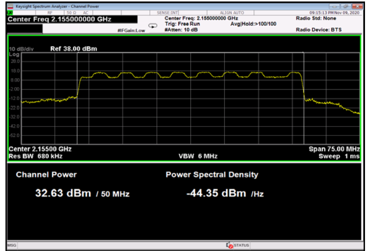
Figure 66: 16QAM 50MHz B.W.; 2155.0MHz, 15kHz
