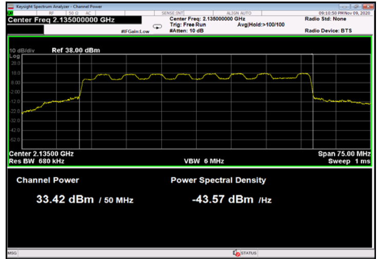
Figure 60: 16QAM 50MHz B.W.; 2135.0MHz, 15kHz
