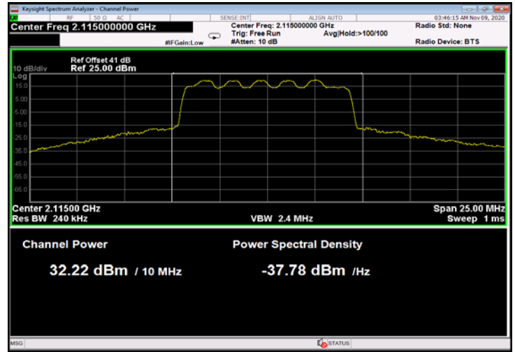
Figure 16: 16QAM 10MHz B.W.; 2115.0MHz, 30kHz
