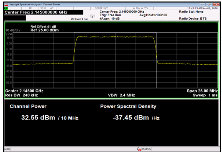
Figure 84: 64QAM 10MHz B.W.; 2145MHz, 15kHz
