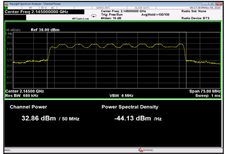
Figure 64: 16QAM 50MHz B.W.; 2145.0MHz, 30kHz
