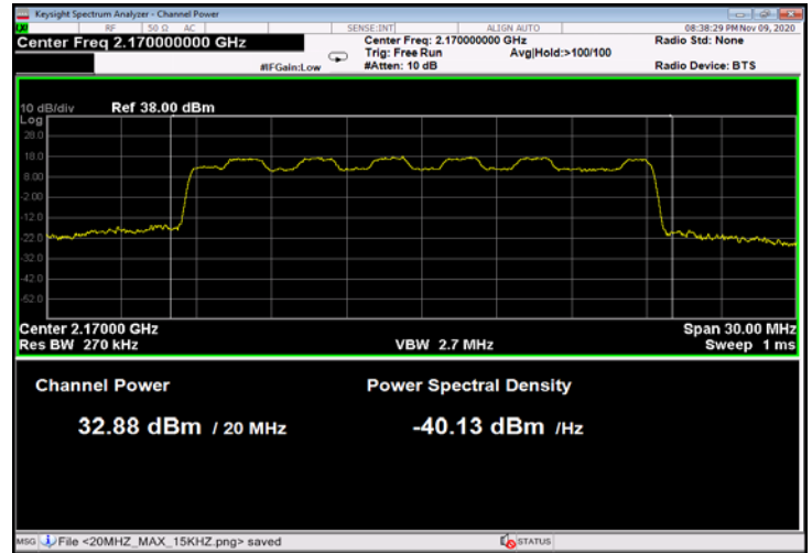
Figure 40: 16QAM 20MHz B.W.; 2170.0MHz, 30kHz
