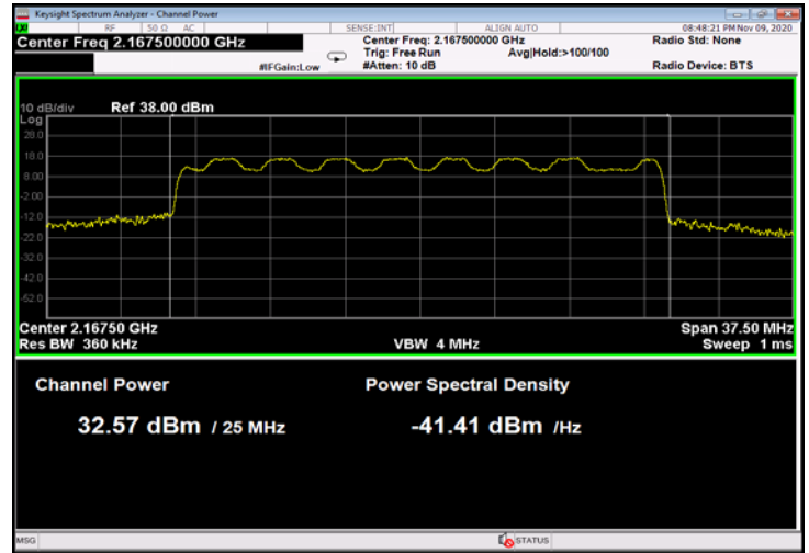
Figure 48: 16QAM 25MHz B.W.; 2167.5MHz, 15kHz
