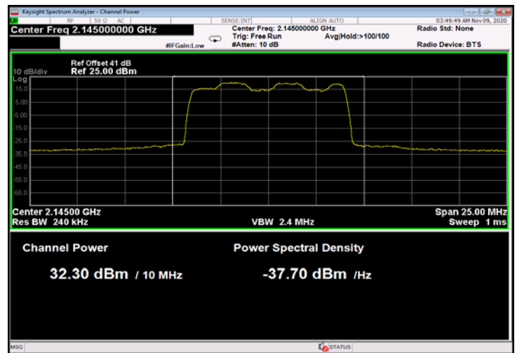
Figure 20: 16QAM 10MHz B.W.; 2145.0MHz, 60kHz
