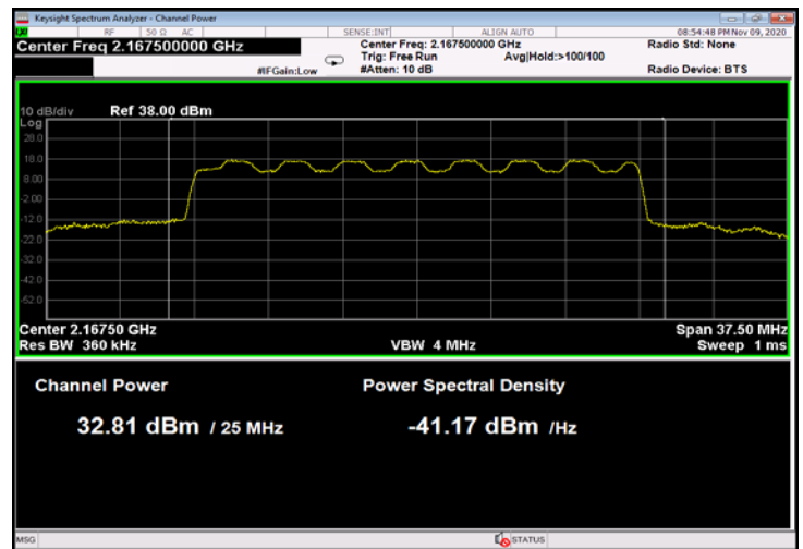
Figure 50: 16QAM 25MHz B.W.; 2167.5MHz, 60kHz
