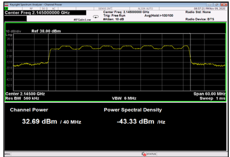
Figure 54: 16QAM 40MHz B.W.; 2145.0MHz, 15kHz
