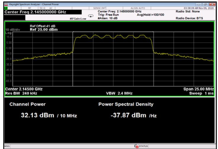
Figure 18: 16QAM 10MHz B.W.; 2145.0MHz, 15kHz
