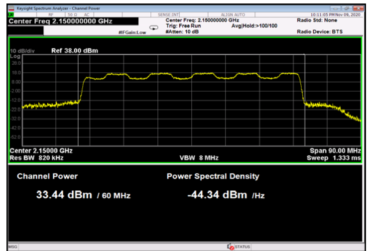
Figure 74: 16QAM 60MHz B.W.; 2150.0MHz, 60kHz
