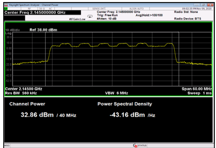
Figure 56: 16QAM 40MHz B.W.; 2145.0MHz, 60kHz
