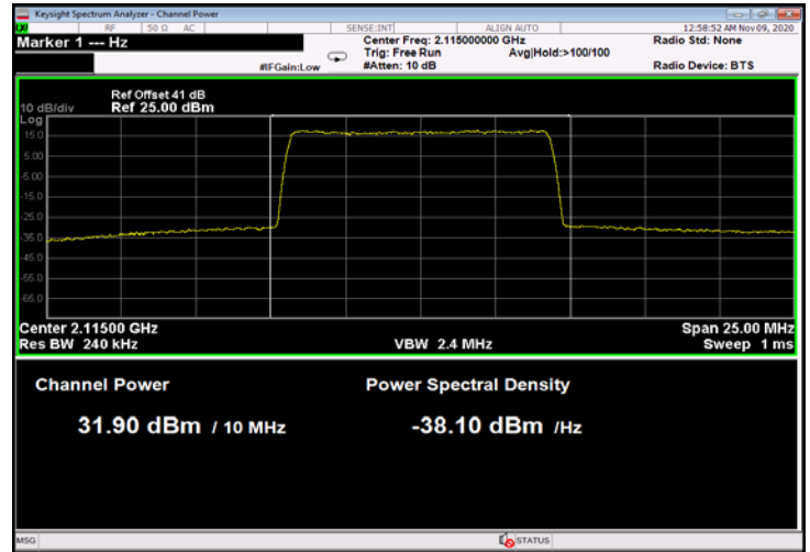
Figure 82: 64QAM 10MHz B.W.; 2115.0MHz, 30kHz
