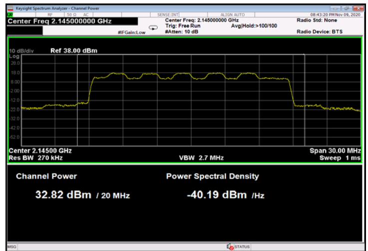
Figure 38: 16QAM 20MHz B.W.; 2145.0MHz, 60kHz
