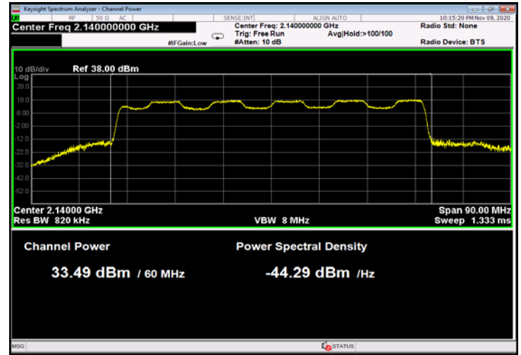
Figure 70: 16QAM 60MHz B.W.; 2140.0MHz, 60kHz
