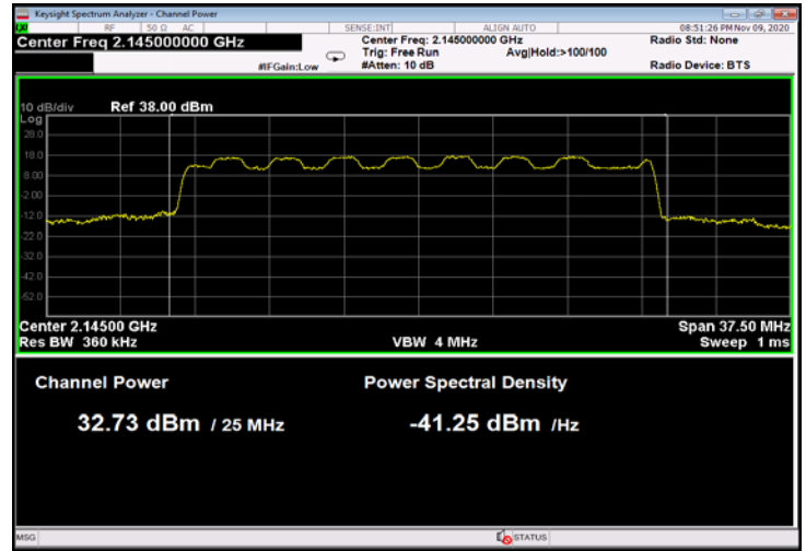
Figure 46: 16QAM 25MHz B.W.; 2145.0MHz, 30kHz
