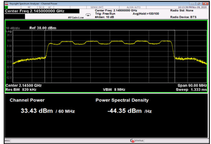
Figure 72: 16QAM 60MHz B.W.; 2145.0MHz, 60kHz
