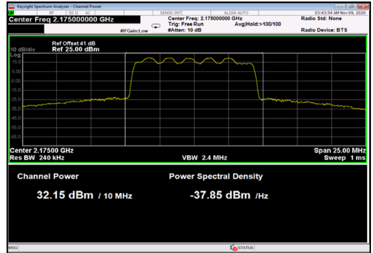
Figure 22: 16QAM 10MHz B.W.; 2175.0MHz, 30kHz
