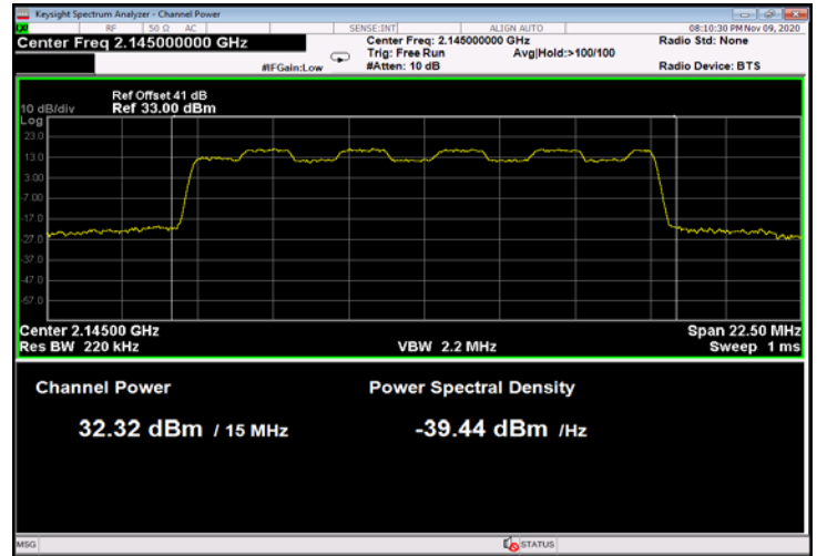
Figure 28: 16QAM 15MHz B.W.; 2145.0MHz, 30kHz
