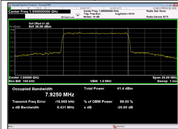
Figure 749: QPSK 10MHz B.W.; 1990.0MHz, 60kHz - Output
