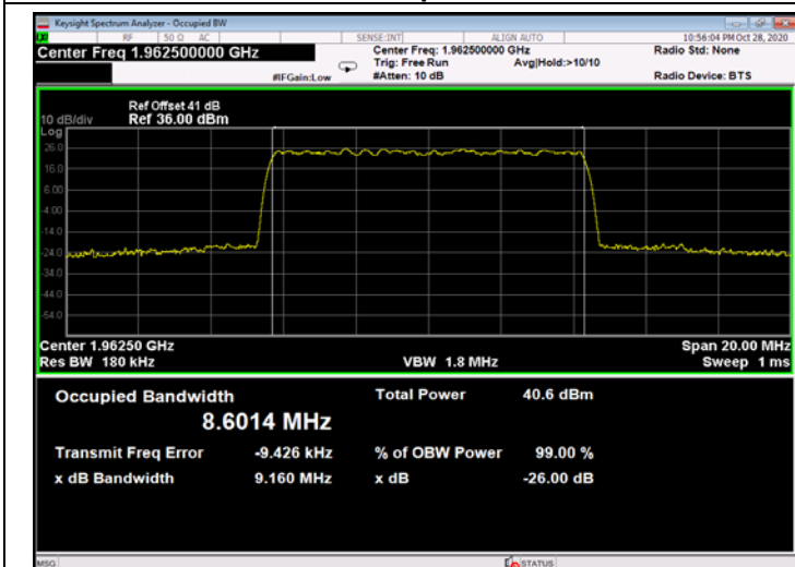
Figure 745: QPSK 10MHz B.W.; 1962.5MHz, 30kHz - Output
