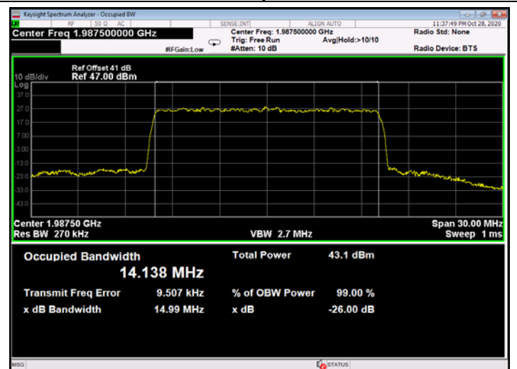
Figure 756: QPSK 15MHz B.W.; 1987.5MHz, 15kHz - Output
