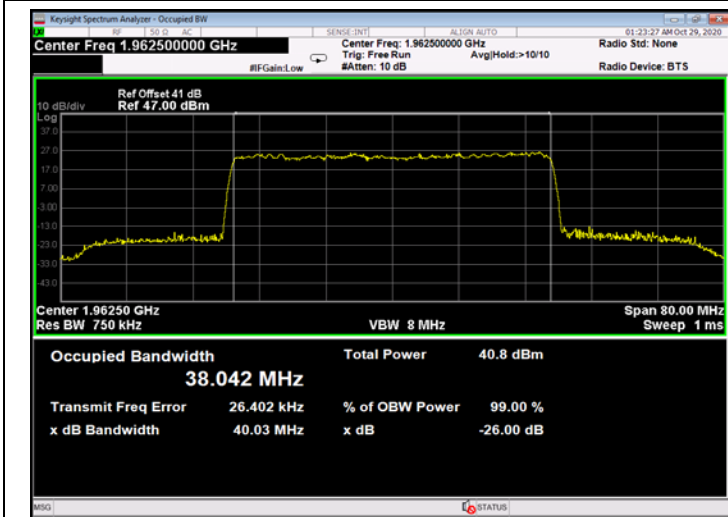
Figure 781: QPSK 40MHz B.W.; 1962.5MHz, 30kHz - Output
