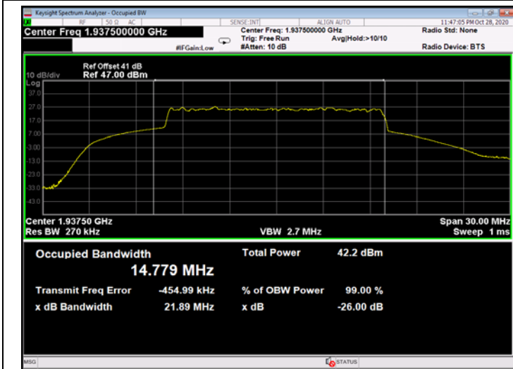
Figure 751: QPSK 15MHz B.W.; 1937.5MHz, 30kHz - Output
