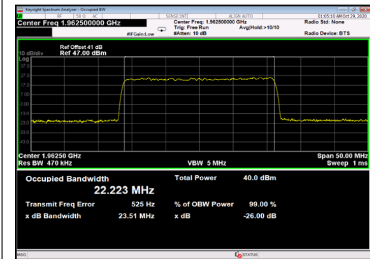
Figure 773: QPSK 25MHz B.W.; 1962.5MHz, 60kHz - Output
