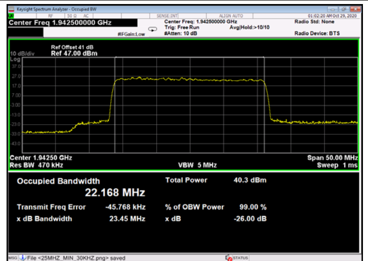
Figure 770: QPSK 25MHz B.W.; 1942.5MHz, 60kHz - Output
