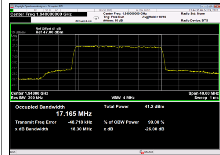
Figure 761: QPSK 20MHz B.W.; 1940.0MHz, 60kHz - Output
