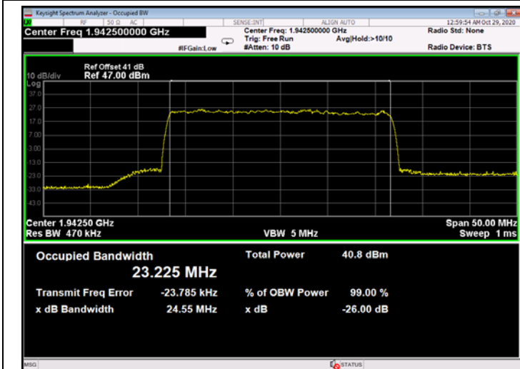
Figure 769: QPSK 25MHz B.W.; 1942.5MHz, 30kHz - Output
