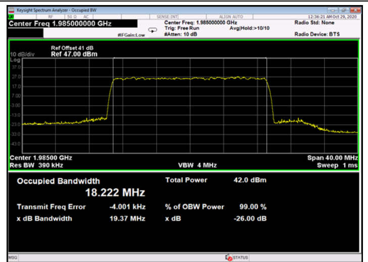
Figure 766: QPSK 20MHz B.W.; 1985.0MHz, 30kHz - Output
