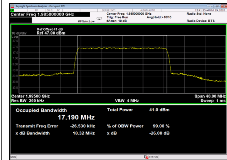
Figure 767: QPSK 20MHz B.W.; 1985.0MHz, 60kHz - Output
