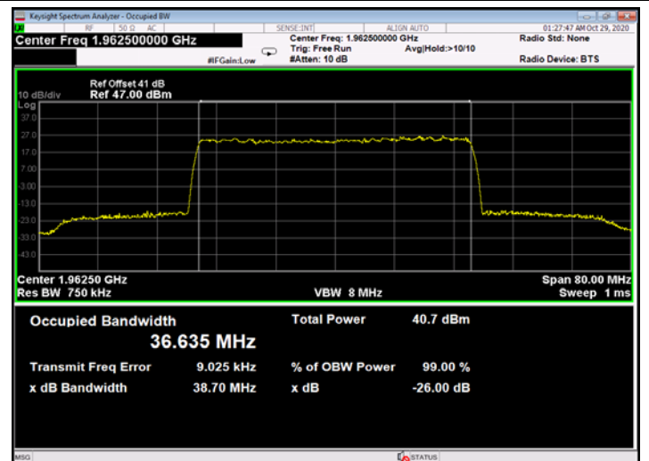
Figure 782: QPSK 40MHz B.W.; 1962.5MHz, 60kHz - Output
