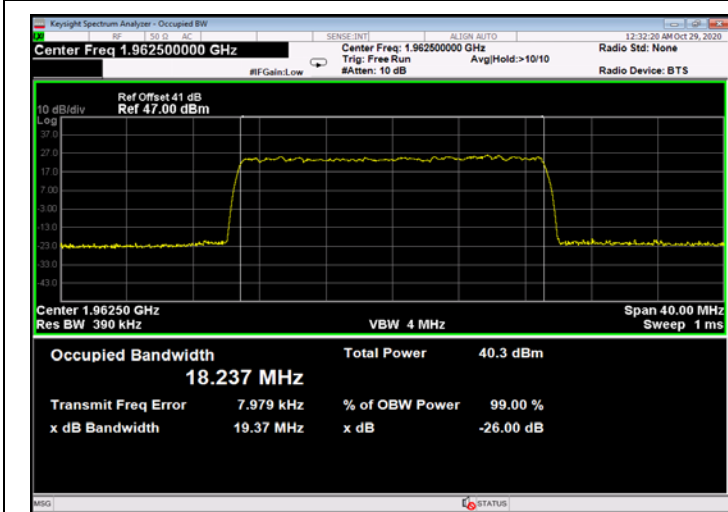
Figure 763: QPSK 20MHz B.W.; 1962.5MHz, 30kHz - Output
