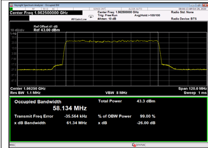
Figure 665: 64QAM 60MHz B.W.; 1962.5MHz, 30kHz - Output
