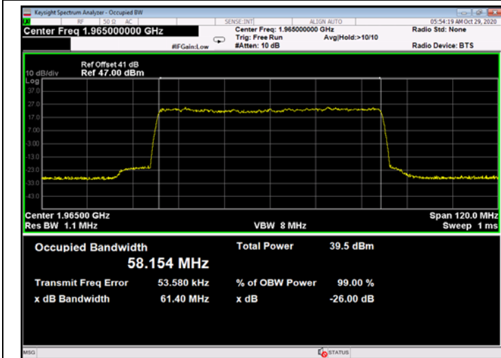
Figure 733: 256QAM 60MHz B.W.; 1965.0MHz, 30kHz - Output
