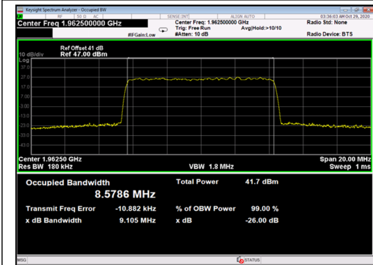
Figure 679: 256QAM 10MHz B.W.; 1962.5MHz, 30kHz - Output
