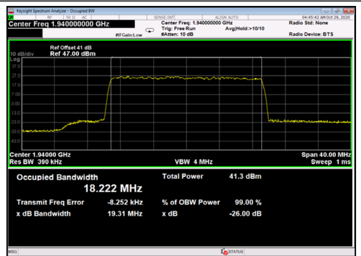
Figure 694: 256QAM 20MHz B.W.; 1940.0MHz, 30kHz - Output
