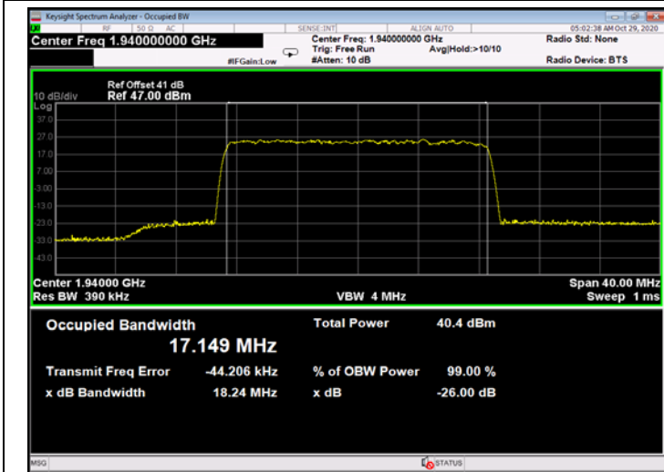
Figure 695: 256QAM 20MHz B.W.; 1940.0MHz, 60kHz - Output
