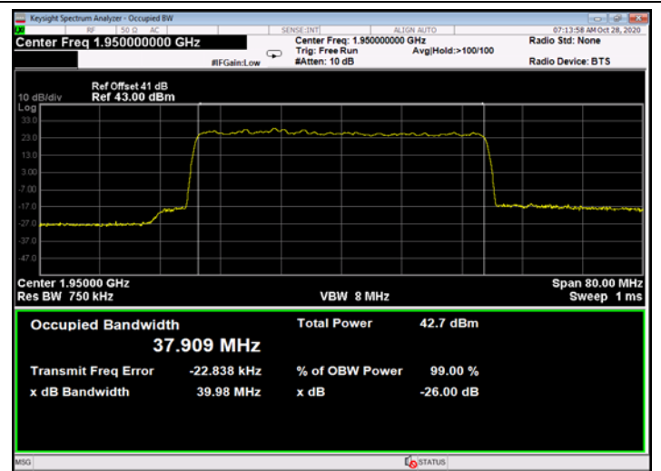
Figure 646: 64QAM 40MHz B.W.; 1950.0MHz, 30kHz - Output
