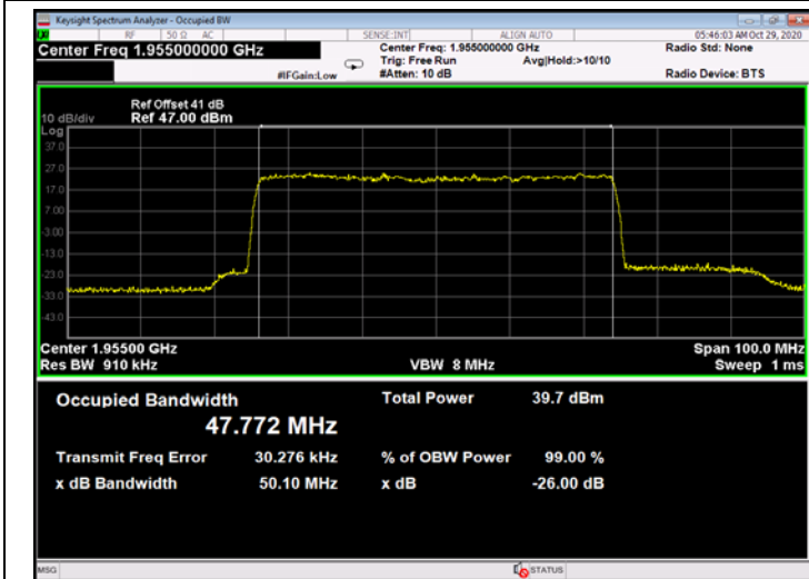
Figure 721: 256QAM 50MHz B.W.; 1955.0MHz, 30kHz - Output
