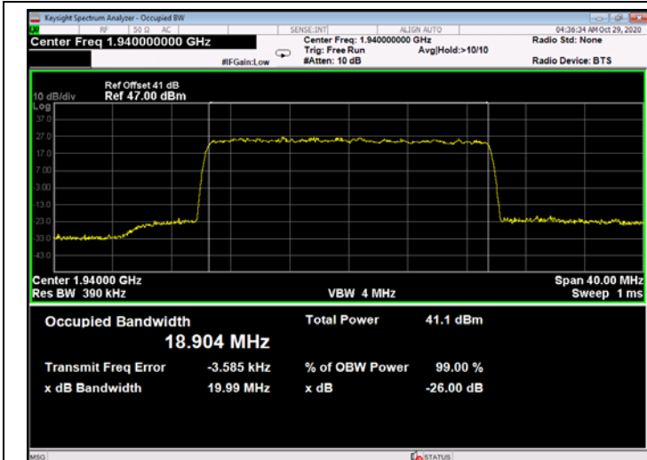
Figure 693: 256QAM 20MHz B.W.; 1940.0MHz, 15kHz - Output
