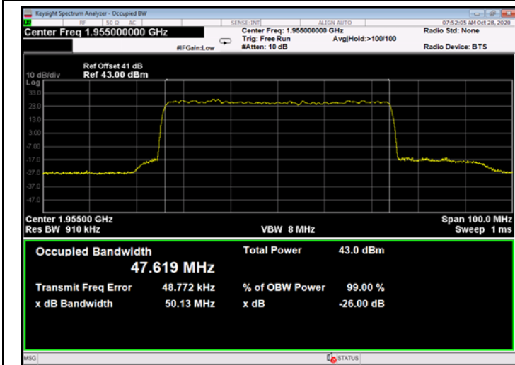
Figure 655: 64QAM 50MHz B.W.; 1955.0MHz, 30kHz - Output
