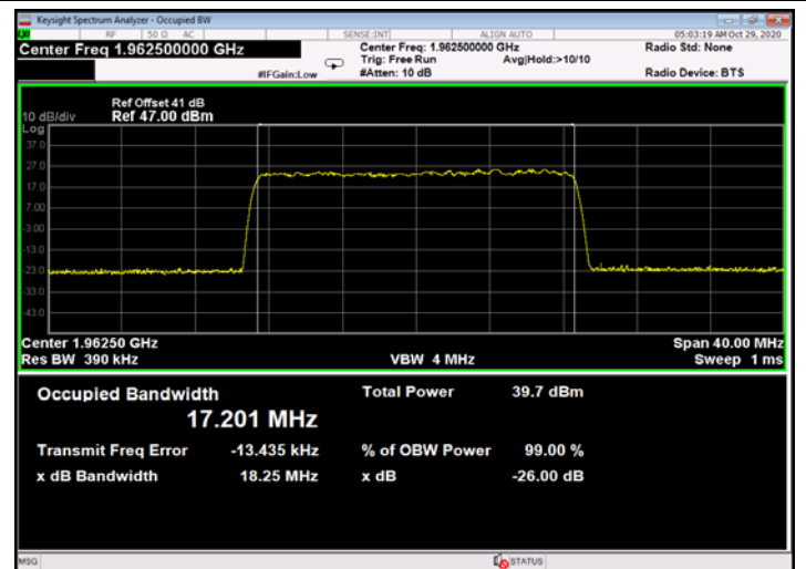
Figure 698: 256QAM 20MHz B.W.; 1962.5MHz, 60kHz - Output
