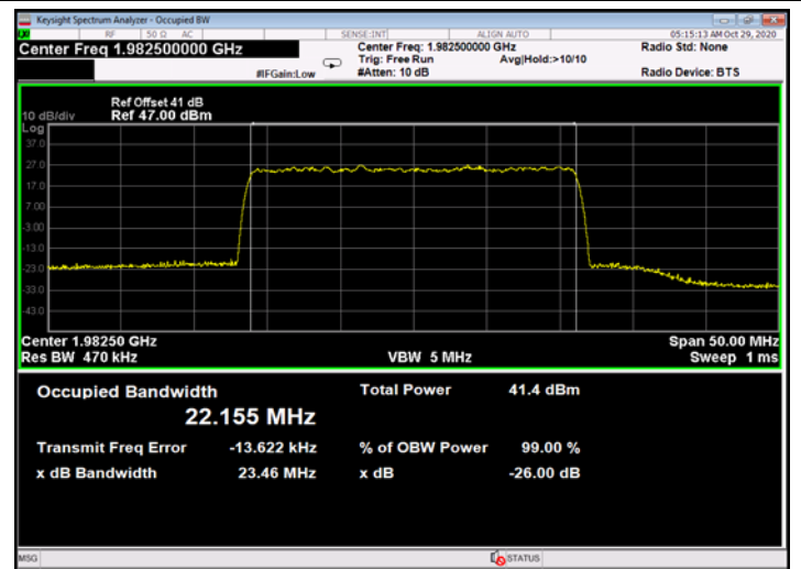
Figure 710: 256QAM 25MHz B.W.; 1982.5MHz, 60kHz - Output
