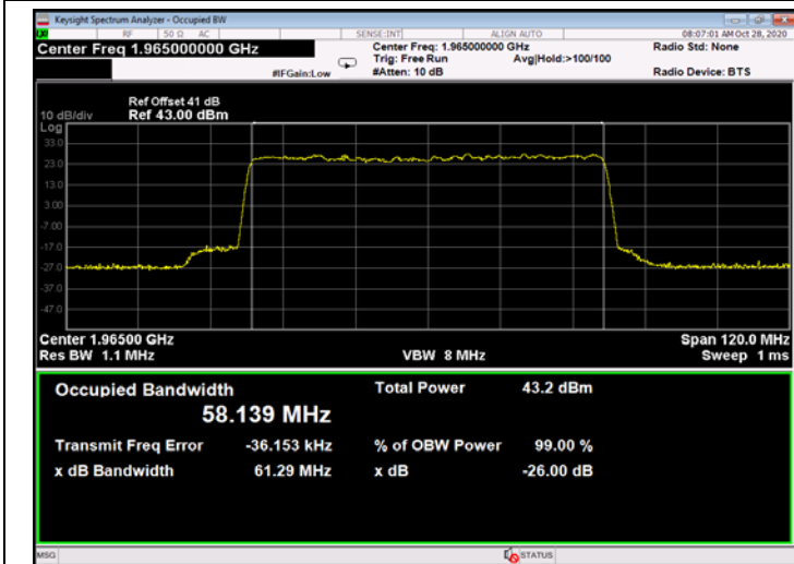
Figure 667: 64QAM 60MHz B.W.; 1965.0MHz, 30kHz - Output
