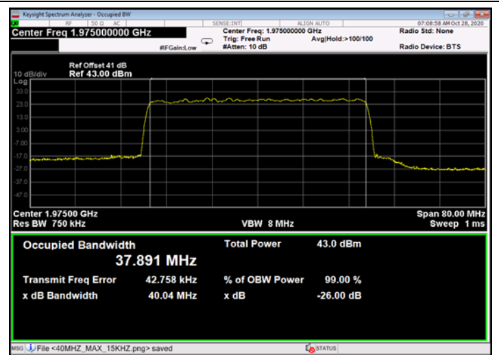
Figure 652: 64QAM 40MHz B.W.; 1975.0MHz, 30kHz - Output
