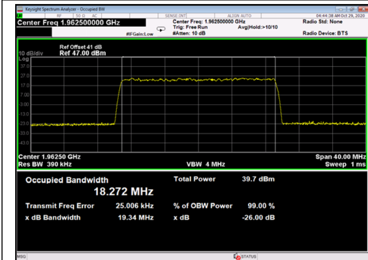
Figure 697: 256QAM 20MHz B.W.; 1962.5MHz, 30kHz - Output
