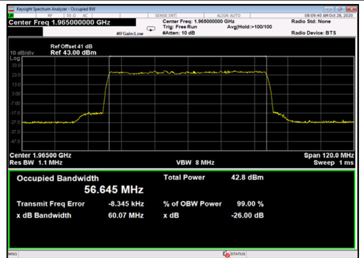
Figure 668: 64QAM 60MHz B.W.; 1965.0MHz, 60kHz - Output
