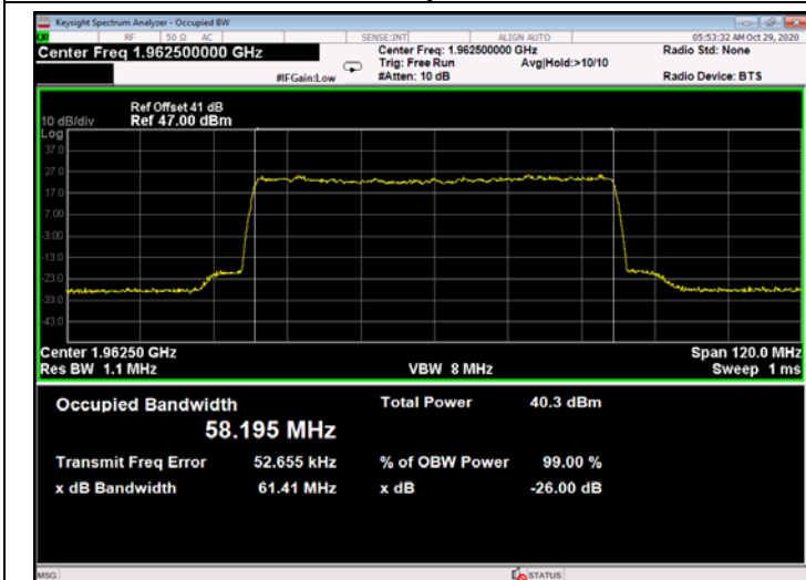
Figure 731: 256QAM 60MHz B.W.; 1962.5MHz, 30kHz - Output
