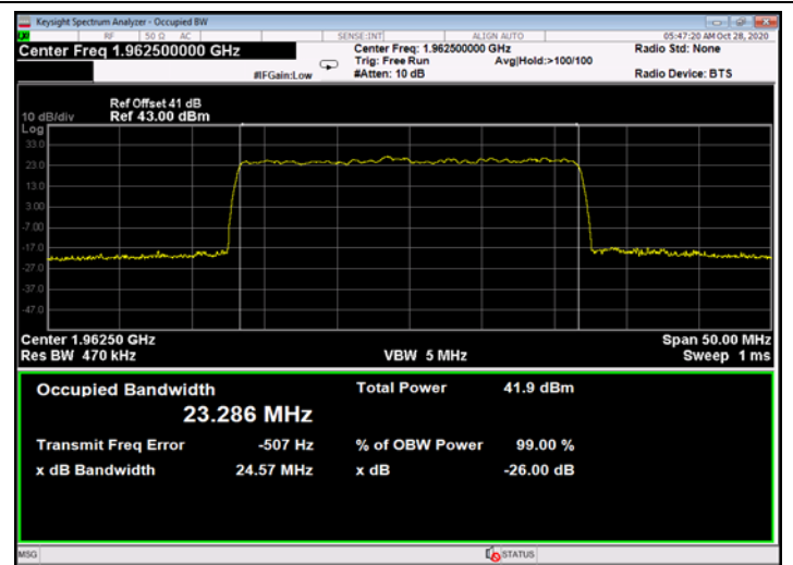
Figure 640: 64QAM 25MHz B.W.; 1962.5MHz, 30kHz - Output
