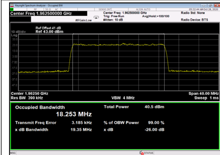
Figure 631: 64QAM 20MHz B.W.; 1962.5MHz, 30kHz - Output
