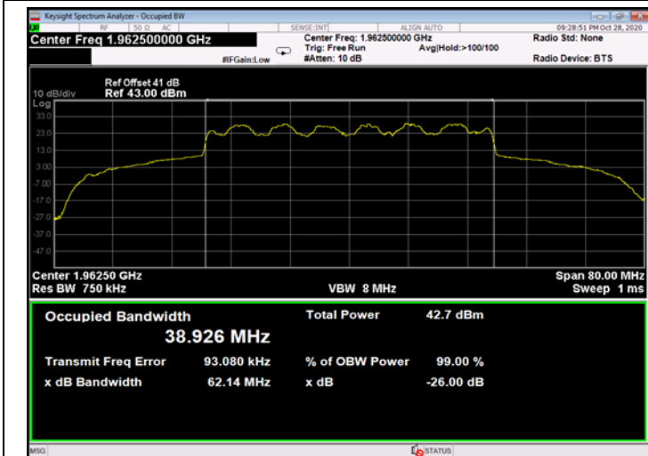
Figure 583: 16QAM 40MHz B.W.; 1962.5MHz, 30kHz - Output
