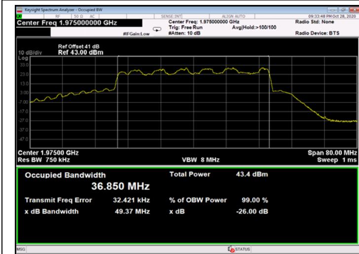
Figure 587: 16QAM 40MHz B.W.; 1975.0MHz, 60kHz - Output
