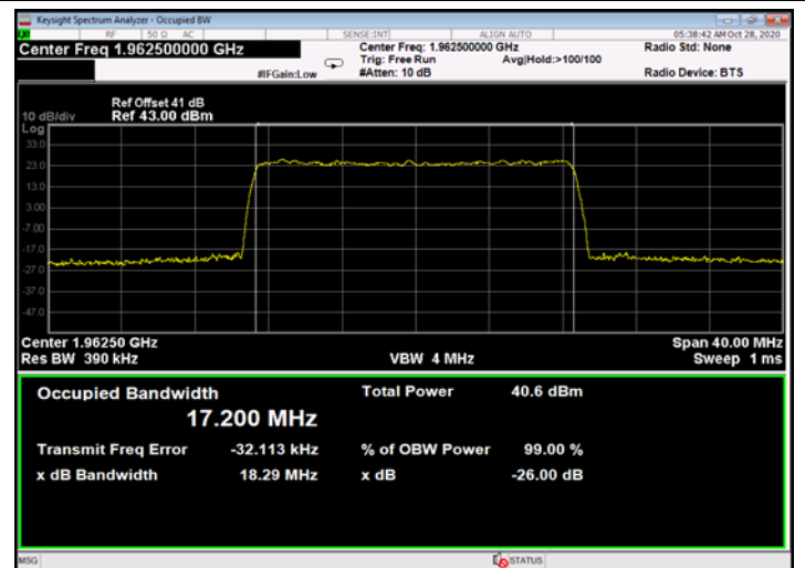
Figure 632: 64QAM 20MHz B.W.; 1962.5MHz, 60kHz - Output
