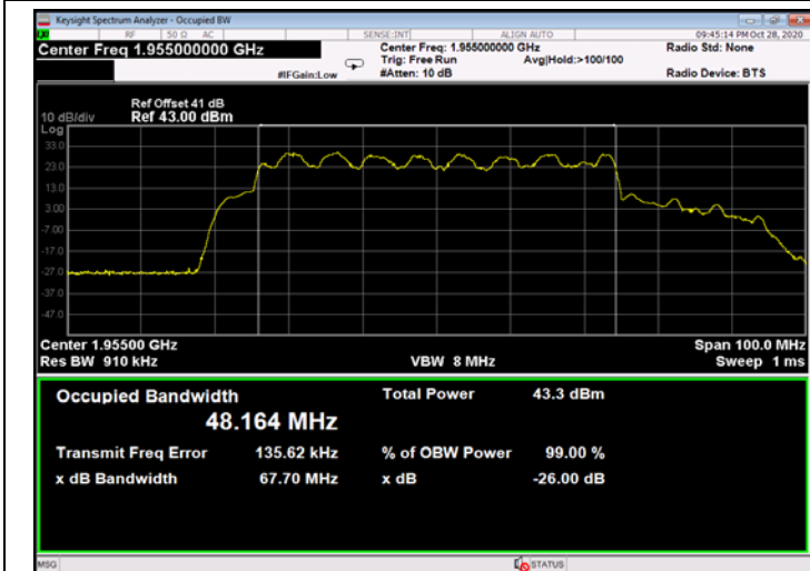
Figure 589: 16QAM 50MHz B.W.; 1955.0MHz, 30kHz - Output
