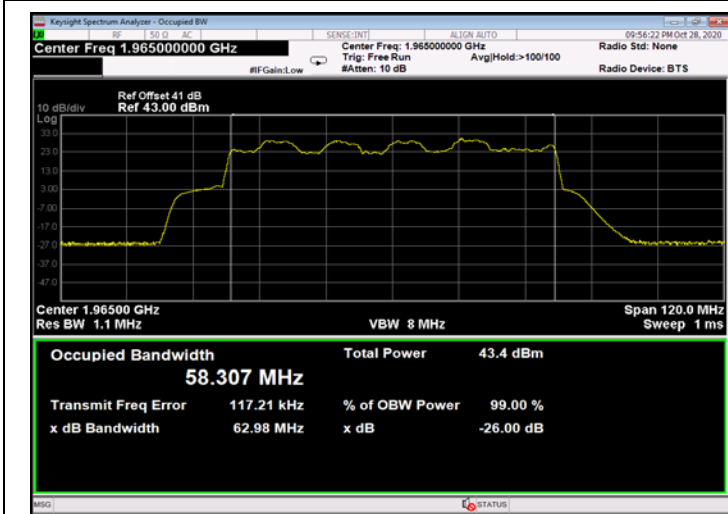
Figure 601: 16QAM 60MHz B.W.; 1965.0MHz, 30kHz - Output
