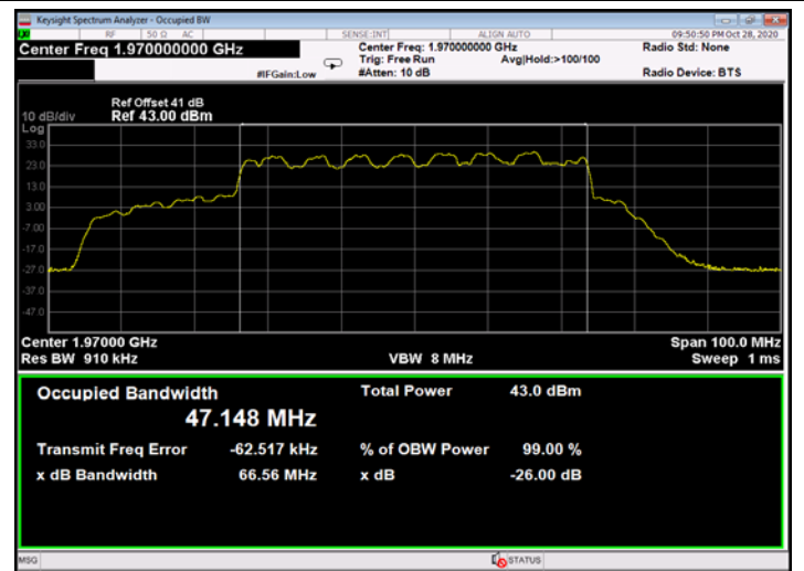
Figure 596: 16QAM 50MHz B.W.; 1970.0MHz, 60kHz - Output
