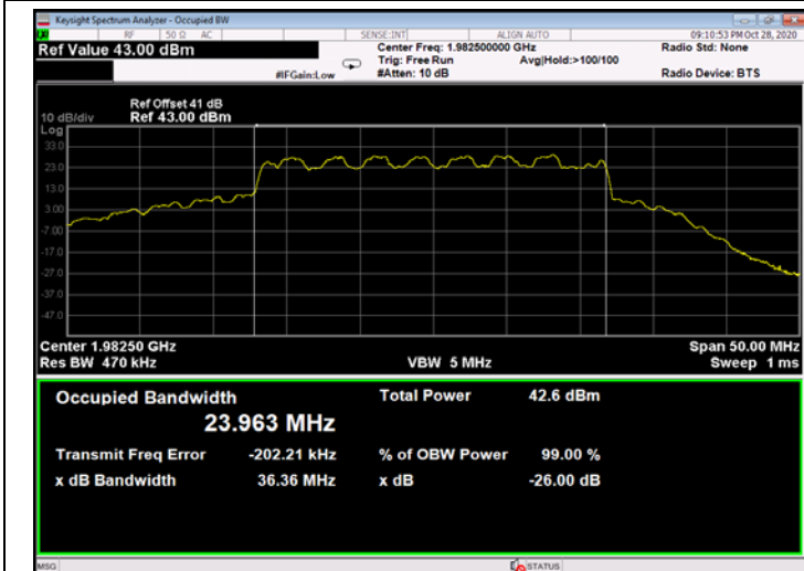
Figure 577: 16QAM 25MHz B.W.; 1982.5MHz, 30kHz - Output
