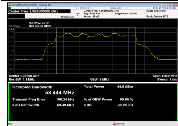
Figure 599: 16QAM 60MHz B.W.; 1962.5MHz, 30kHz - Output
