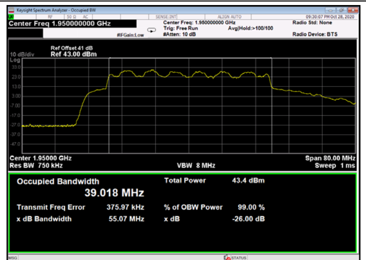
Figure 580: 16QAM 40MHz B.W.; 1950.0MHz, 30kHz - Output
