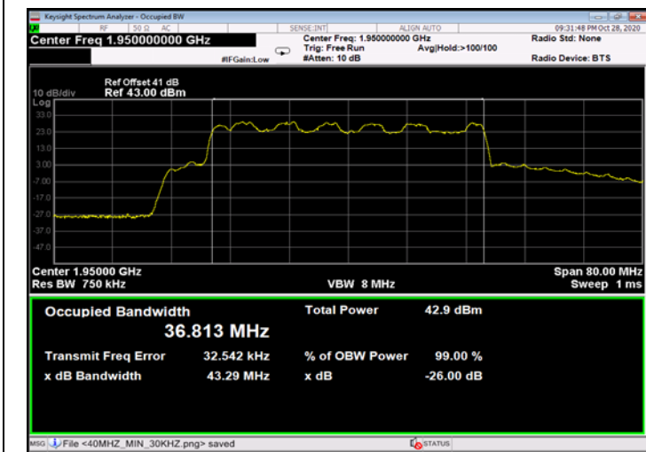
Figure 581: 16QAM 40MHz B.W.; 1950.0MHz, 60kHz - Output
