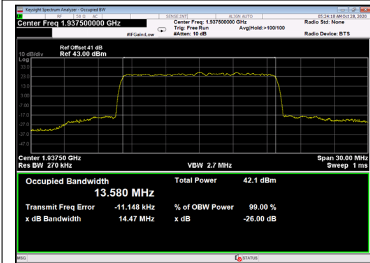
Figure 619: 64QAM 15MHz B.W.; 1937.5MHz, 30kHz - Output
