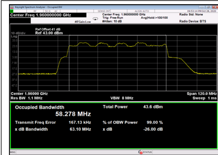
Figure 597: 16QAM 60MHz B.W.; 1960.0MHz, 30kHz - Output
