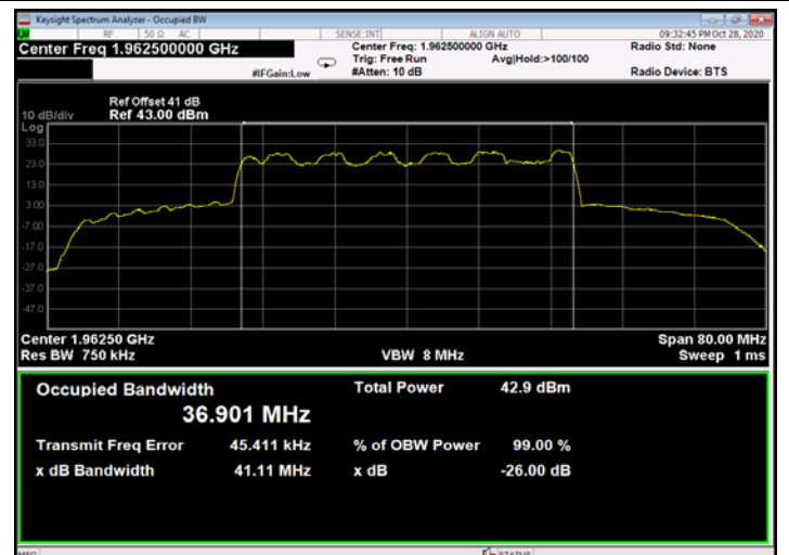
Figure 584: 16QAM 40MHz B.W.; 1962.5MHz, 60kHz - Output
