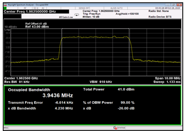
Figure 606: 64QAM 5MHz B.W.; 1962.5MHz, 30kHz - Output
