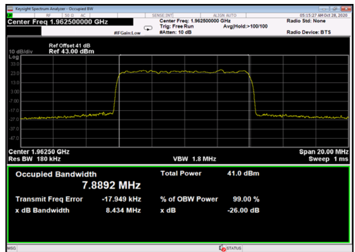
Figure 614: 64QAM 10MHz B.W.; 1962.5MHz, 60kHz - Output
