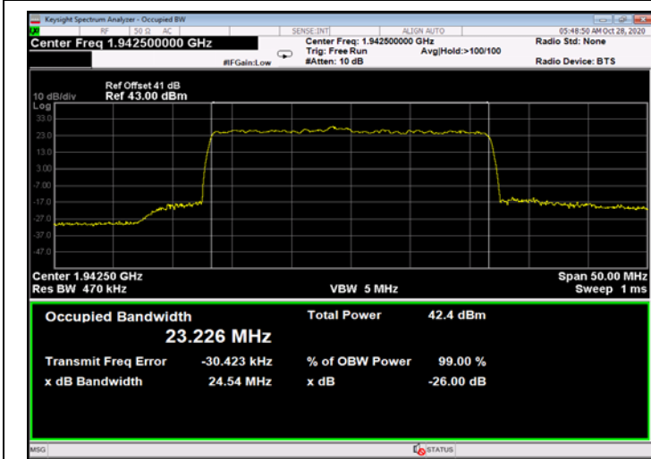
Figure 637: 64QAM 25MHz B.W.; 1942.5MHz, 30kHz - Output
