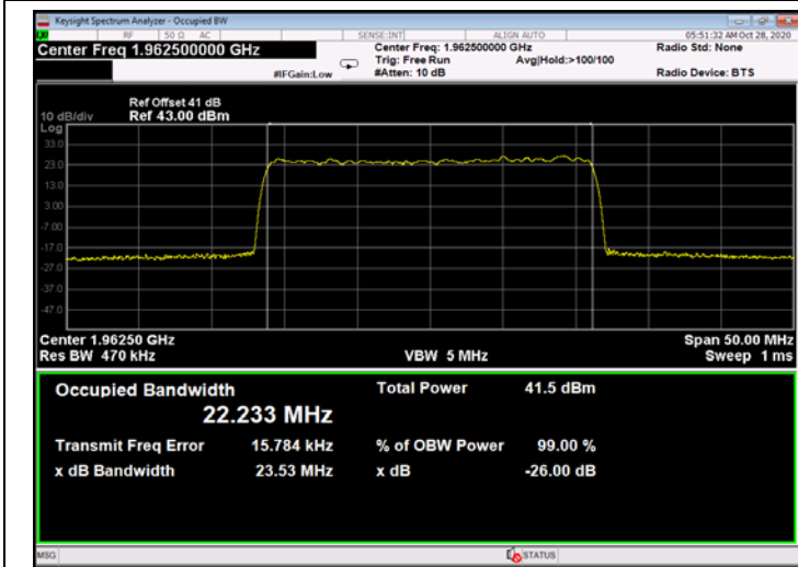
Figure 641: 64QAM 25MHz B.W.; 1962.5MHz, 60kHz - Output
