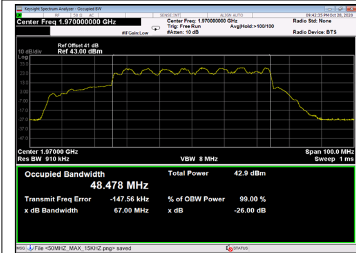
Figure 595: 16QAM 50MHz B.W.; 1970.0MHz, 30kHz - Output
