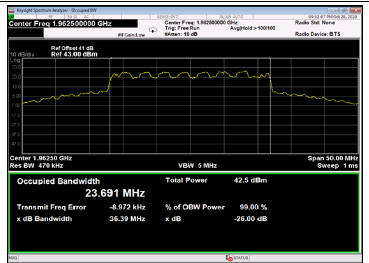
Figure 574: 16QAM 25MHz B.W.; 1962.5MHz, 30kHz - Output
