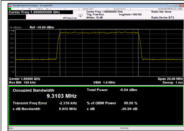
Figure 483: QPSK 10MHz B.W.; 1990.0MHz, 15kHz - Input
