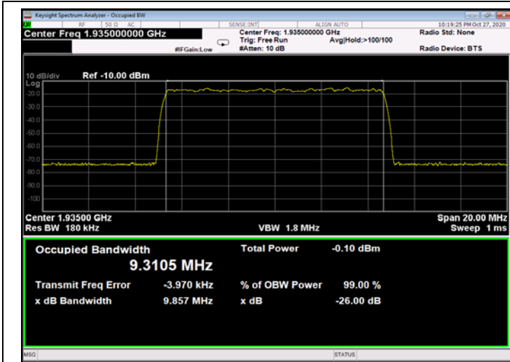
Figure 477: QPSK 10MHz B.W.; 1935.00MHz, 15kHz - Input
