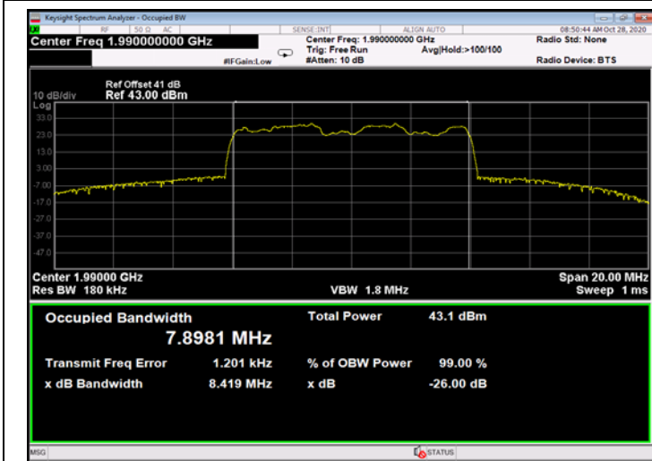
Figure 551: 16QAM 10MHz B.W.; 1990.0MHz, 60kHz - Output
