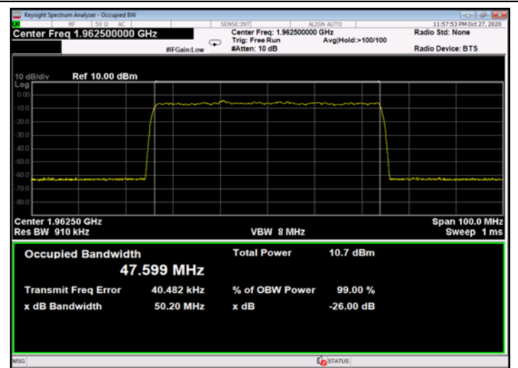
Figure 526: QPSK 50MHz B.W.; 1962.5MHz, 30kHz - Input
