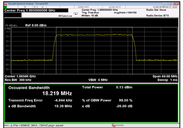
Figure 502: QPSK 20MHz B.W.; 1985.0MHz, 30kHz - Input
