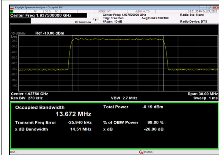
Figure 487: QPSK 15MHz B.W.; 1937.5MHz, 30kHz - Input
