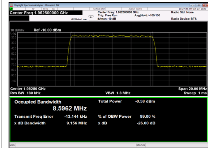
Figure 481: QPSK 10MHz B.W.; 1962.5MHz, 30kHz - Input
