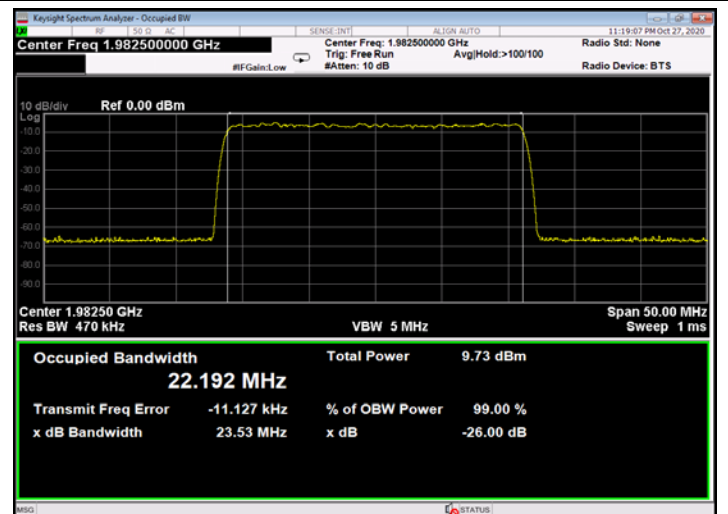
Figure 512: QPSK 25MHz B.W.; 1982.5MHz, 60kHz - Input
