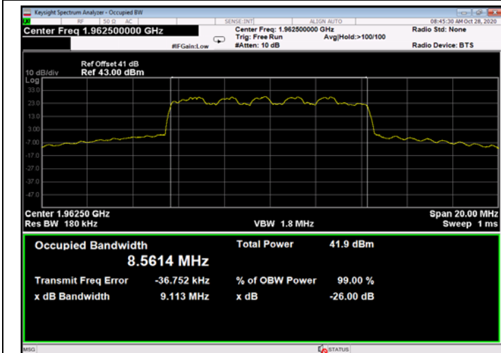
Figure 547: 16QAM 10MHz B.W.; 1962.5MHz, 30kHz - Output
