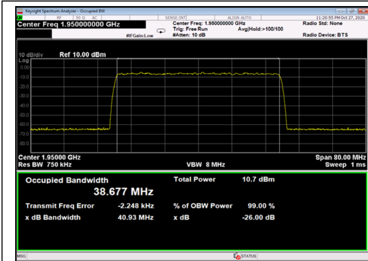
Figure 513: QPSK 40MHz B.W.; 1950.0MHz, 15kHz - Input
