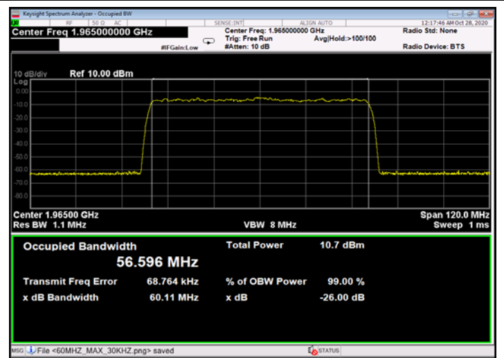
Figure 536: QPSK 60MHz B.W.; 1965.0MHz, 60kHz- Input
