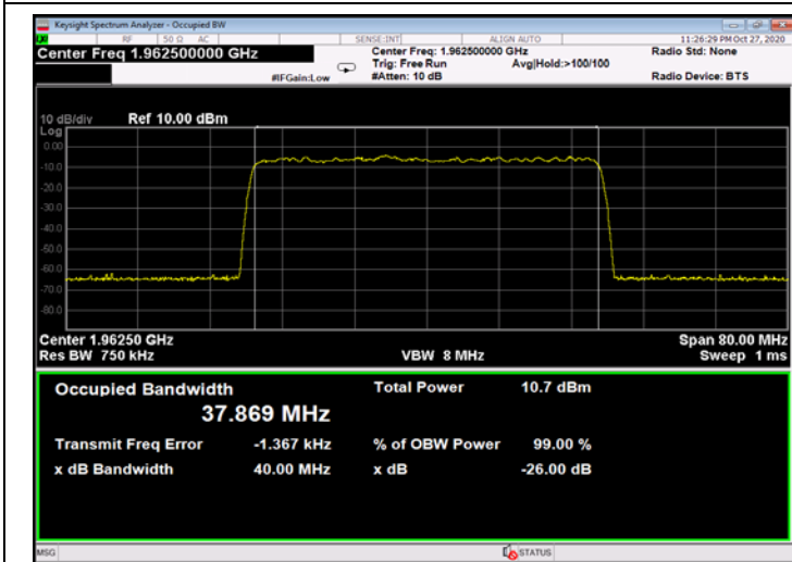
Figure 517: QPSK 40MHz B.W.; 1962.5MHz, 30kHz - Input
