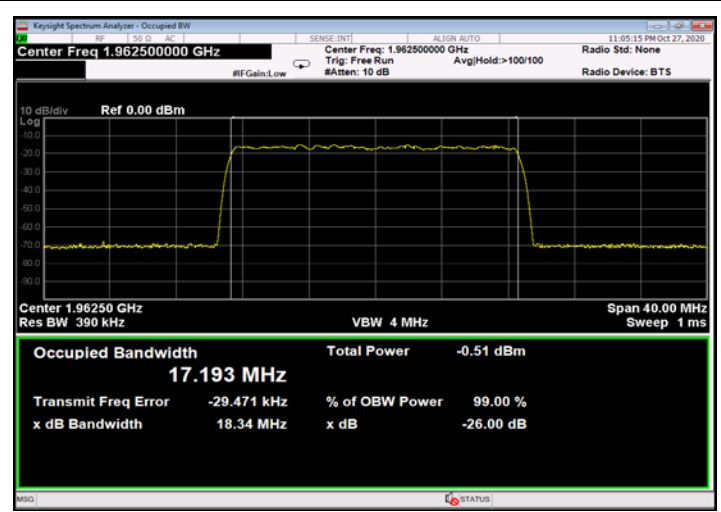
Figure 500: QPSK 20MHz B.W.; 1962.5MHz, 60kHz - Input
