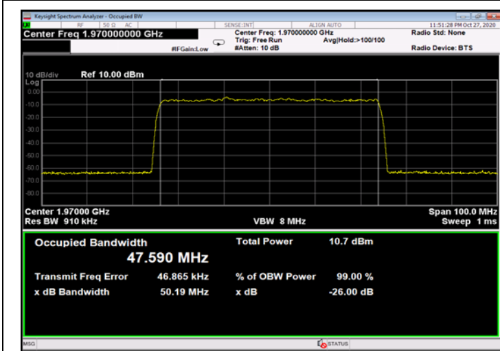
Figure 529: QPSK 50MHz B.W.; 1970.0MHz, 30kHz - Input
