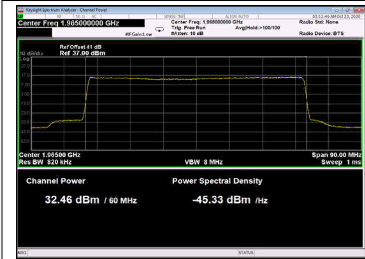
Figure 139: 64QAM 60MHz B.W.; 1965.0MHz, 30kHz
