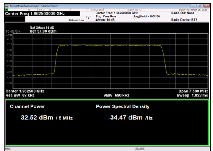
Figure 144: 256QAM 5MHz B.W.; 1962.5MHz, 30kHz
