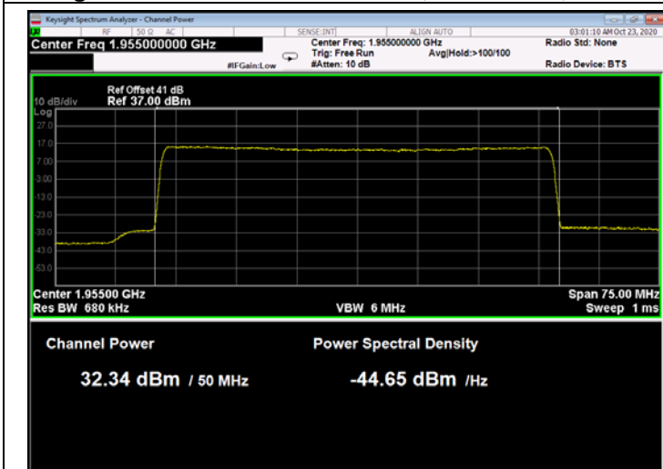
Figure 127: 64QAM 50MHz B.W.; 1955.0MHz, 30kHz
