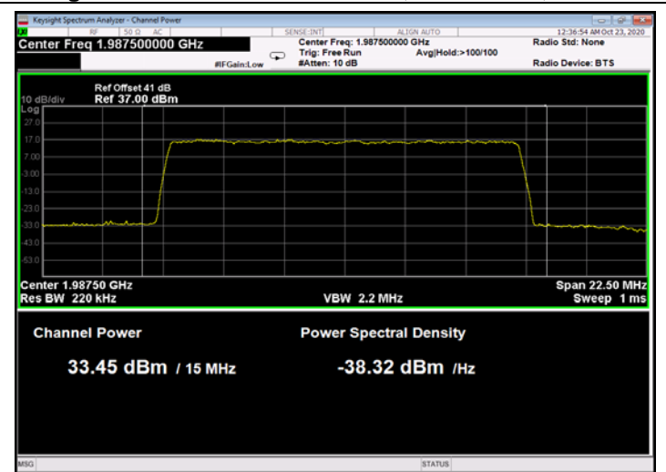
Figure 98: 64QAM 15MHz B.W.; 1987.5MHz, 60kHz
