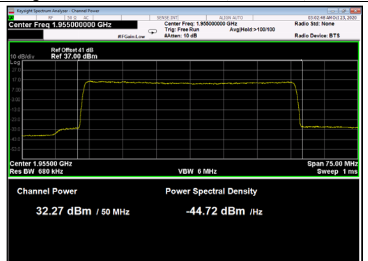
Figure 128: 64QAM 50MHz B.W.; 1955.0MHz, 60kHz
