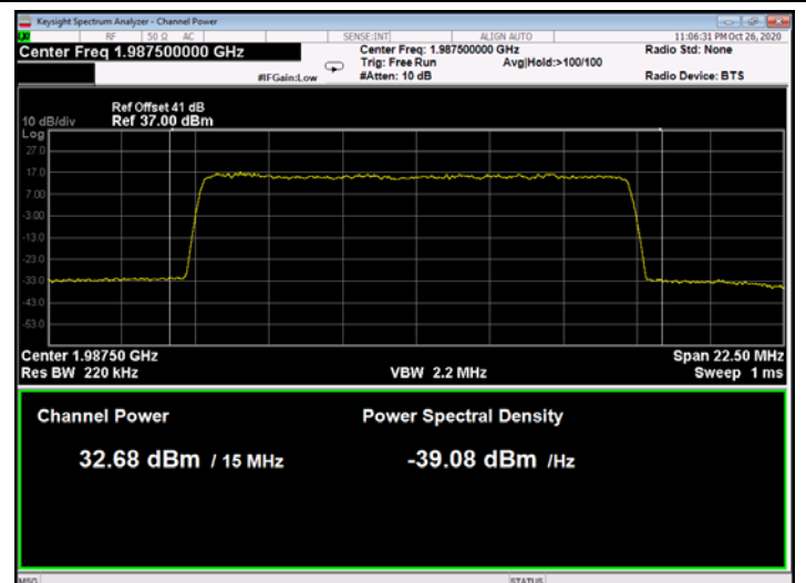
Figure 164: 256QAM 15MHz B.W.; 1987.5MHz, 60kHz
