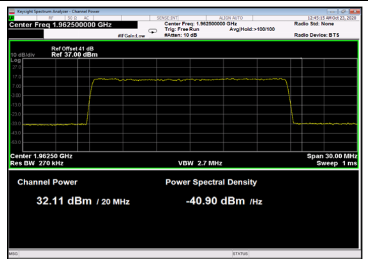
Figure 104: 64QAM 20MHz B.W.; 1962.5MHz, 60kHz
