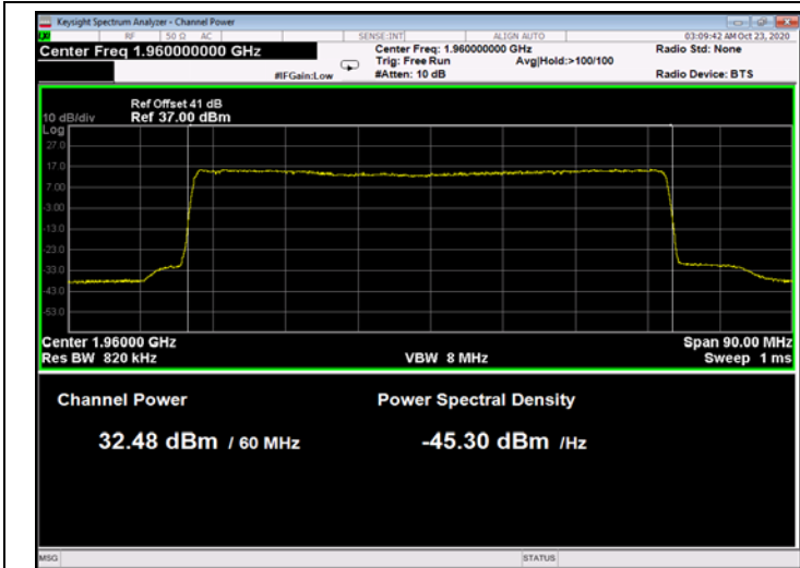
Figure 135: 64QAM 60MHz B.W.; 1960.0MHz, 30kHz
