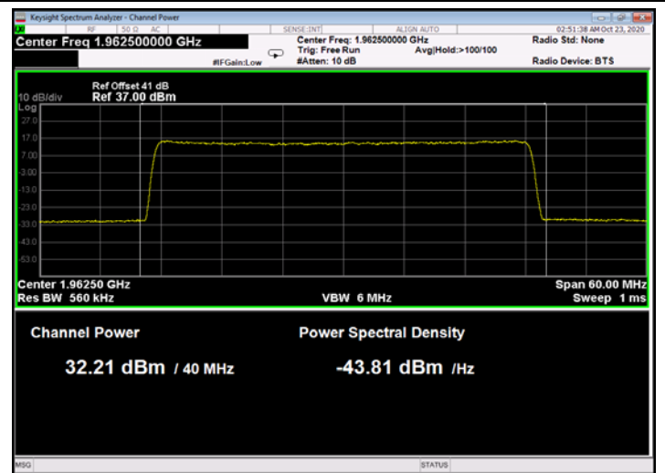
Figure 122: 64QAM 40MHz B.W.; 1962.5MHz, 60kHz
