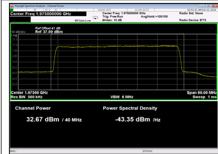
Figure 125: 64QAM 40MHz B.W.; 1975.0MHz, 60kHz
