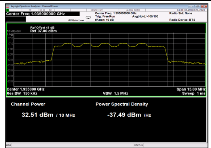
Figure 16: 16QAM 10MHz B.W.; 1935.0MHz, 30kHz
