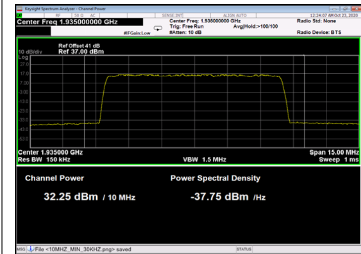
Figure 83: 64QAM 10MHz B.W.; 1935.0MHz, 60kHz
