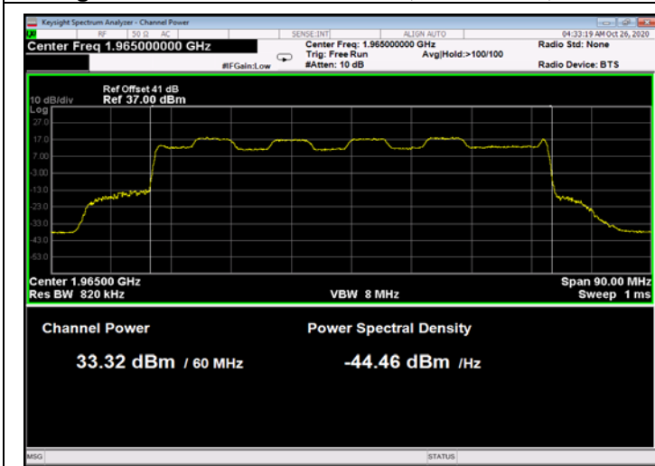
Figure 73: 16QAM 60MHz B.W.; 1965.0MHz, 30kHz
