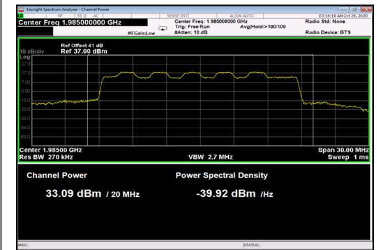
Figure 41: 16QAM 20MHz B.W.; 1985.0MHz, 60kHz
