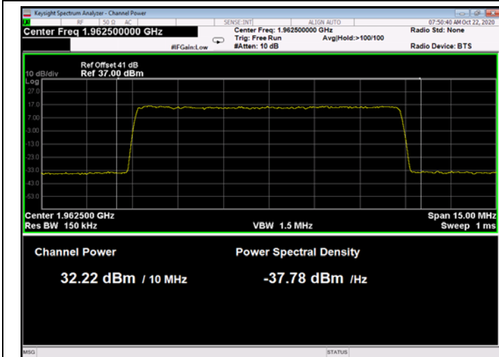
Figure 85: 64QAM 10MHz B.W.; 1962.5MHz, 30kHz
