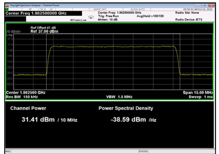
Figure 84: 64QAM 10MHz B.W.; 1962.5MHz, 15kHz
