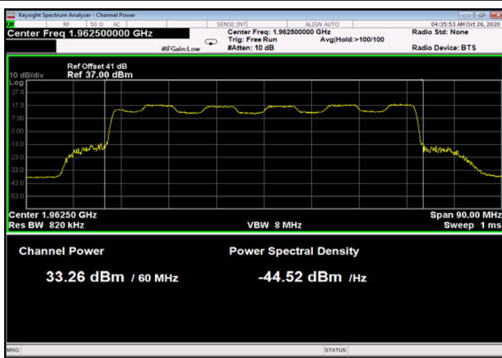
Figure 72: 16QAM 60MHz B.W.; 1962.5MHz, 60kHz
