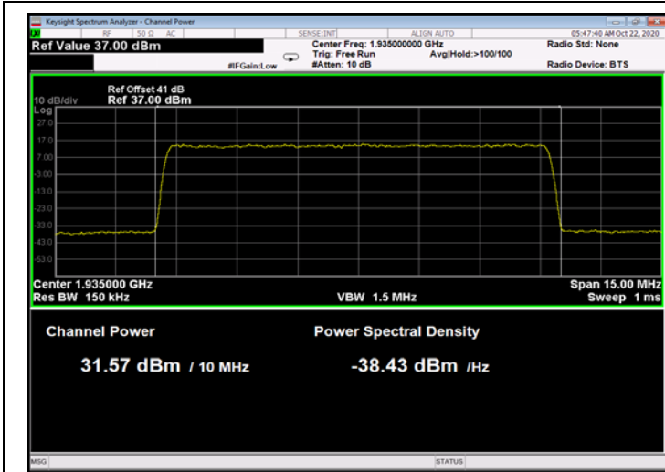
Figure 81: 64QAM 10MHz B.W.; 1935.00MHz, 15kHz
