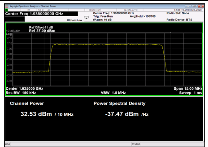
Figure 82: 64QAM 10MHz B.W.; 1935.0MHz, 30kHz
