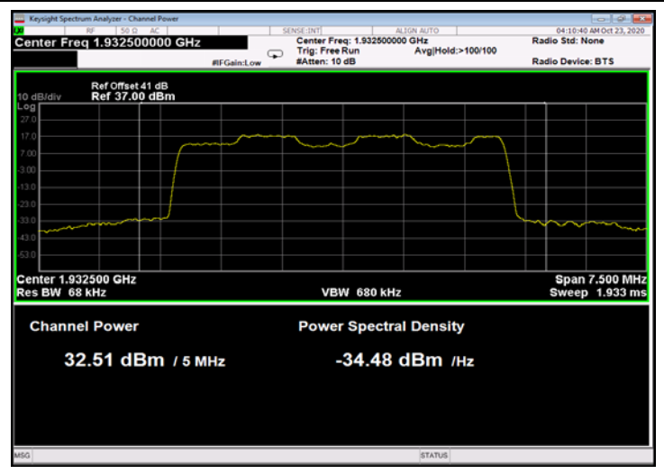
Figure 10: 16QAM 5MHz B.W.; 1932.5MHz, 30kHz
