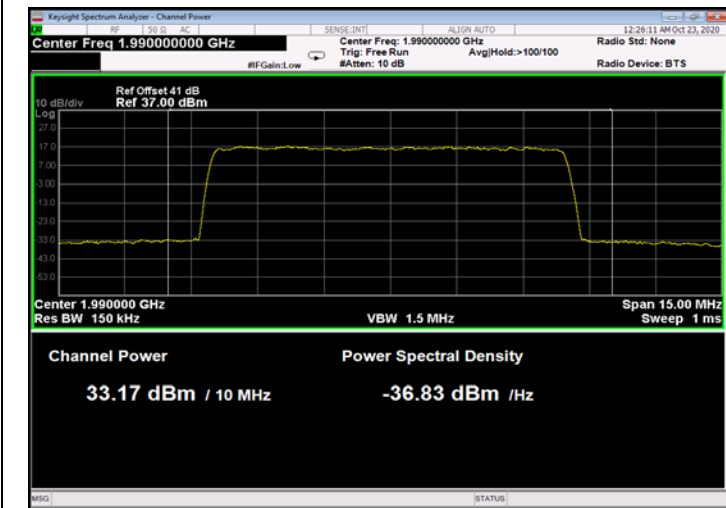
Figure 89: 64QAM 10MHz B.W.; 1990.0MHz, 60kHz
