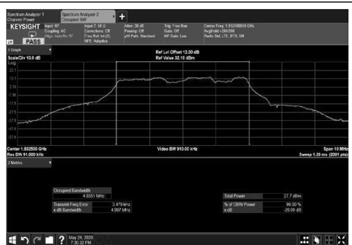
Figure 206: 16QAM 5MHz B.W.; 1932.5MHz, 30kHz Output
