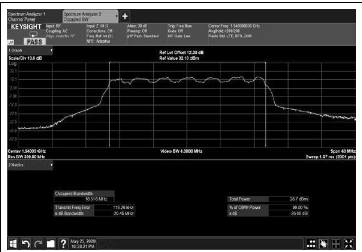
Figure 230: 16QAM 20MHz B.W.; 1940.0MHz, 30kHz Output
