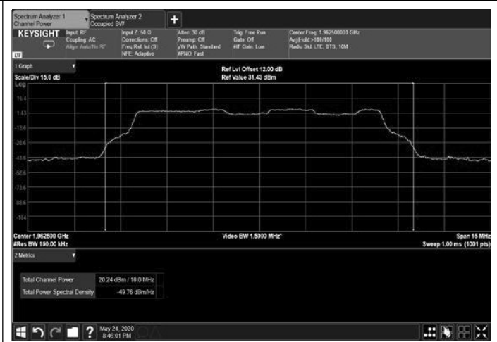
Figure 18: 16QAM 10MHz B.W.; 1962.5MHz, 60kHz
