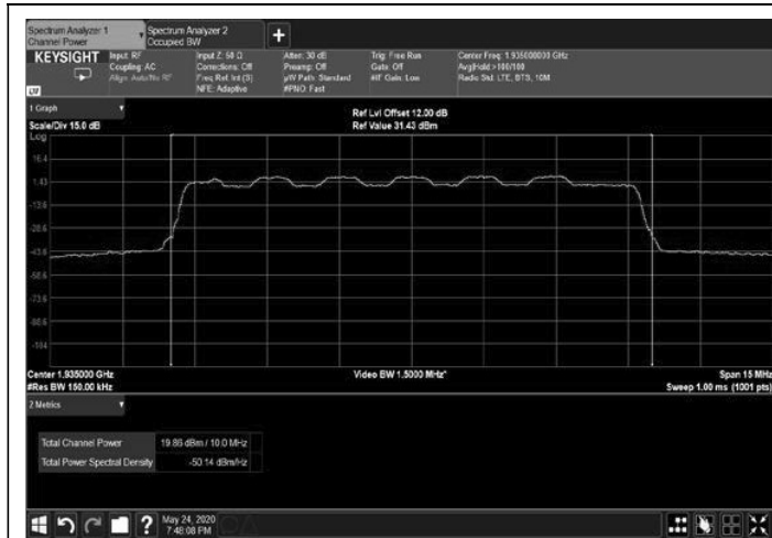
Figure 13: 16QAM 10MHz B.W.; 1935.0MHz, 15kHz
