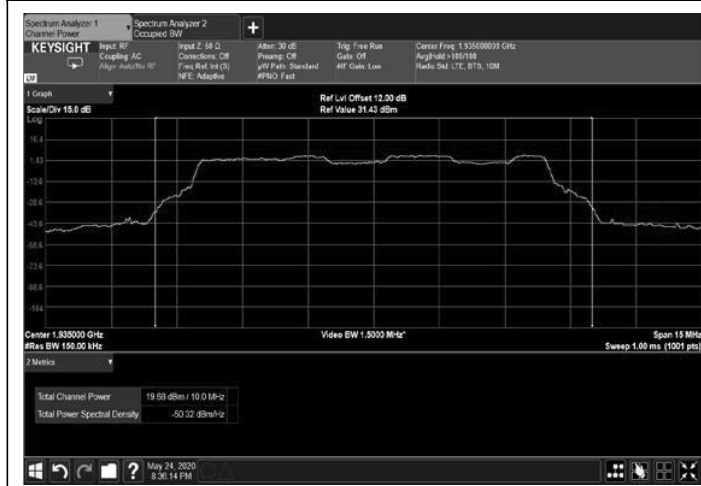
Figure 15: 16QAM 10MHz B.W.; 1935.0MHz, 60kHz
