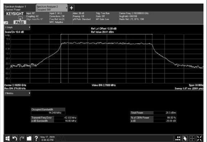
Figure 258: 64QAM 15MHz B.W.; 2192.5MHz, 15kHz Output
