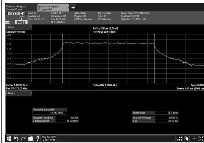
Figure 291: 256QAM 15MHz B.W.; 2192.5MHz, 15kHz Output
