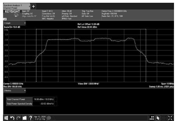
Figure 18: 16QAM 10MHz B.W.; 2155.0MHz, 60kHz
