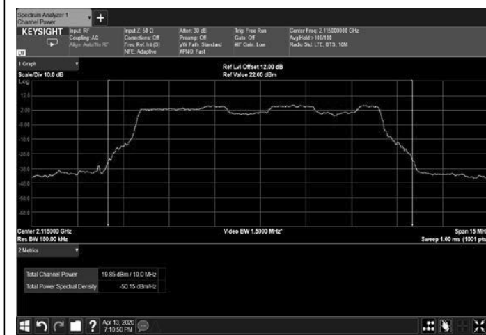
Figure 15: 16QAM 10MHz B.W.; 2115.0MHz, 60kHz
