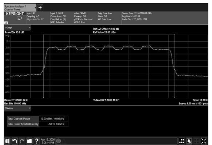
Figure 16: 16QAM 10MHz B.W.; 2155.0MHz, 15kHz
