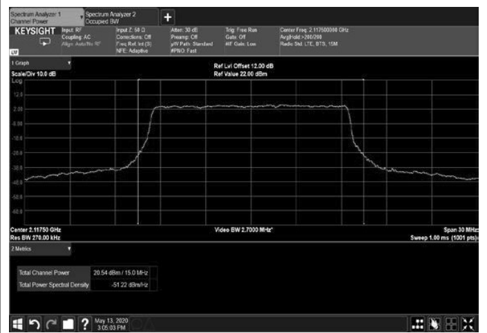
Figure 90: 256QAM 15MHz B.W.; 2117.5MHz, 60kHz
