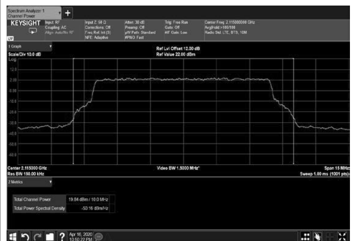
Figure 48: 64QAM 10MHz B.W.; 2115.0MHz, 60kHz
