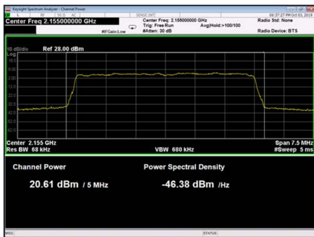
Figure 26 5MHz BW, 2155MHz
