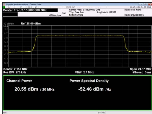
Figure 59 20MHz BW, 2155MHz
