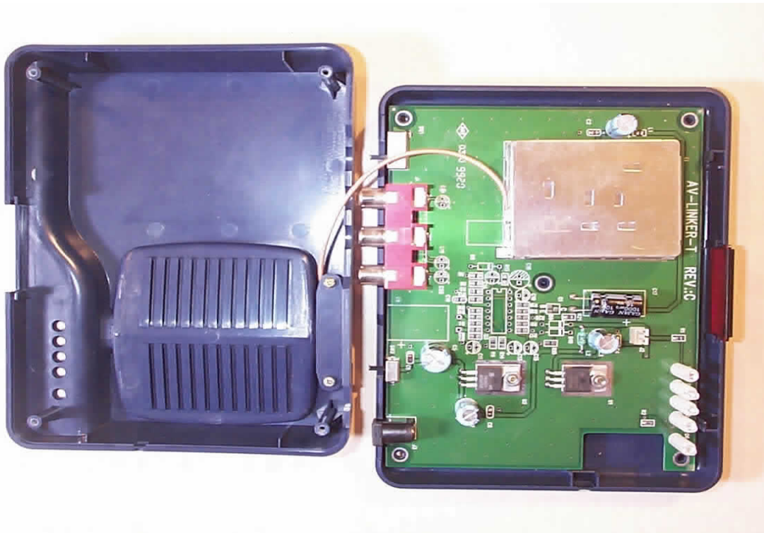
(4) EUT Photo
