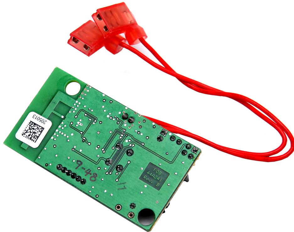
HH PCB BOTTOM
