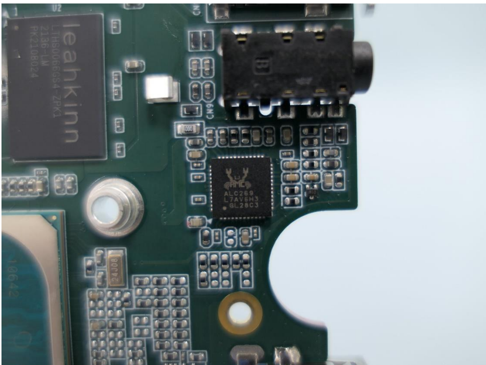
(46) EUT Photo
