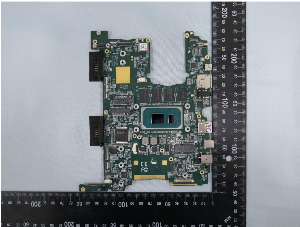
(40) EUT Photo
