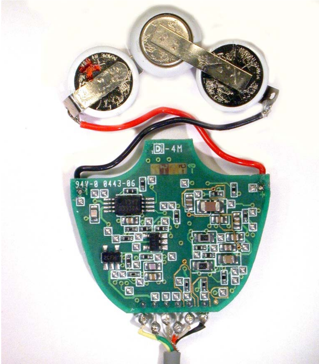
PCB BOTTOM 2
