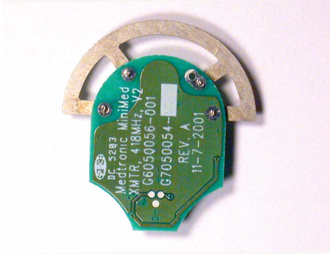
PCB TOP 2
