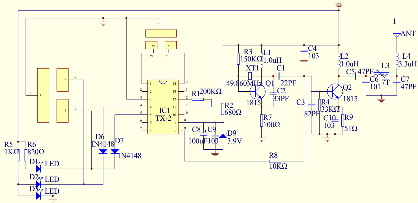
17039 49MHz发射电路图
