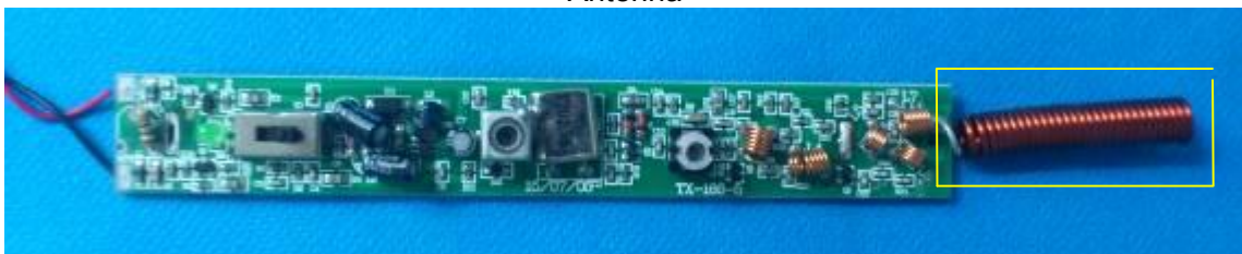
Antenna
