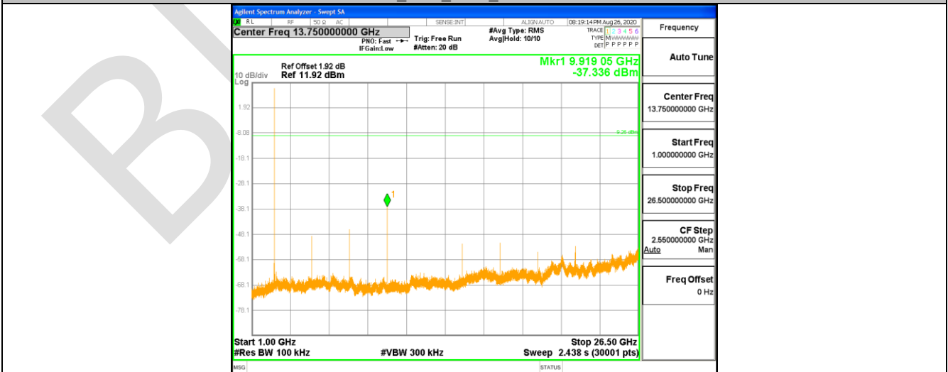
2.4G_Ant1_2480_1000~26500
