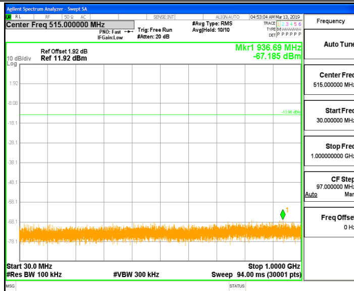
TX_Ant1_2442_30~1000
