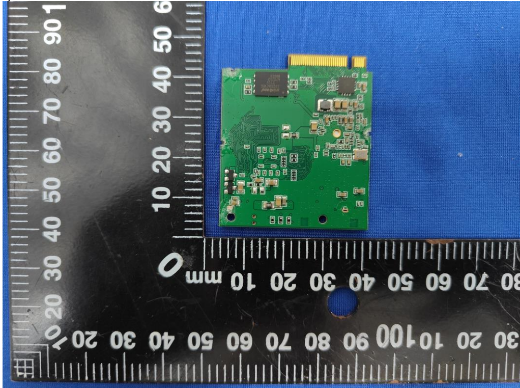
10) EUT Photo
