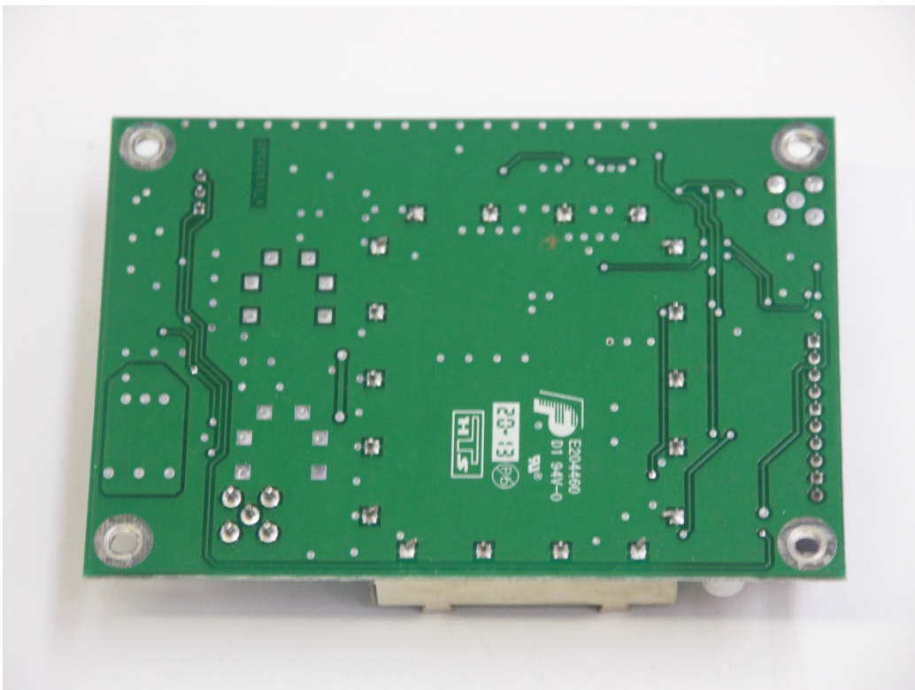
VCO BOTTOM
