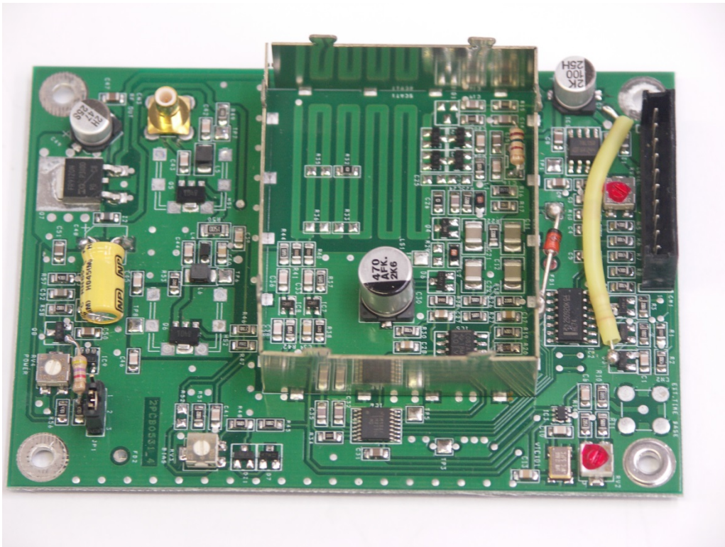
VCO BOTTOM
