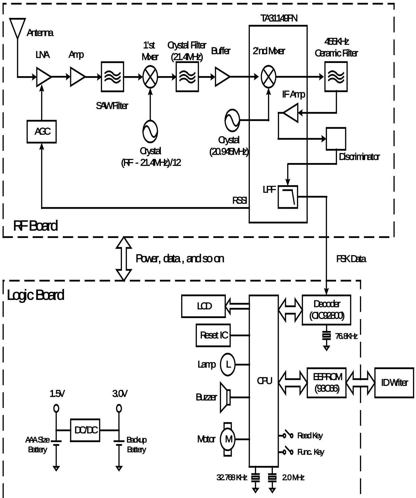
AN1000 Flex Block Diagram
