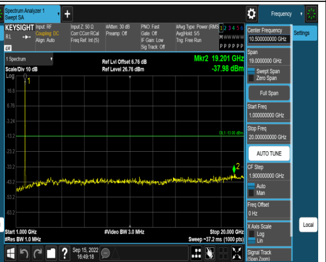
Band66-20MHz-16QAM-132072-1RB#0-Range2:1000 ~20000MHz
