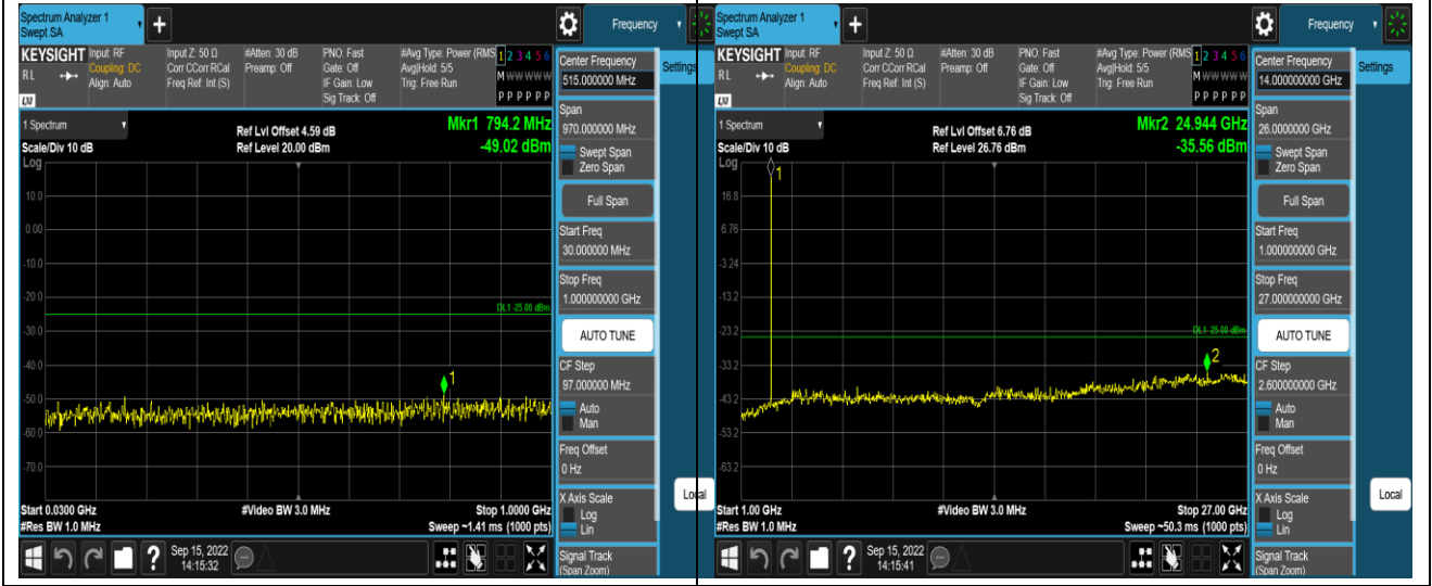
Band7-5MHz-QPSK-21425-1RB#0-Range1:30~10 00MHz Band7-5MHz-QPSK-21425-1RB#0-Range2:1000~270 00MHz
