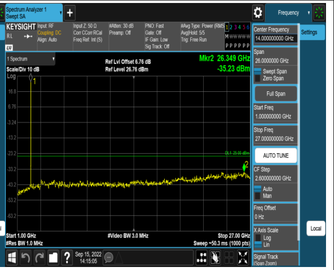
Band7-5MHz-QPSK-20775-1RB#0-Range2:1000~27000MHz
