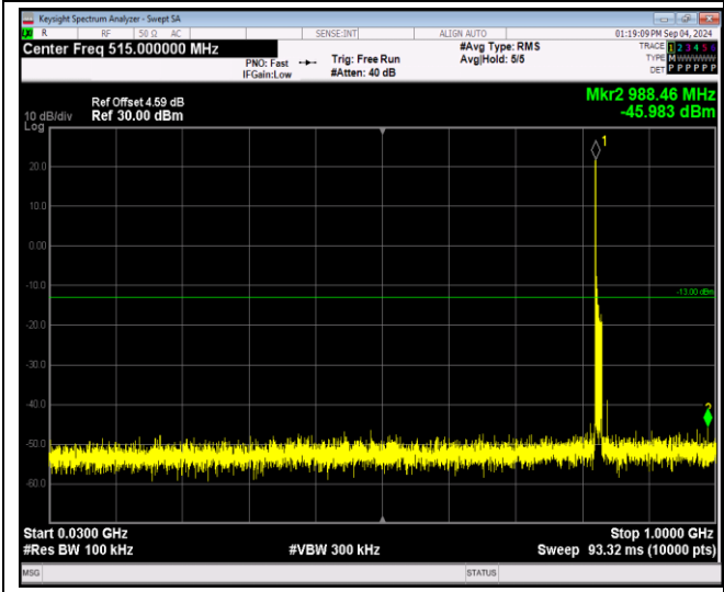
Band5-10MHz-QPSK-20525-1RB#0-Range1:1:30~100 OMHz
