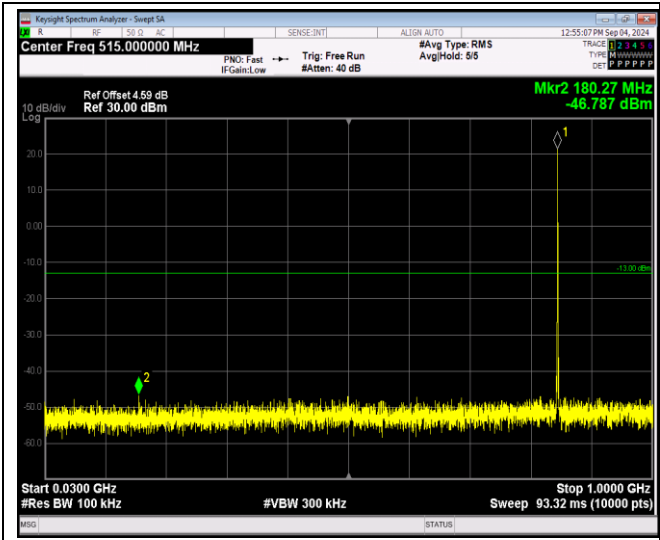
Band5-10MHz-QPSK-20450-1RB#0-Range1:1:30~100 OMHz
