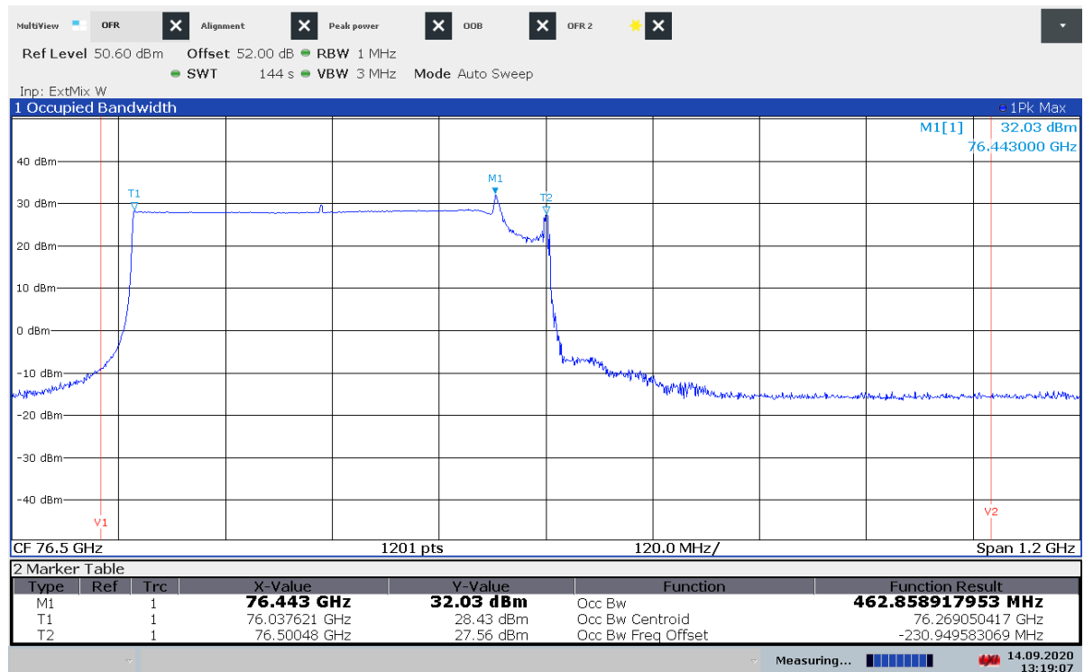
Plot 4: Mode 9(b), T_{\text{nom}} / V_{\text{nom}}
