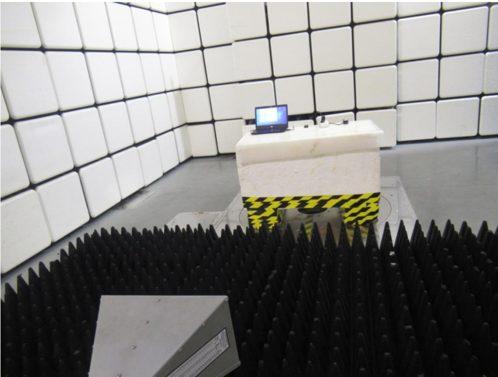
1GHz-18GHz
