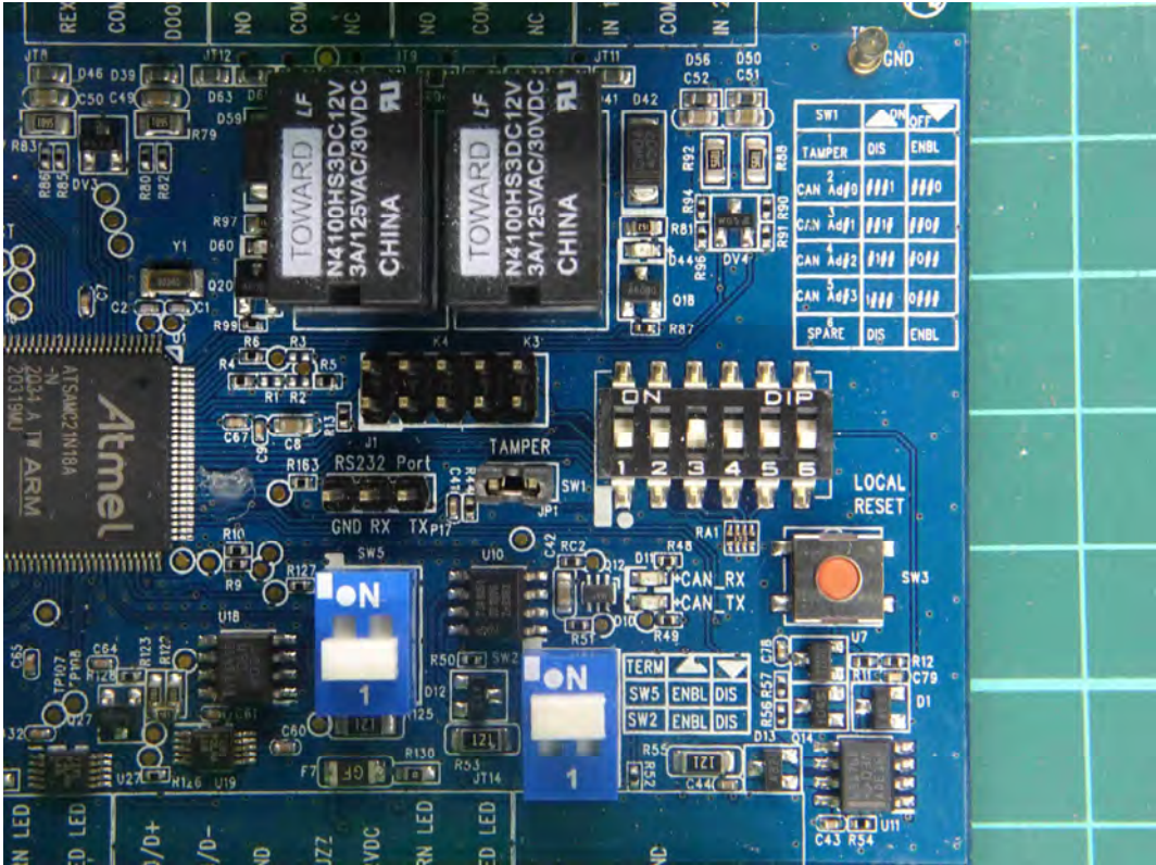
(207) EUT Photo
