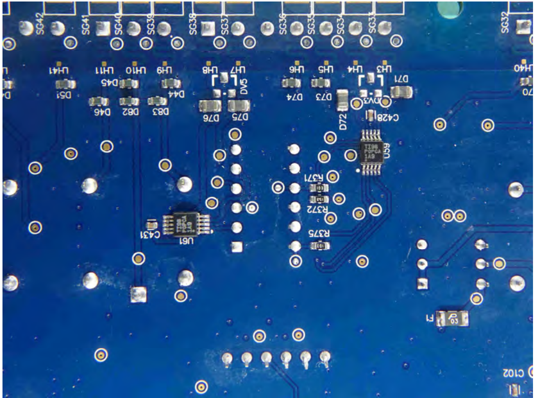
(248) EUT Photo
