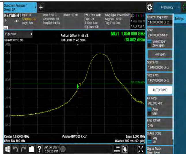
Band2-5MHz-QPSK-18625-1RB#24
