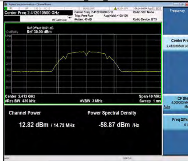
11B_Ant2_2412
