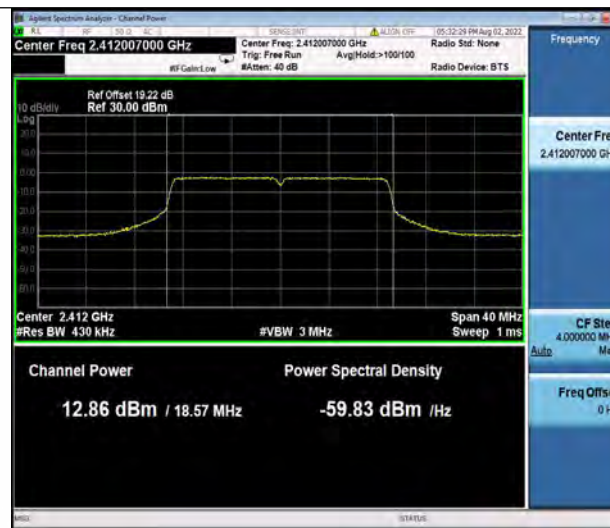
11N20MIMO_Ant2_2412
