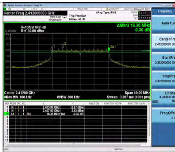
11G_Ant2_2412
