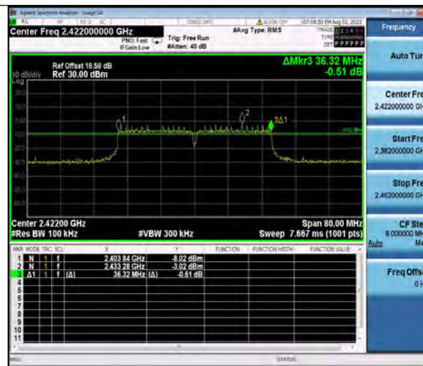
11N40MIMO_Ant2_2422
