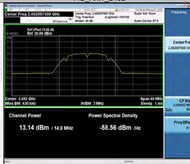
11B_Ant2_2462
