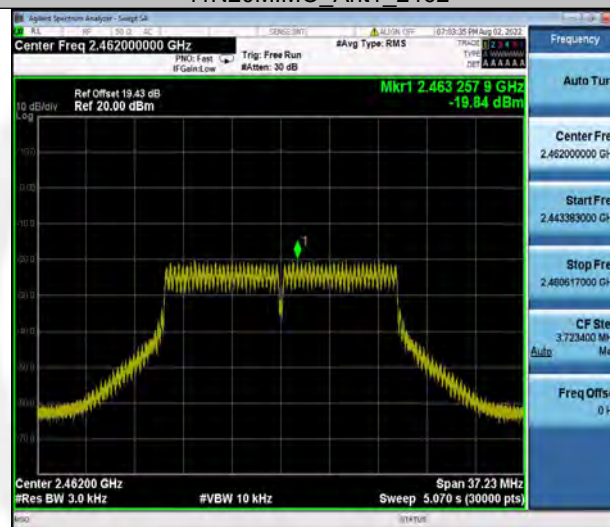
11N20MIMO_Ant2_2462
