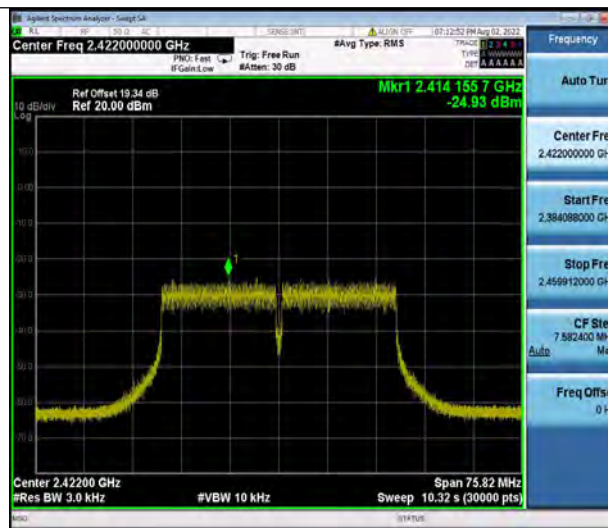
11N40MIMO_Ant2_2422
