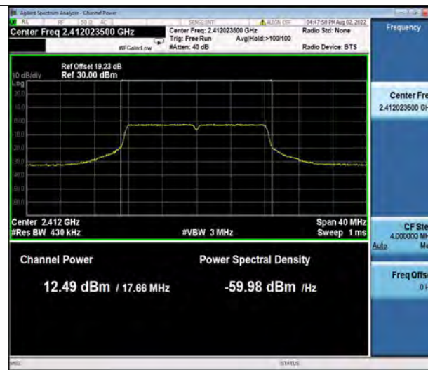
11G_Ant2_2412
