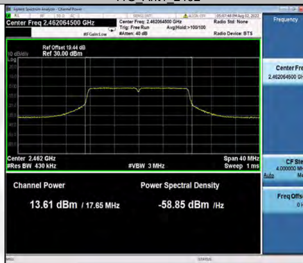
11G_Ant2_2462
