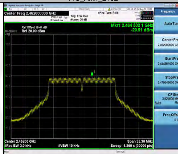
11G_Ant2_2462
