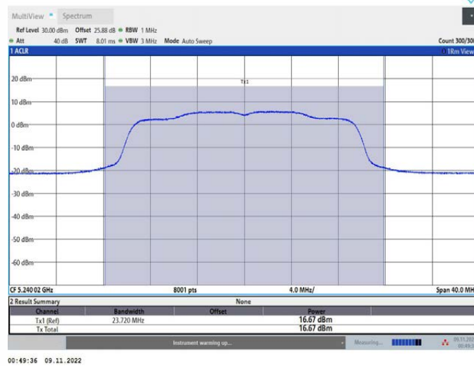
11AX20MIMO_Ant1_5240
