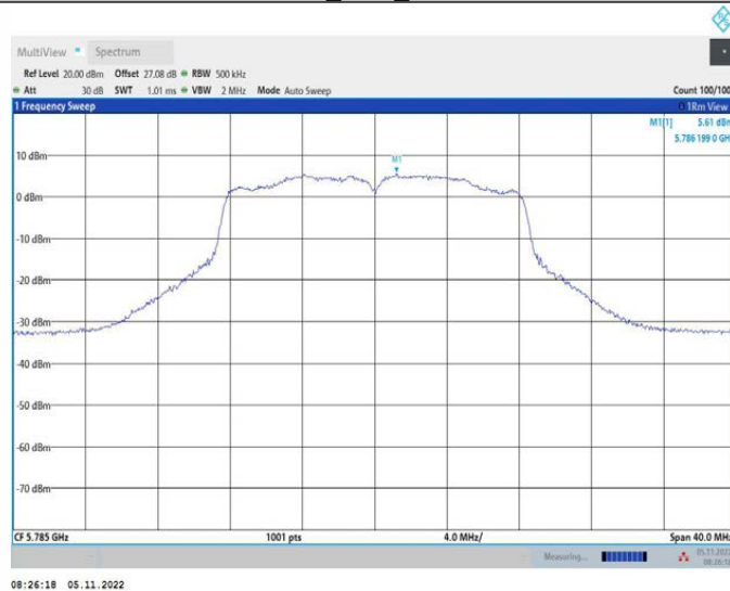
11A_Ant2_5785
