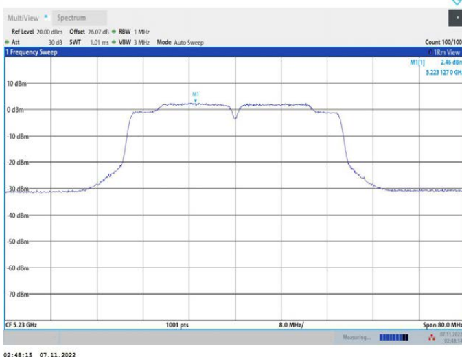
11N40MIMO_Ant2_5230
