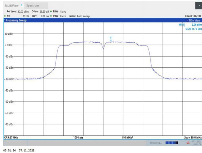
11N40MIMO_Ant2_5670
