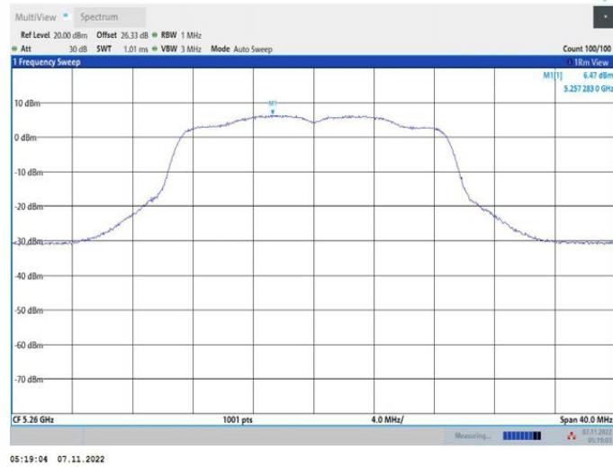
11AC20MIMO_Ant2_5260
