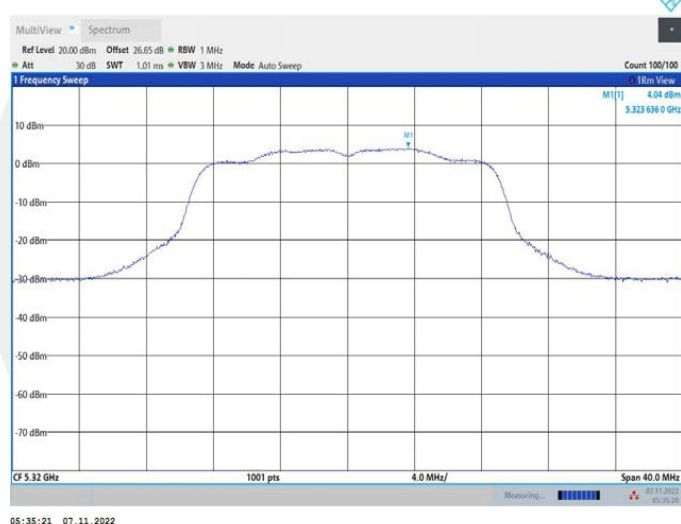
11AC20MIMO_Ant2_5320
