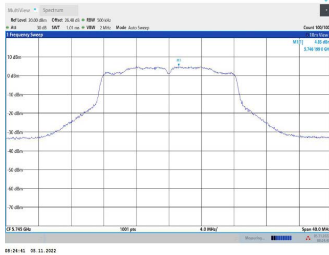
11A_Ant2_5745
