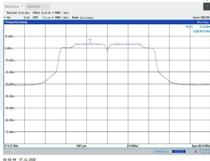
11N40MIMO_Ant2_5270
