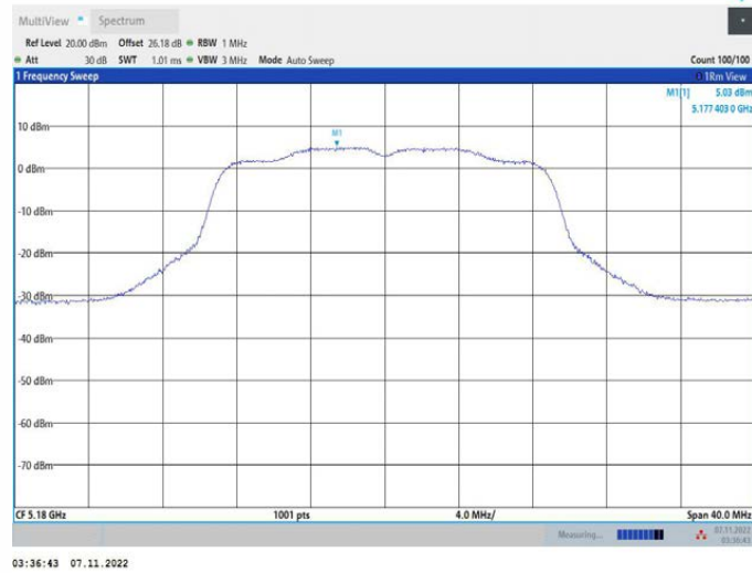
11AC20MIMO_Ant2_5180
