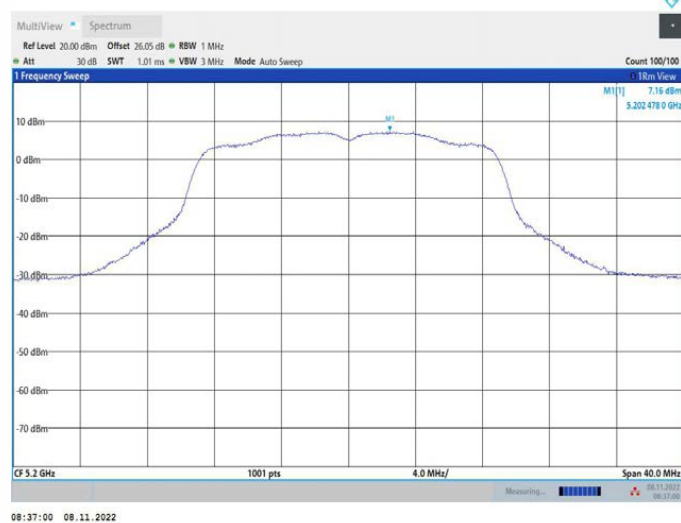
11AC20MIMO_Ant2_5200
