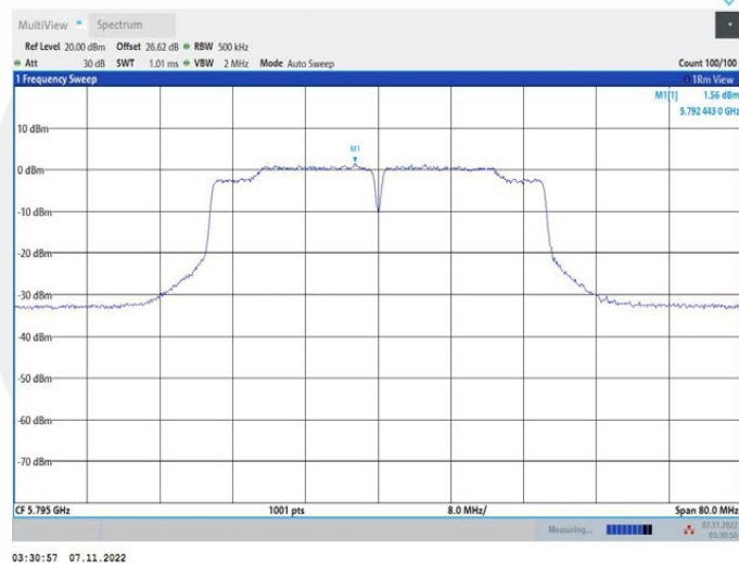
11N40MIMO_Ant2_5795
