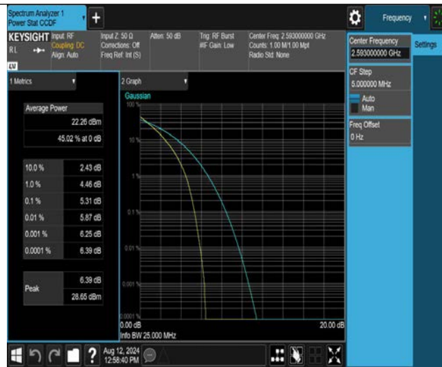
Band41-20MHz-QPSK-41490-1RB#0
